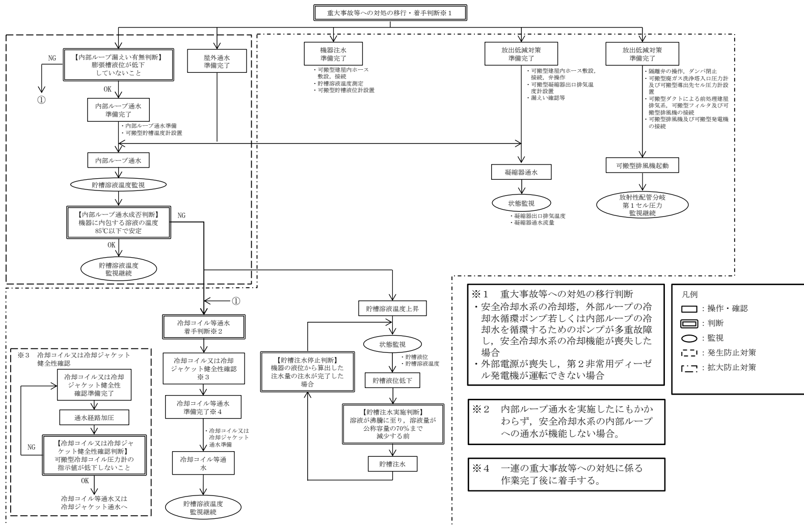
第62図 「地震発生による全交流動力電源の喪失を伴う前処理建屋の冷却機能喪失事故」の手順の概要
