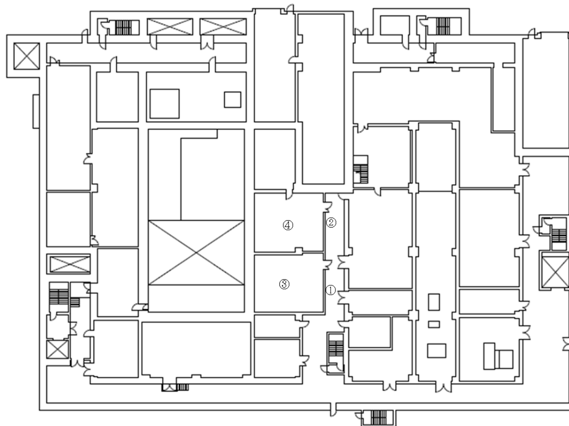
第 51 図 「高レベル廃液ガラス固化建屋の冷却機能喪失事故」の内部ループ通水接続口配置図（地上1階）
