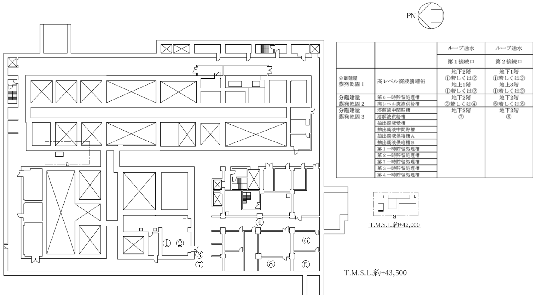
第13図 「分離建屋の冷却機能喪失事故」のループ通水接続口配置図（地下2階）
