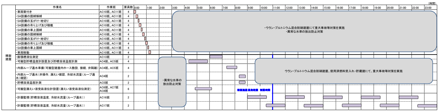
第74図 火山を想定した場合の精製建屋における内部ループへの通水に必要な要員及び作業項目
