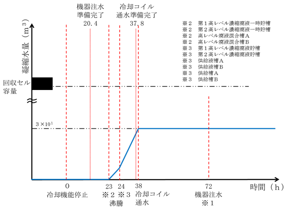
第 101 図 放出低減対策実施時の高レベル廃液ガラス固化建屋からの放出及び蒸気の凝縮傾向
