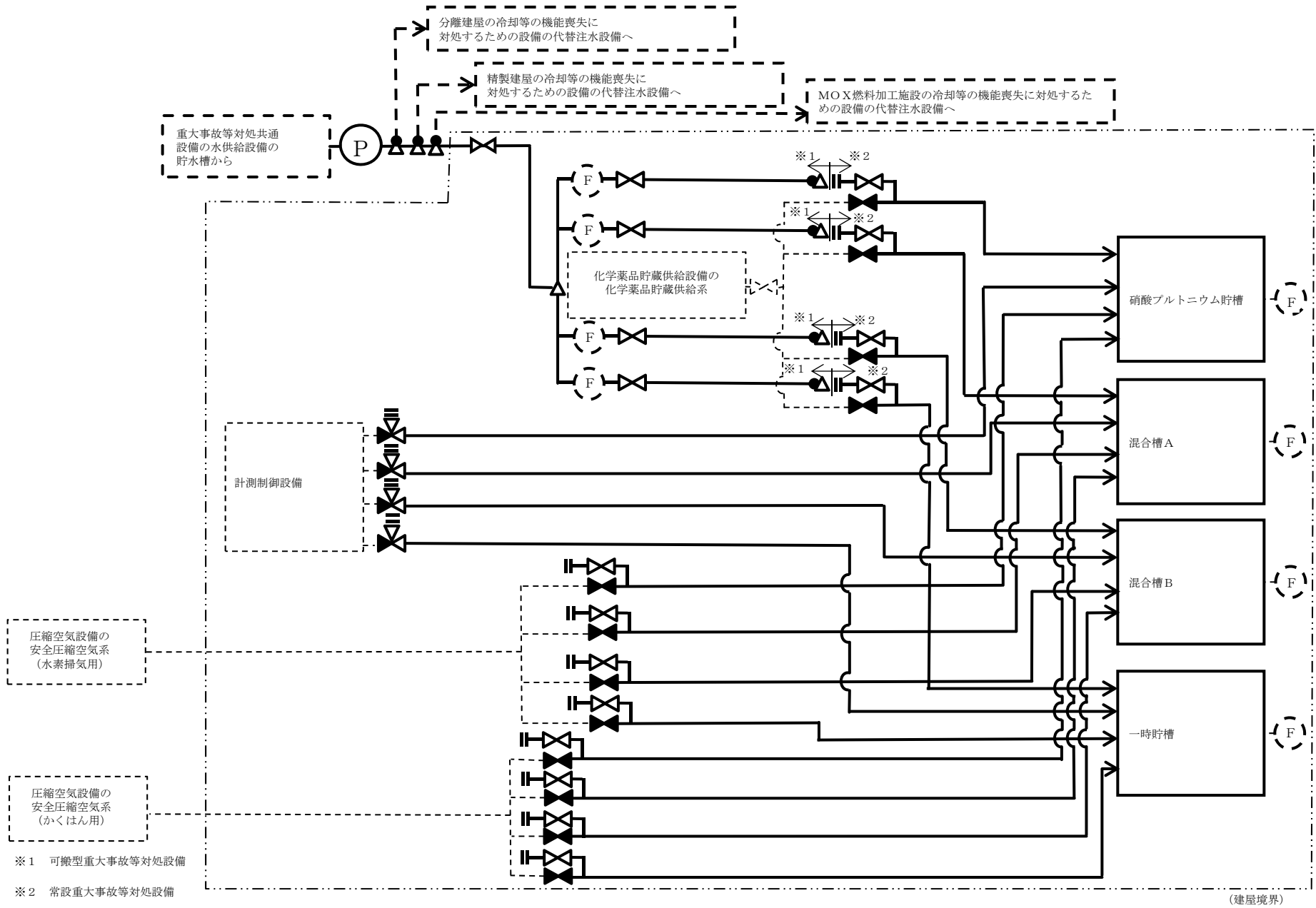
第42図 「ウラン・プルトニウム混合脱硝建屋の冷却機能喪失事故」の機器注水系統概要図
