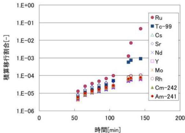
第2. - 3図 凝縮液のICP-MS分析結果 (~400℃/100W)
