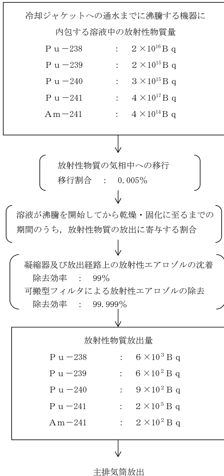
第 104 図 「地震発生による全交流動力電源の喪失を伴うウラン・プルトニウム混合脱硝建屋の冷却機能喪失事故」時の放射性物質の大気放出過程
