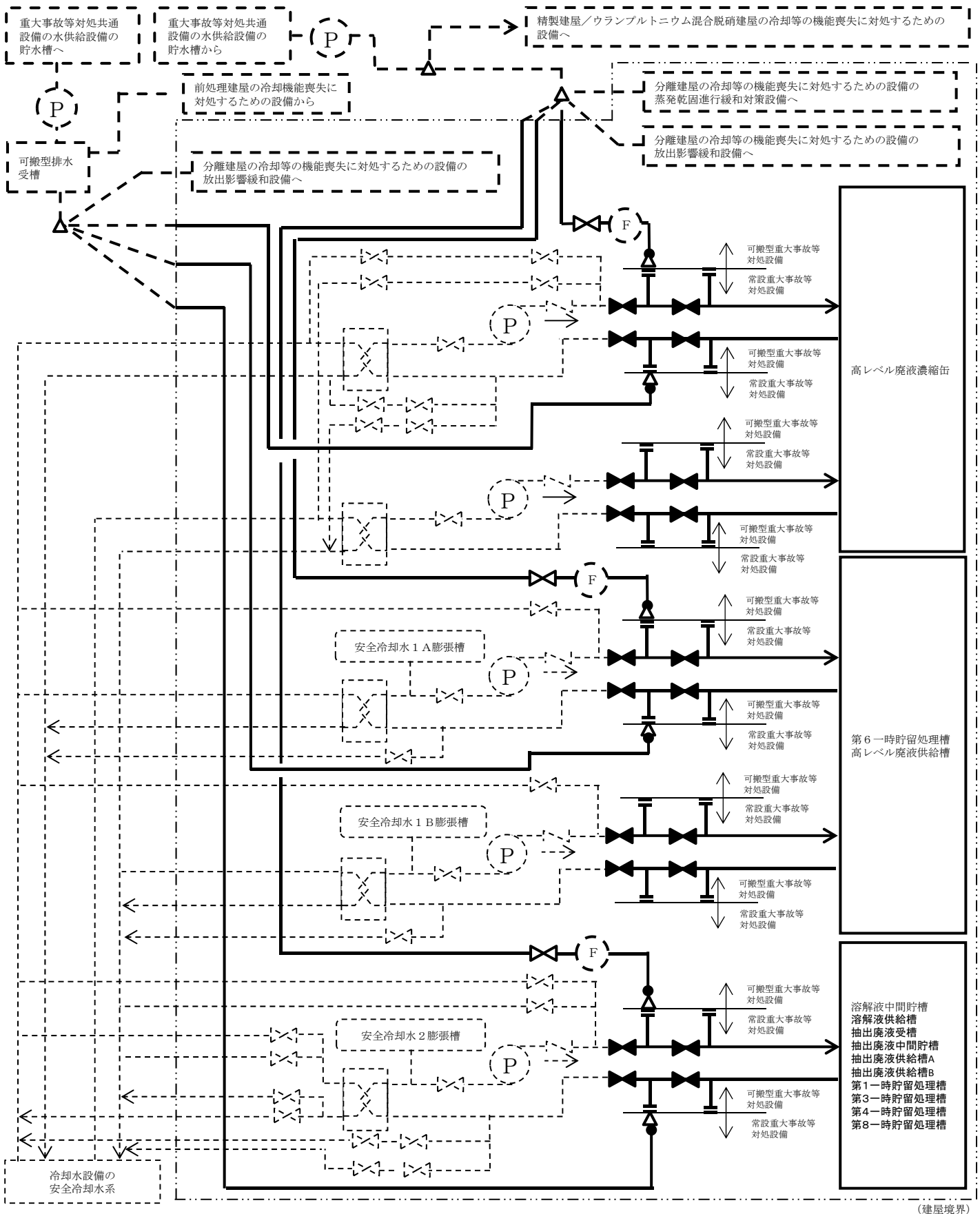
本図は、分離建屋蒸発乾固1の2系統のうち1系統、離建屋蒸発乾固2の2系統のうち1系統及び分離建屋蒸発乾固3の第1接続口の接続例である。分離建屋蒸発乾固1の他の1系統、分離建屋蒸発乾固2の他の1系統及び分離建屋蒸発乾固3並びに第2接続口に接続した場合も同様の系統である。ただし、接続金具等の位置は、ホース敷設ルート毎に異なる。
