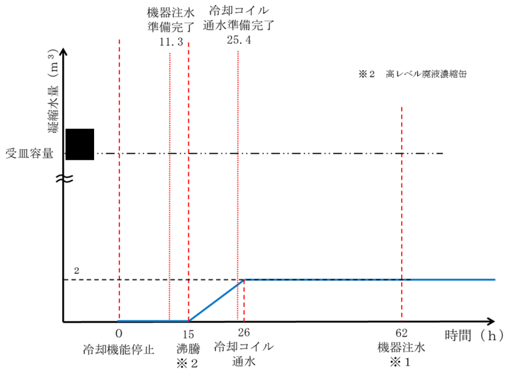
第 89 図 放出低減対策実施時の分離建屋からの放出及び蒸気の凝縮傾向
