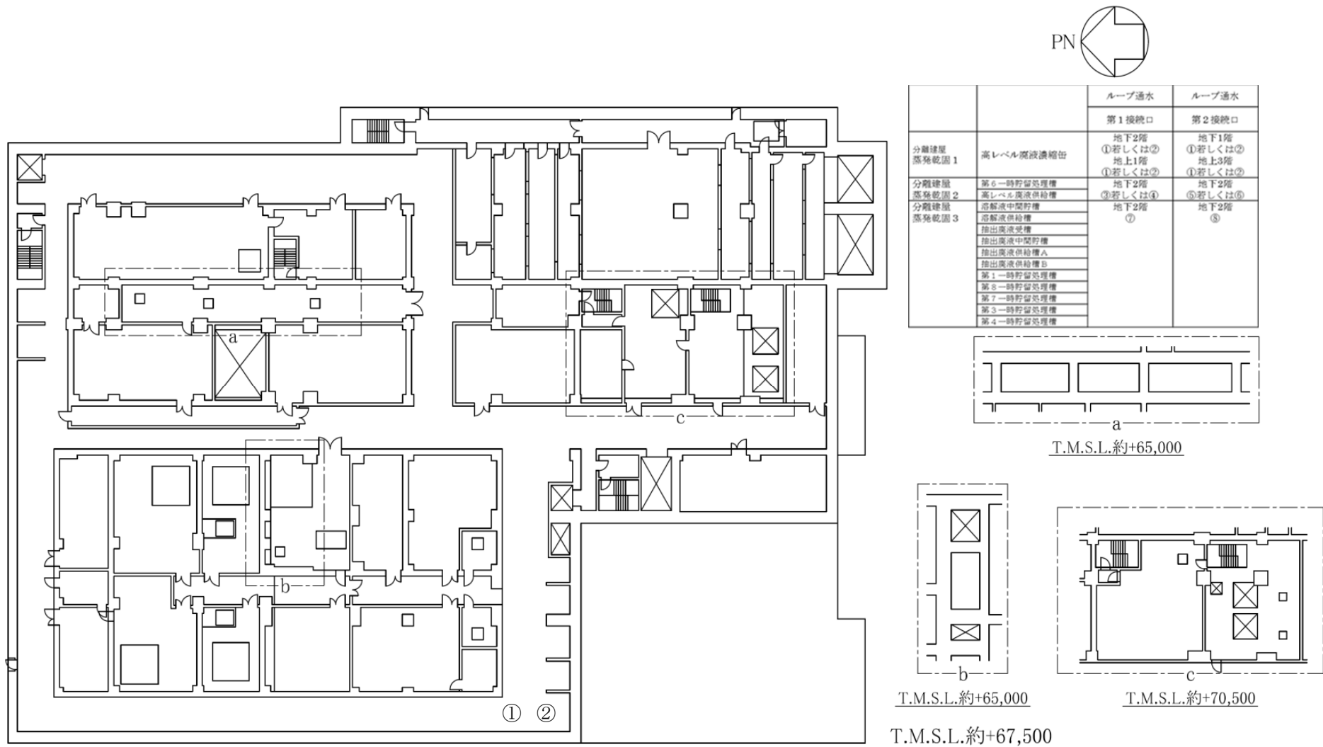
第16図 「分離建屋の冷却機能喪失事故」のループ通水接続口配置図（地上3階）
