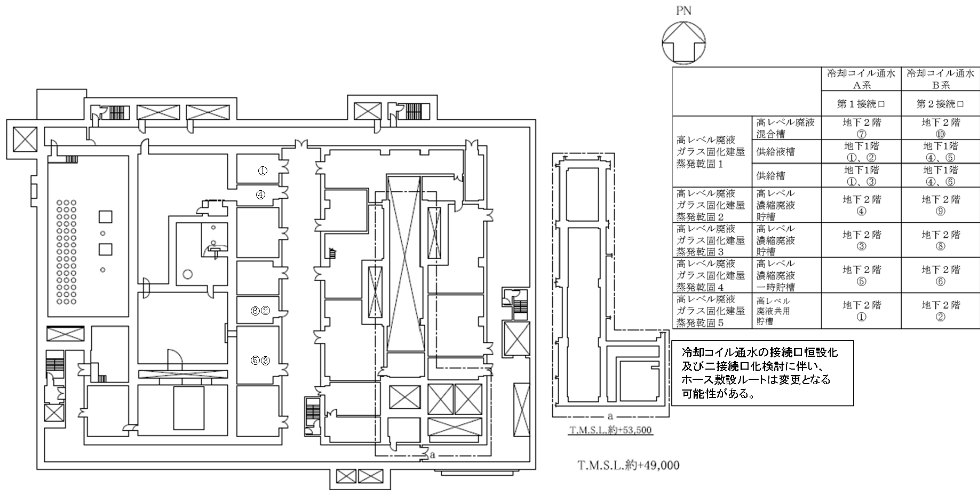
第 59 図 「高レベル廃液ガラス固化建屋の冷却機能喪失事故」の冷却コイル通水接続口配置図（地下 1
