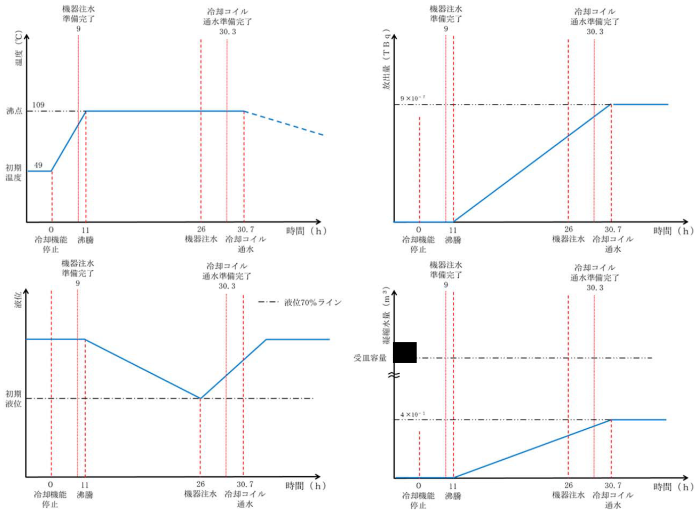
第92図 放出低減対策実施時のプルトニウム濃縮液一時貯槽に内包する溶液の温度、液位、放出及び蒸気の凝縮傾向
