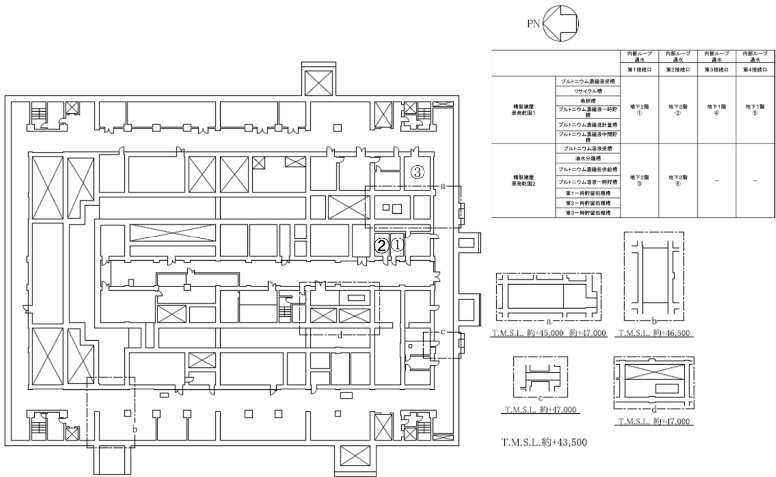
第 29 図 「精製建屋の冷却機能喪失事故」の機器注水接続口配置図（地下 2 階）
