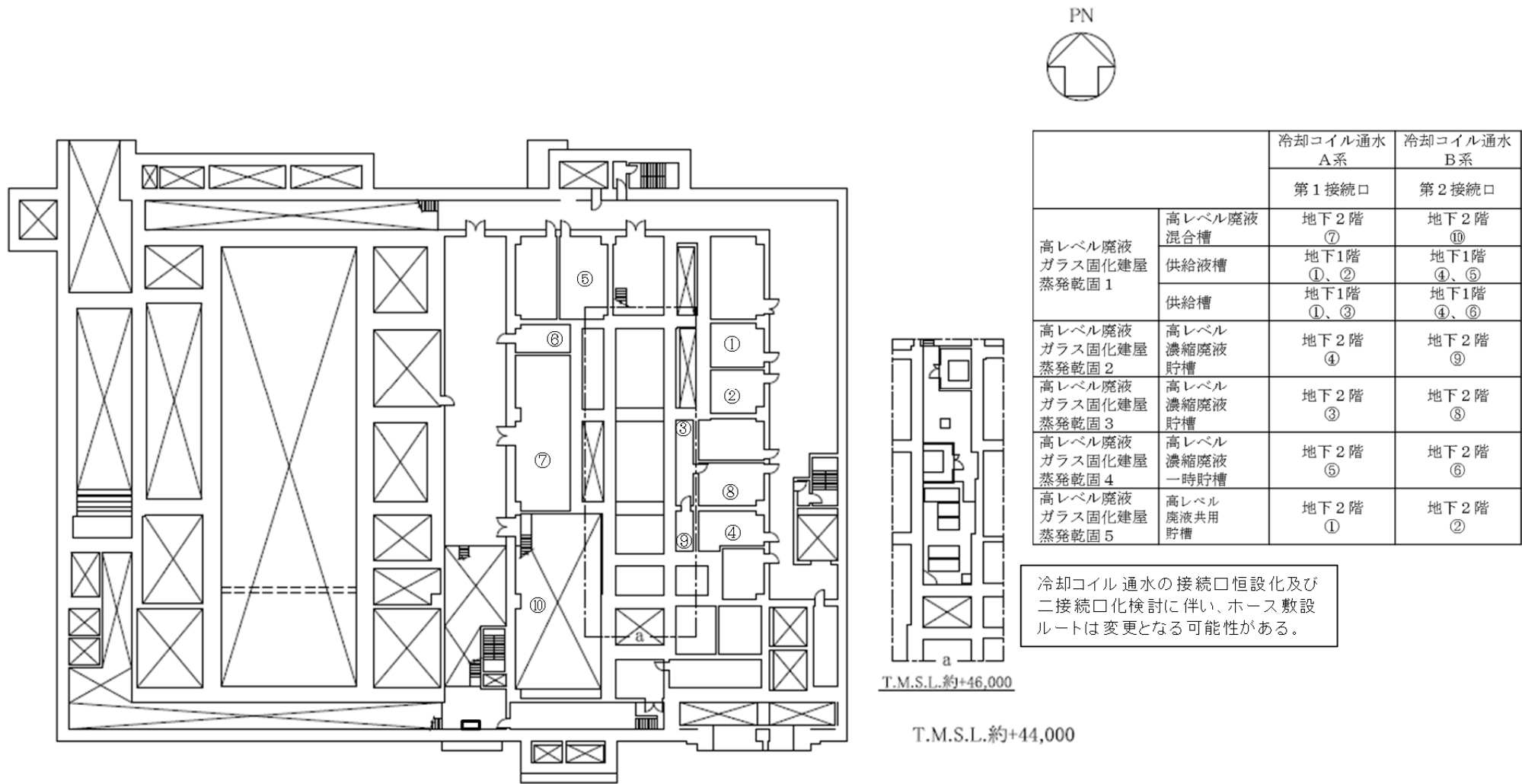
第 58 図 「高レベル廃液ガラス固化建屋の冷却機能喪失事故」の冷却コイル通水接続口配置図（地下2階）
