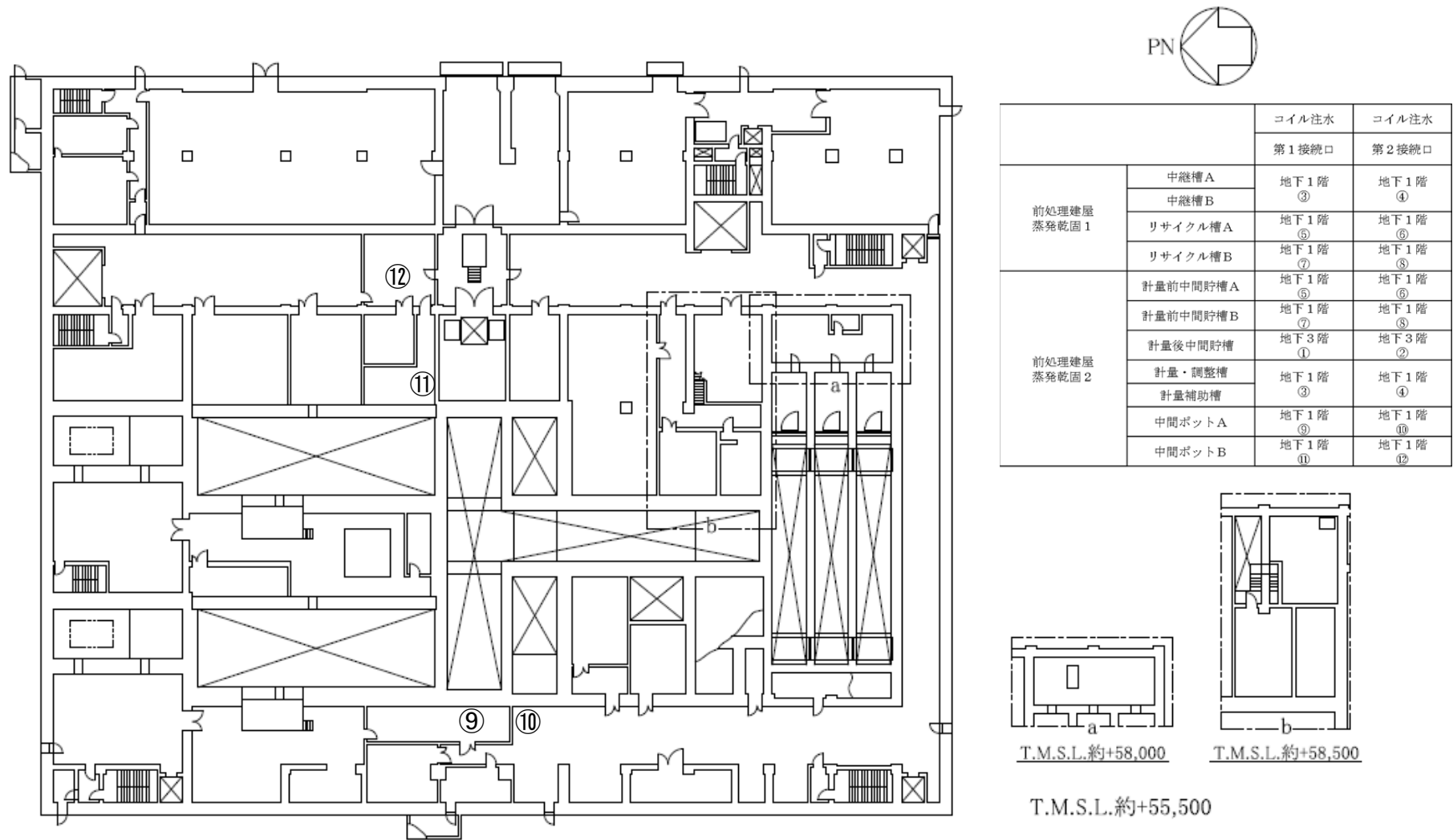
第9図 「前処理建屋の冷却機能喪失事故」の冷却コイル注水接続口配置図（地上1階）
