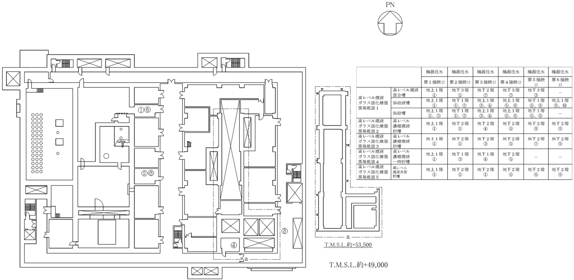
第55図 「高レベル廃液ガラス固化建屋の冷却機能喪失事故」の機器注水接続口配置図（地下1階）
