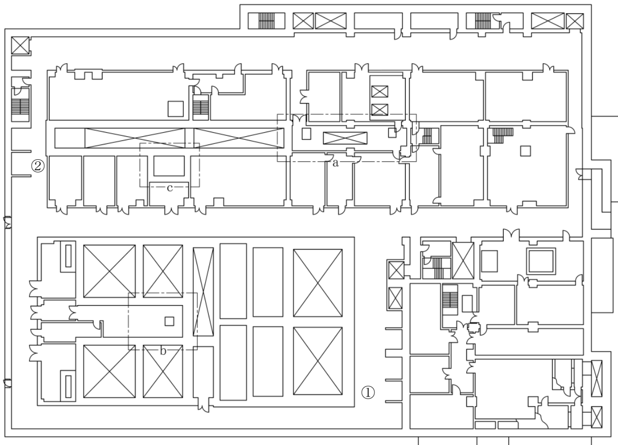
第23図 「分離建屋の冷却機能喪失事故」のコイル通水接続口配置図（地上2階）
