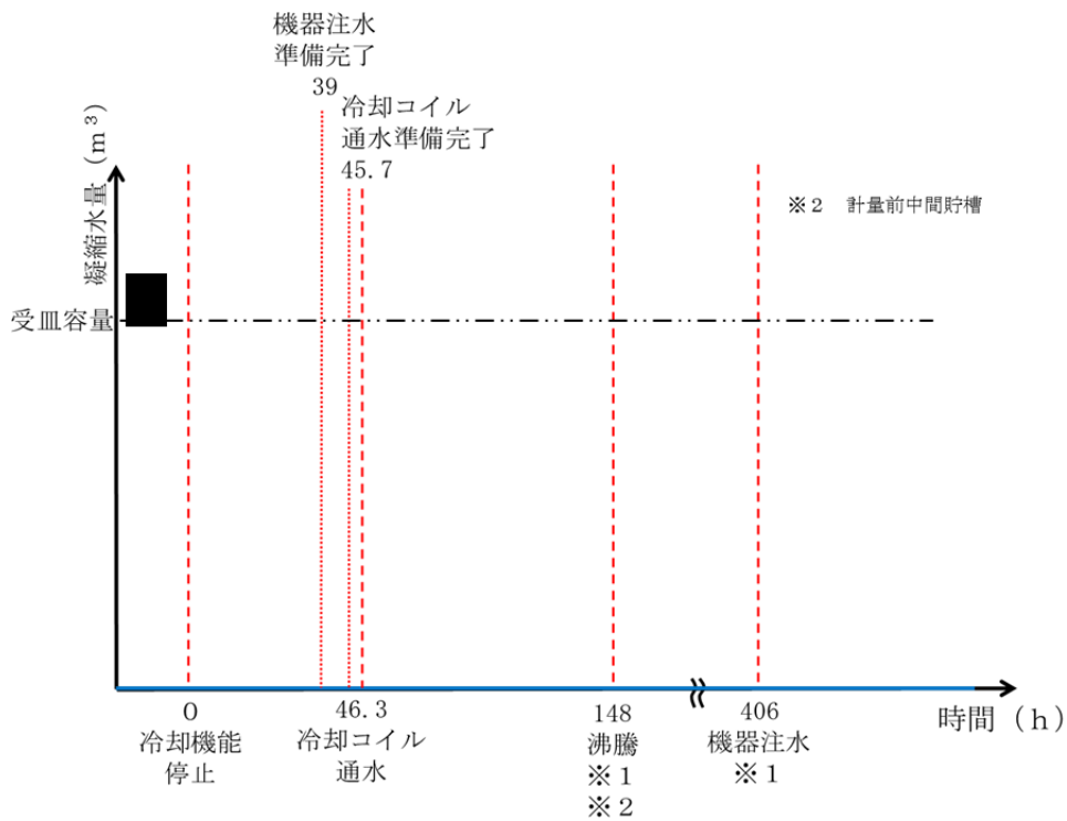
第 85 図 放出低減対策実施時の前処理建屋からの放出及び蒸気の凝縮傾向
