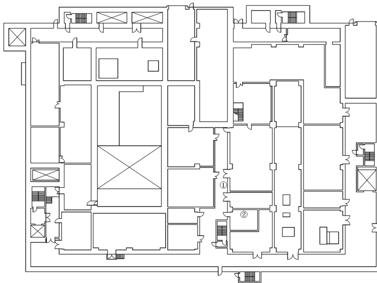
第 61 図 「高レベル廃液ガラス固化建屋の冷却機能喪失事故」の凝縮器通水接続口配置図（地上1階）
