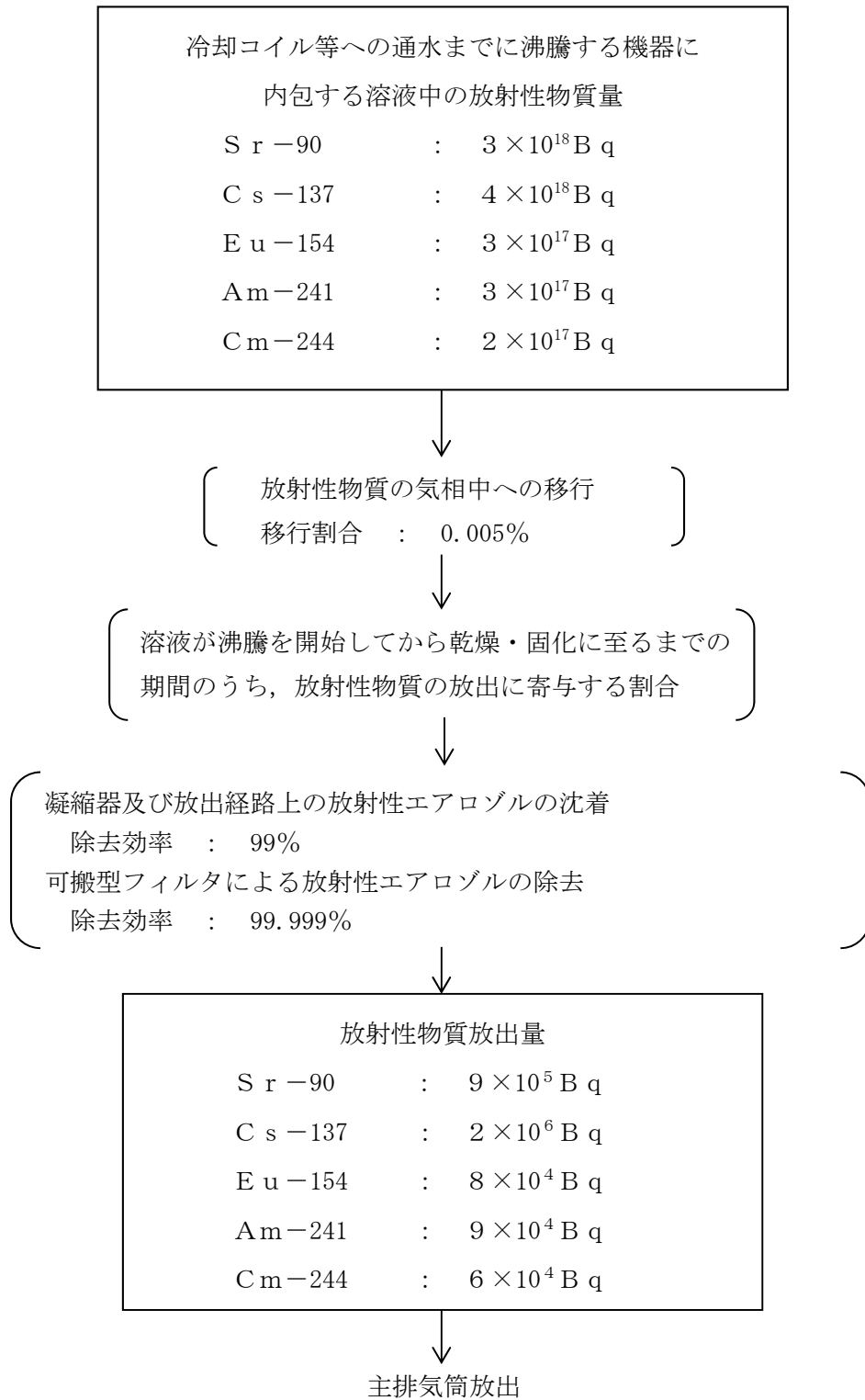
第 105 図 「地震発生による全交流動力電源の喪失を伴う高レベル廃液ガラス固化建屋の冷却機能喪失事故」時の放射性物質の大気放出過程
