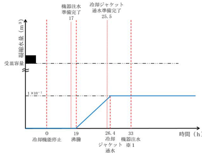
第 96 図 放出低減対策実施時の硝酸プルトニウム貯槽に 内包する溶液の温度，液位，放出及び蒸気の凝縮傾向
