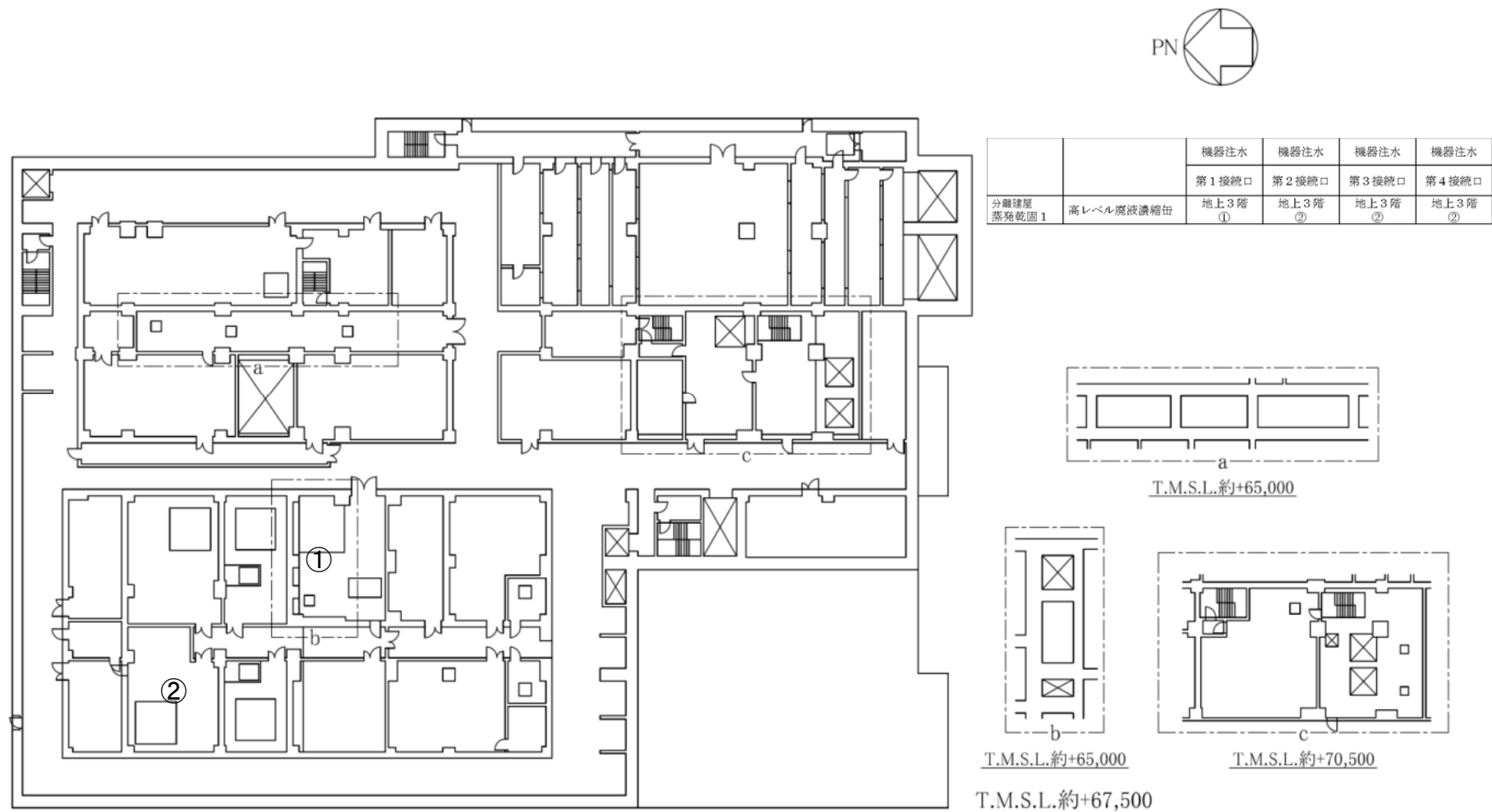
第 18 図 「分離建屋の冷却機能喪失事故」の機器注水接続口配置図（地上 3 階）
