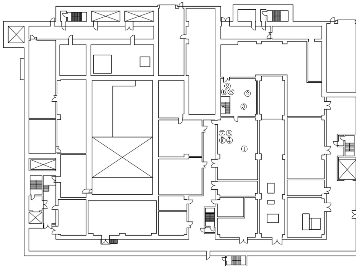
第56図 「高レベル廃液ガラス固化建屋の冷却機能喪失事故」の機器注水接続口配置図（地上1階）
