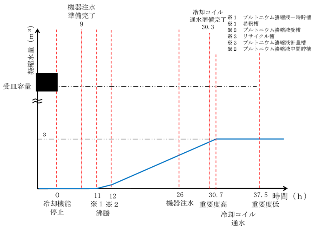
第 93 図 放出低減対策実施時の精製建屋からの放出及び蒸気の凝縮傾向
