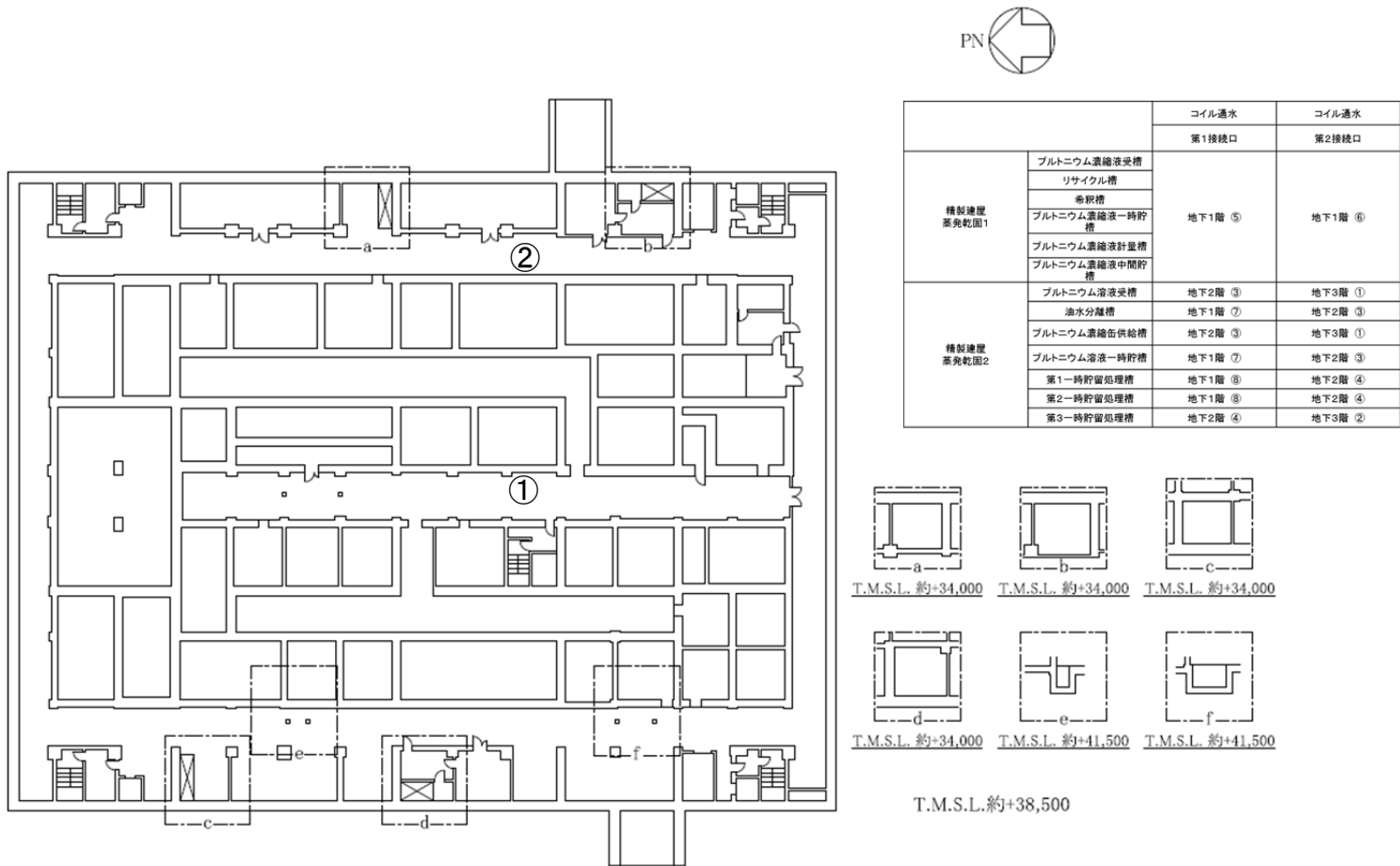
第 35 図 「精製建屋の冷却機能喪失事故」の冷却コイル通水接続口配置図（地下 3 階）
