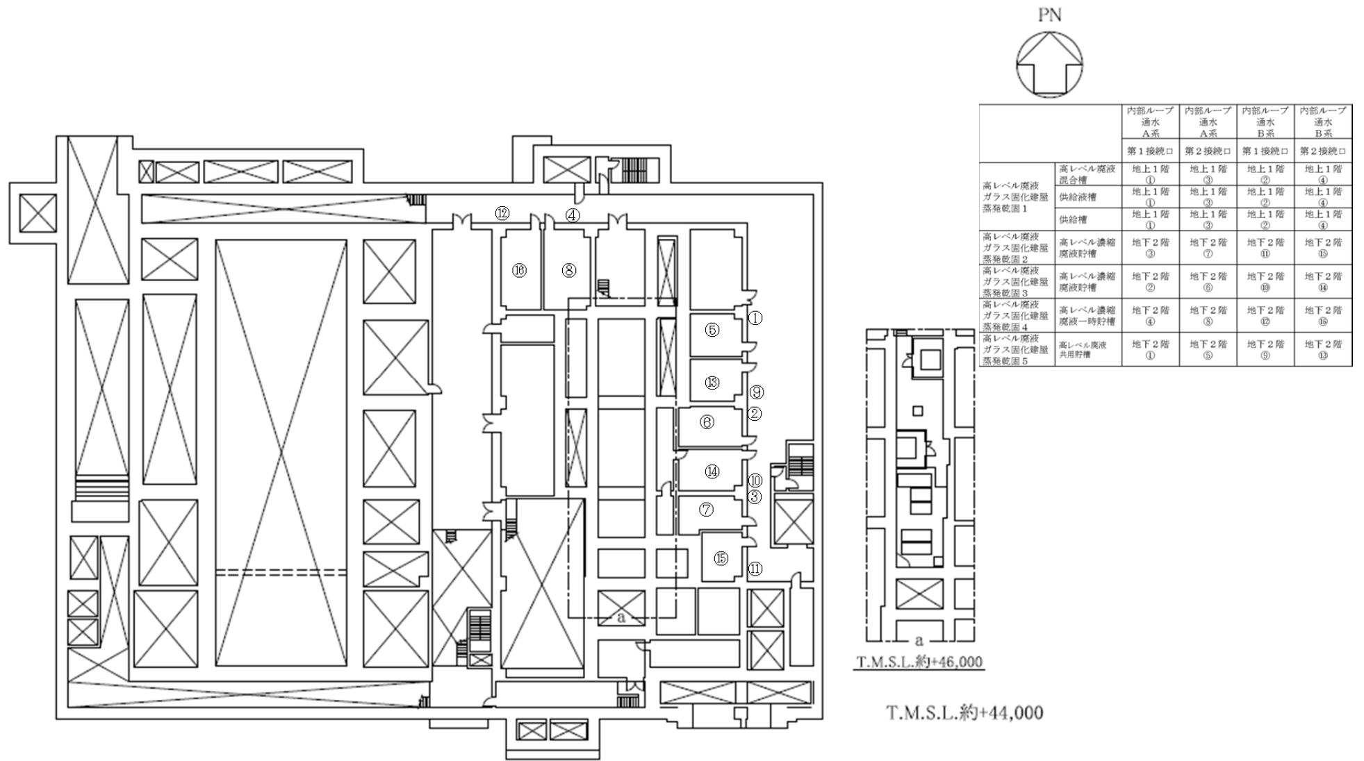
第50図 「高レベル廃液ガラス固化建屋の冷却機能喪失事故」の内部ループ通水接続口配置図（地下2階）
