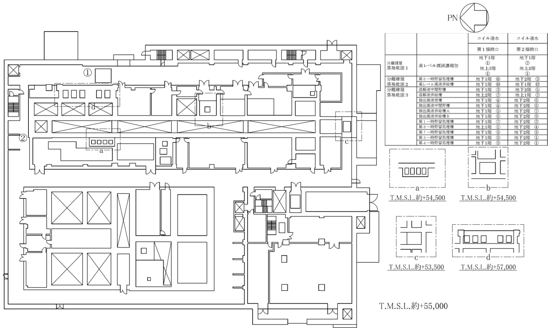
第 22 図 「分離建屋の冷却機能喪失事故」のコイル通水接続口配置図（地上 1 階）
