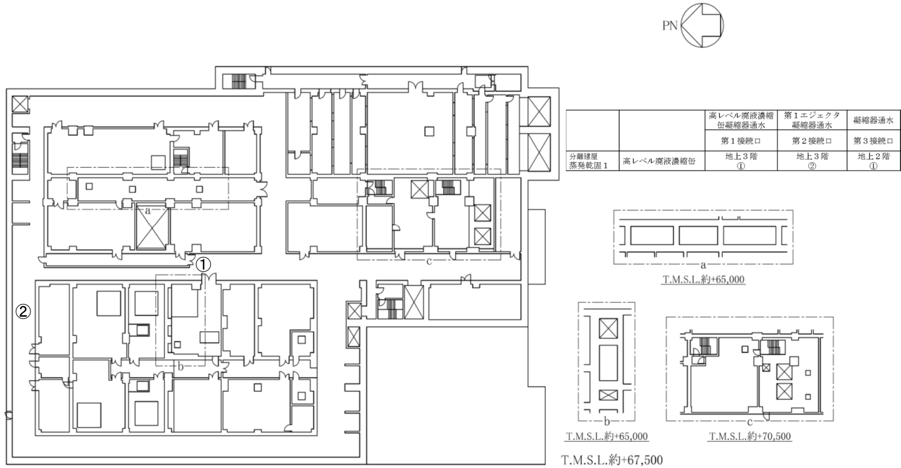
第 27 図 「分離建屋の冷却機能喪失事故」の凝縮器通水接続口配置図（地上 3 階）
