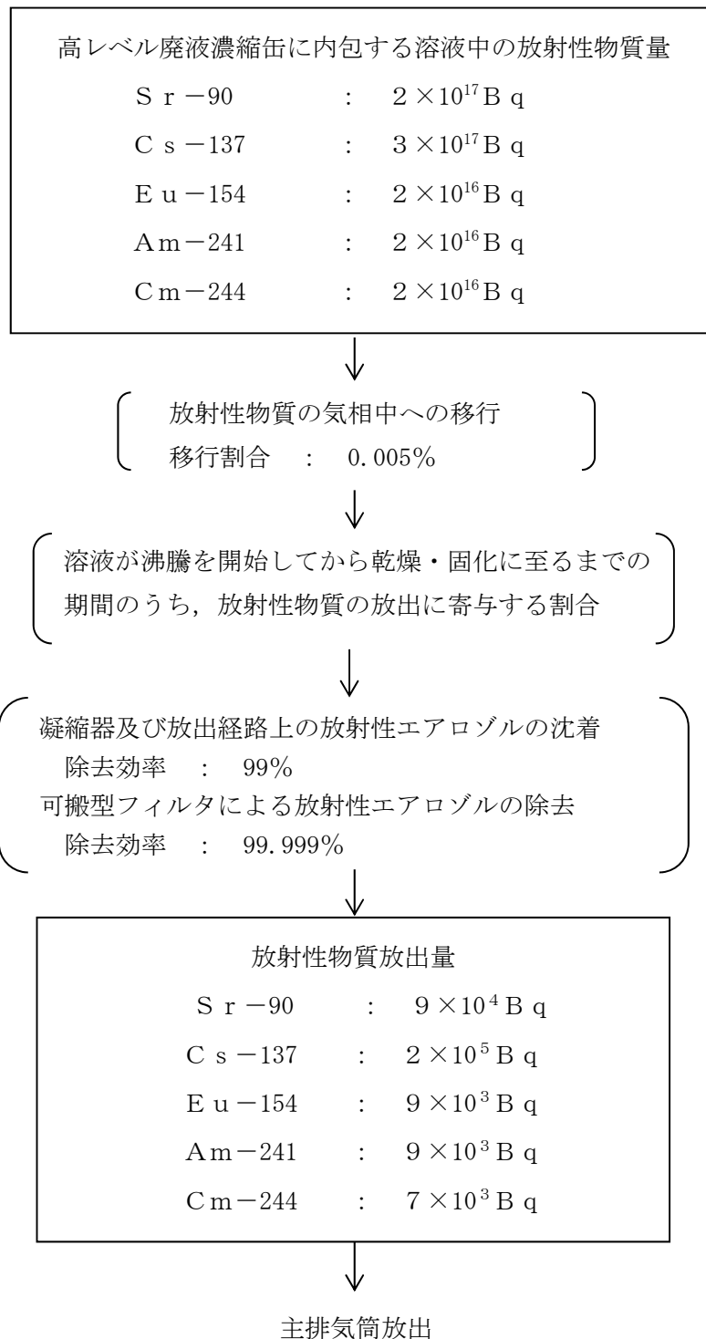
第 102 図 「地震発生による全交流動力電源の喪失を伴う分離建屋の冷却機能喪失事故」時の放射性物質の大気放出過程
