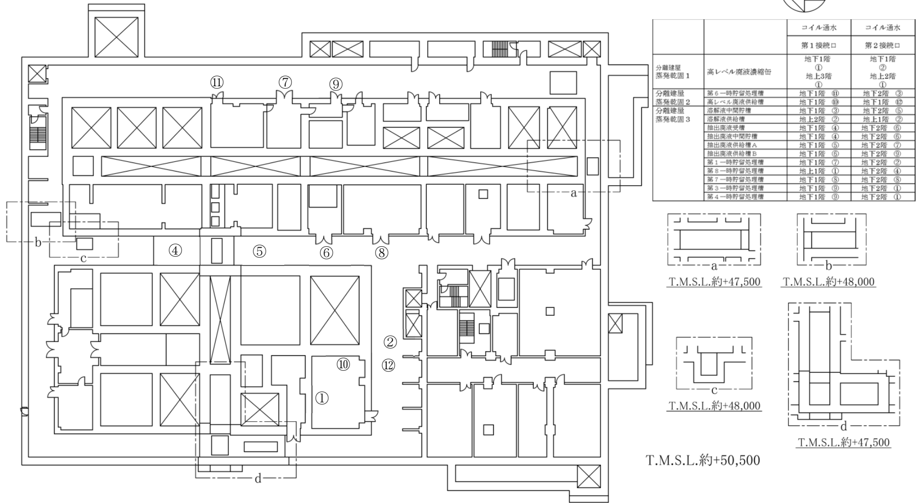
第 21 図 「分離建屋の冷却機能喪失事故」のコイル通水接続口配置図（地下 1 階）
