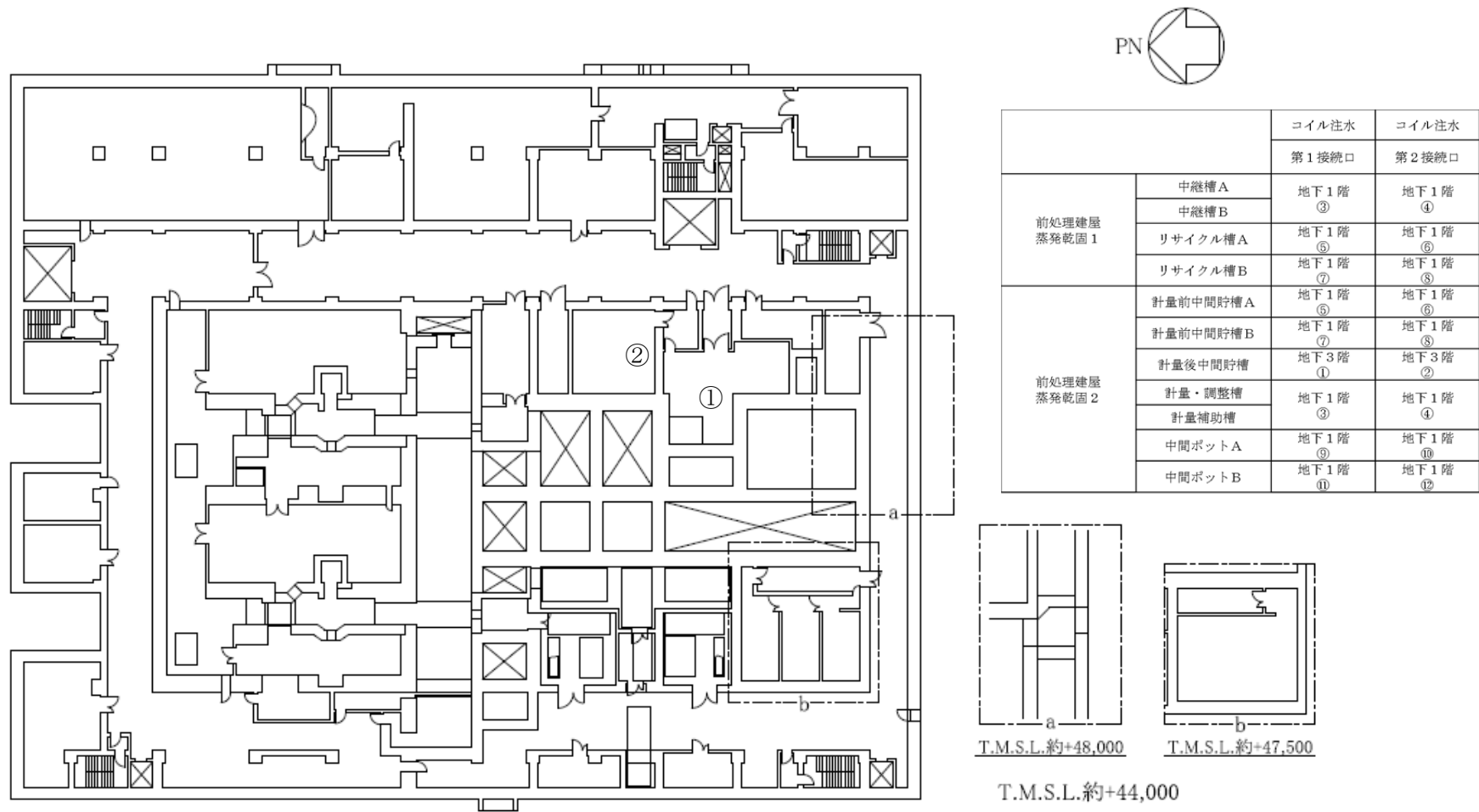
第7図 「前処理建屋の冷却機能喪失事故」の冷却コイル注水接続口配置図（地下3階）
