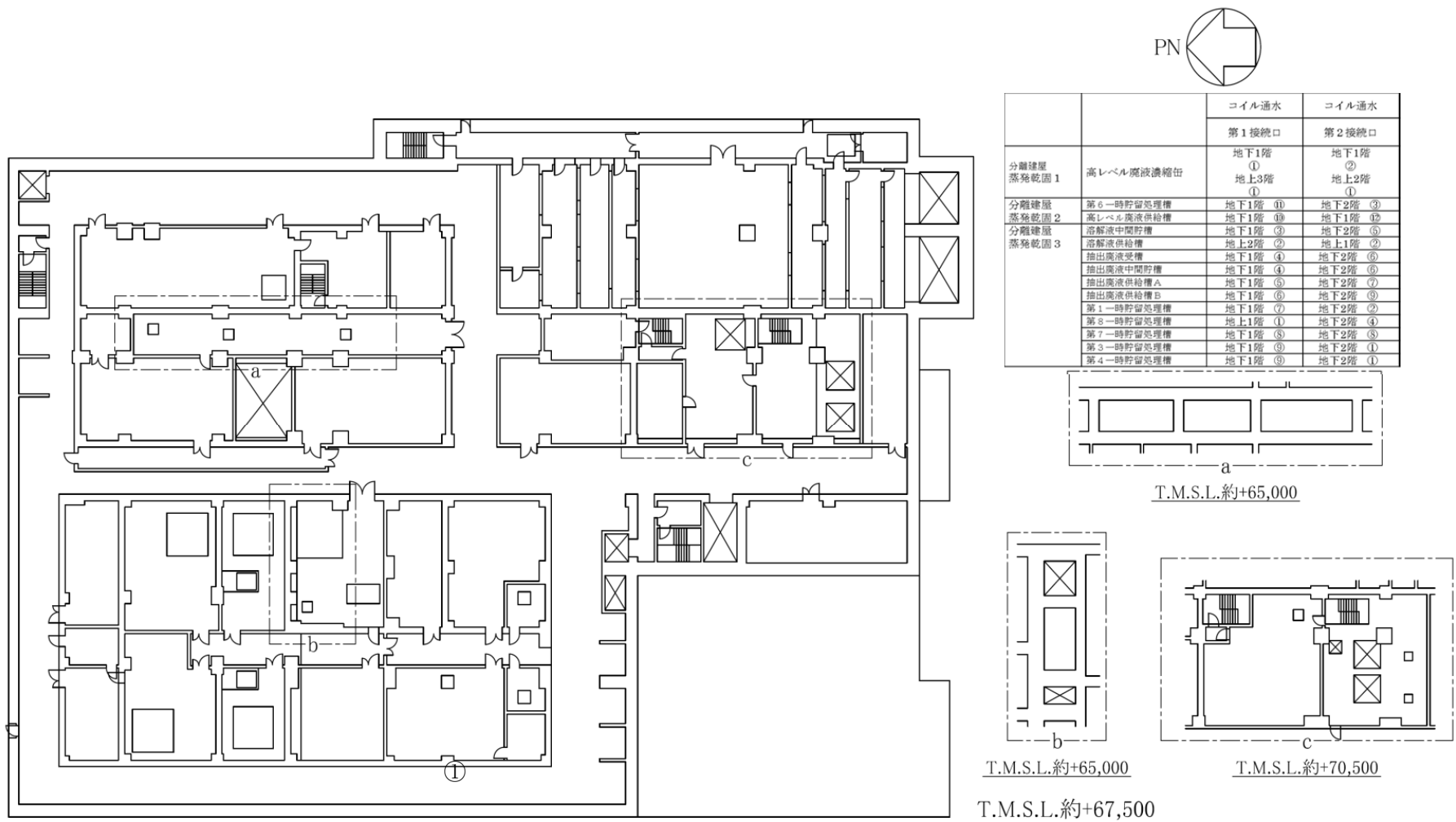
第 24 図 「分離建屋の冷却機能喪失事故」のコイル通水接続口配置図（地上 3 階）
