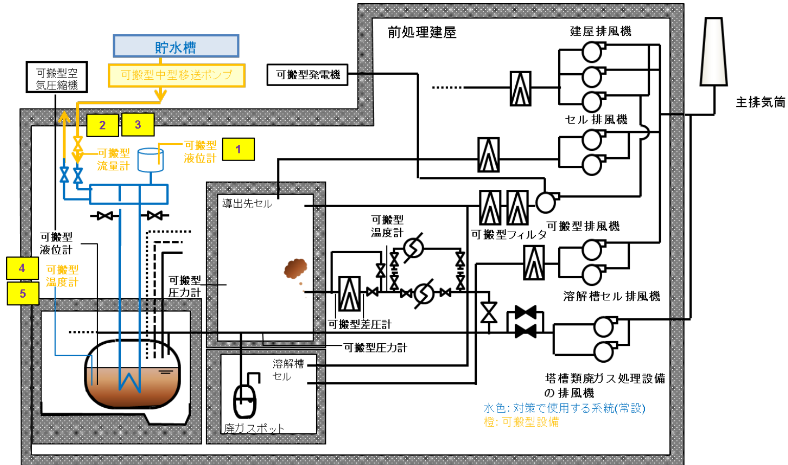
第 1. - 1 図 前処理建屋の内部ループ通水による冷却概要図
