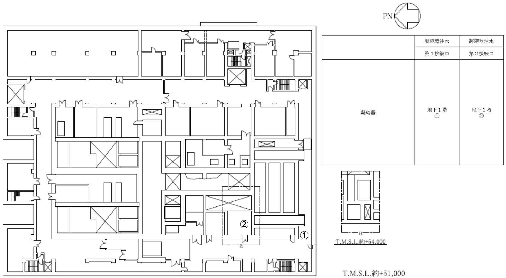
第11図 「前処理建屋の冷却機能喪失事故」の凝縮器注水接続口配置図（地下1階）
