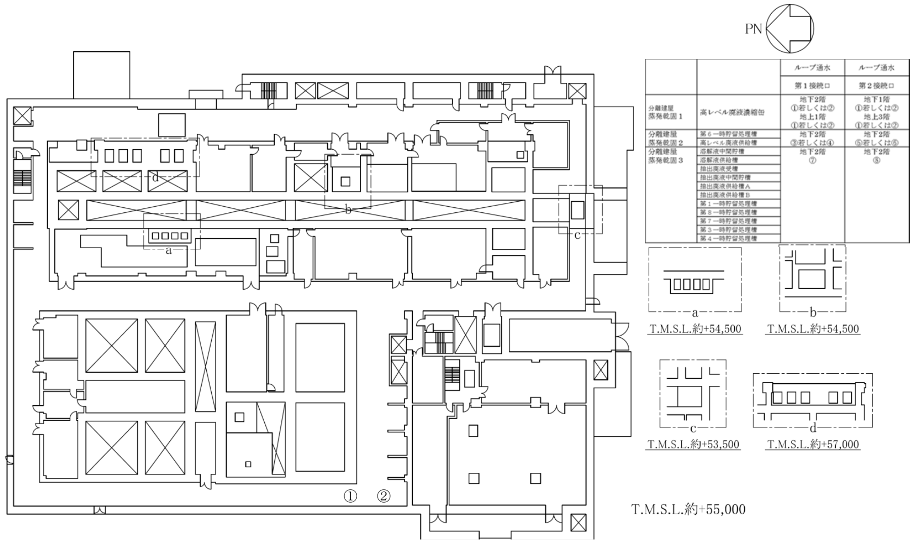
第15図 「分離建屋の冷却機能喪失事故」のループ通水接続口配置図（地上1階）
