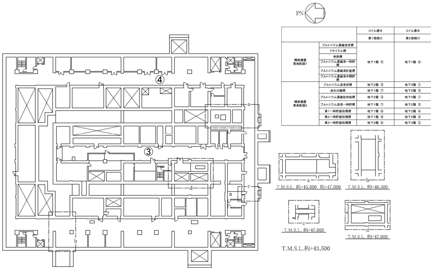
第 36 図 「精製建屋の冷却機能喪失事故」の冷却コイル通水接続口配置図（地下 2 階）
