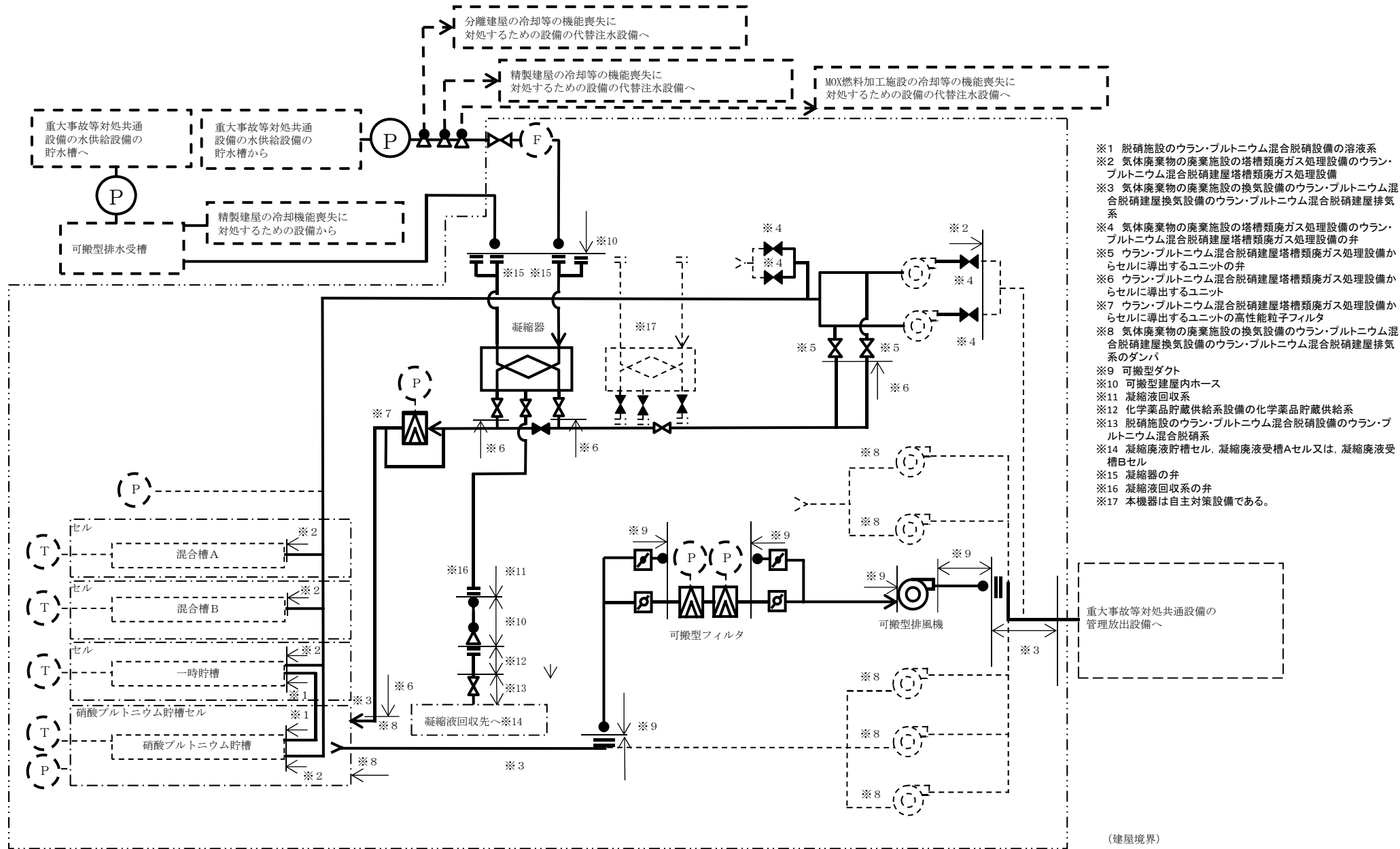
第47図 「ウラン・プルトニウム混合脱硝建屋の冷却機能喪失事故」の換気系統遮断・セル内導出及び放出影響緩和系統概要図
