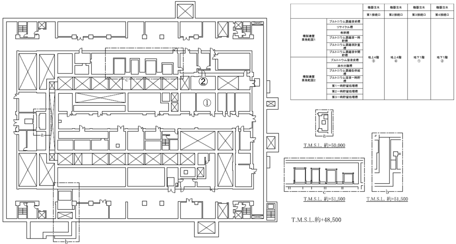
第 32 図 「精製建屋の冷却機能喪失事故」の機器注水接続口配置図（地上 1 階）
