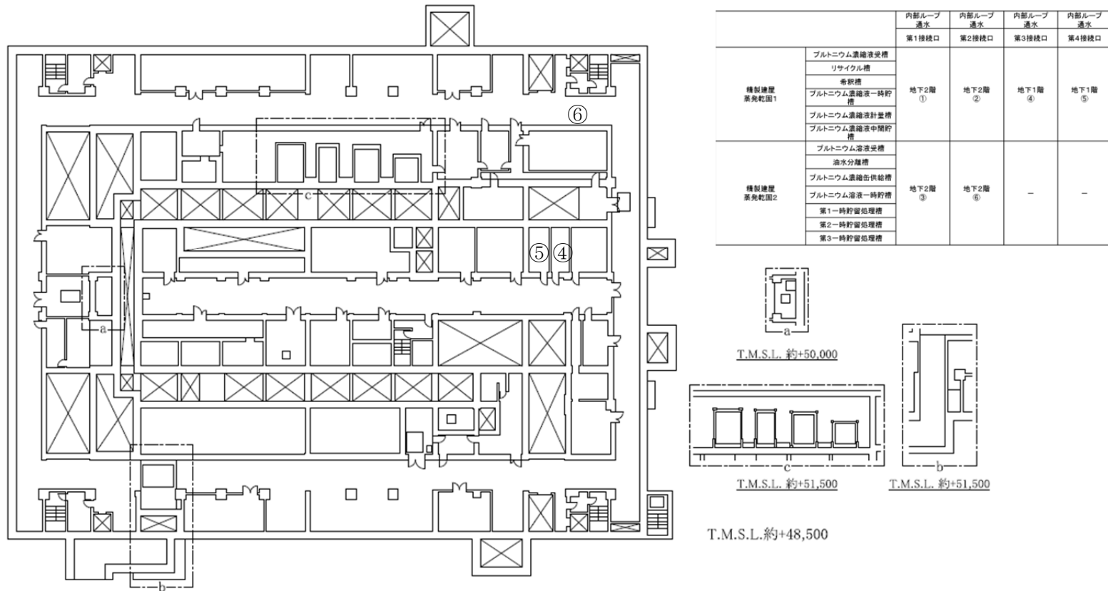
第 30 図 「精製建屋の冷却機能喪失事故」の機器注水接続口配置図（地下 2 階）
