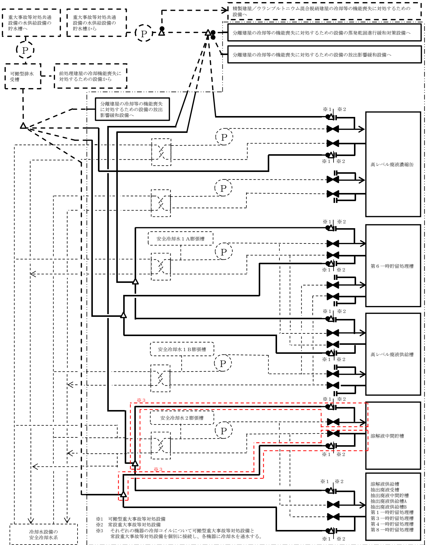
第19図 「分離建屋の冷却機能喪失事故」の冷却コイル又は冷却ジャケット通水系統概要図
