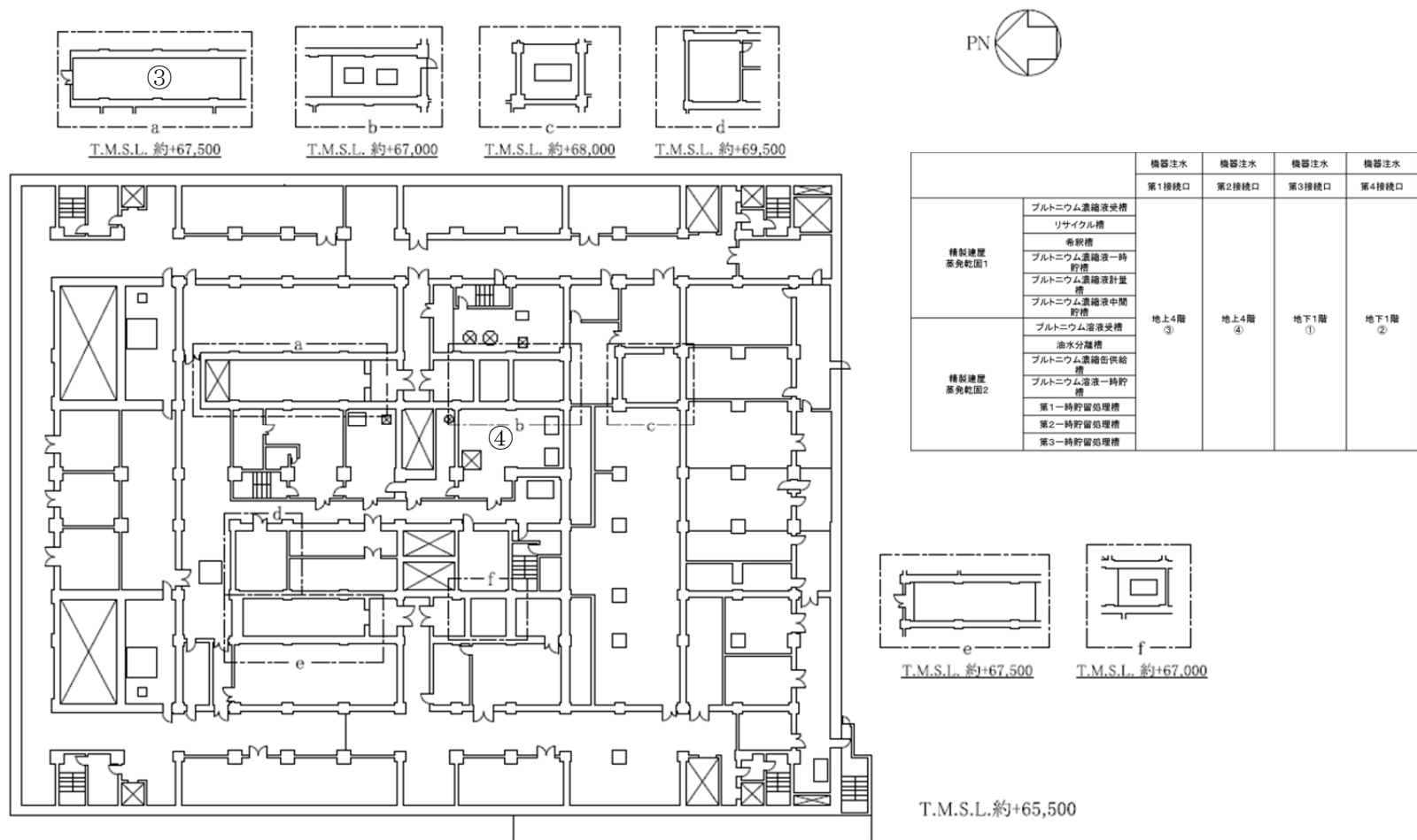
第 33 図 「精製建屋の冷却機能喪失事故」の機器注水接続口配置図（地上 4 階）
