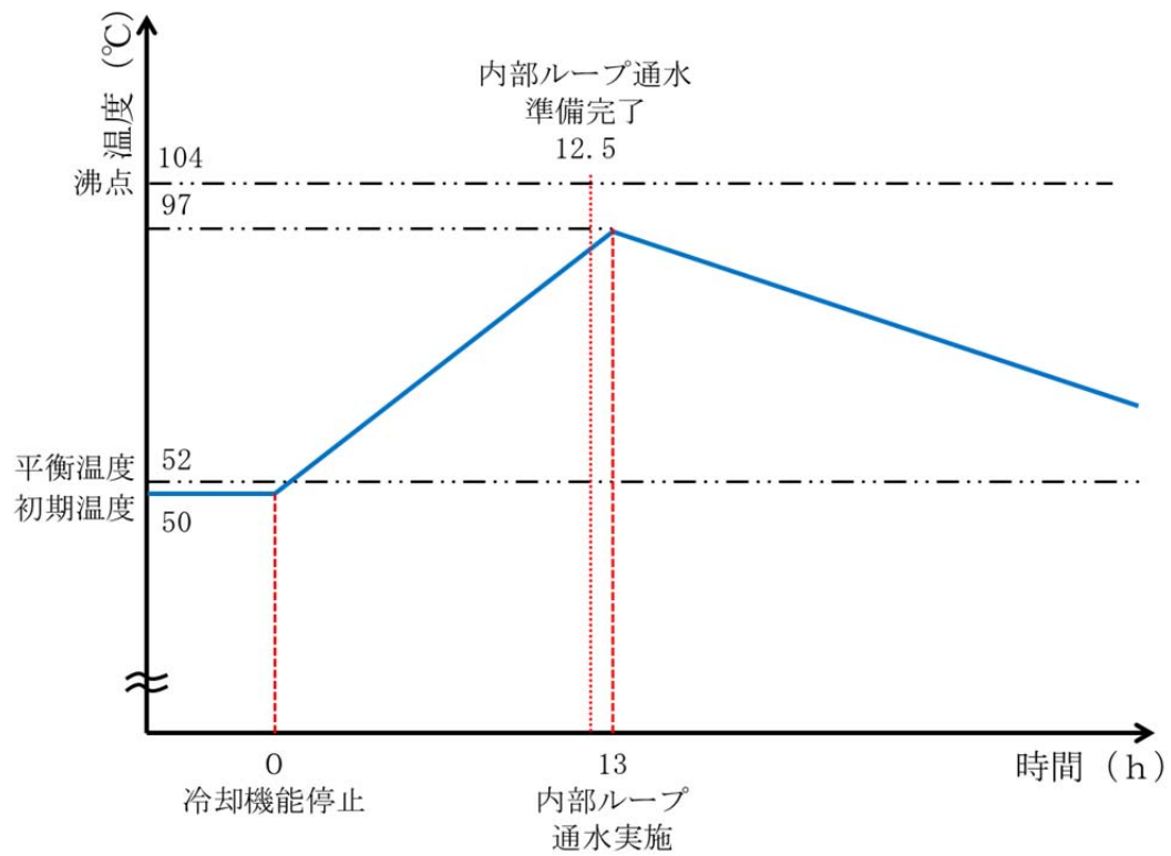
第 86 図 内部ループ通水実施時の高レベル廃液濃縮缶に内包する溶液の温度傾向
