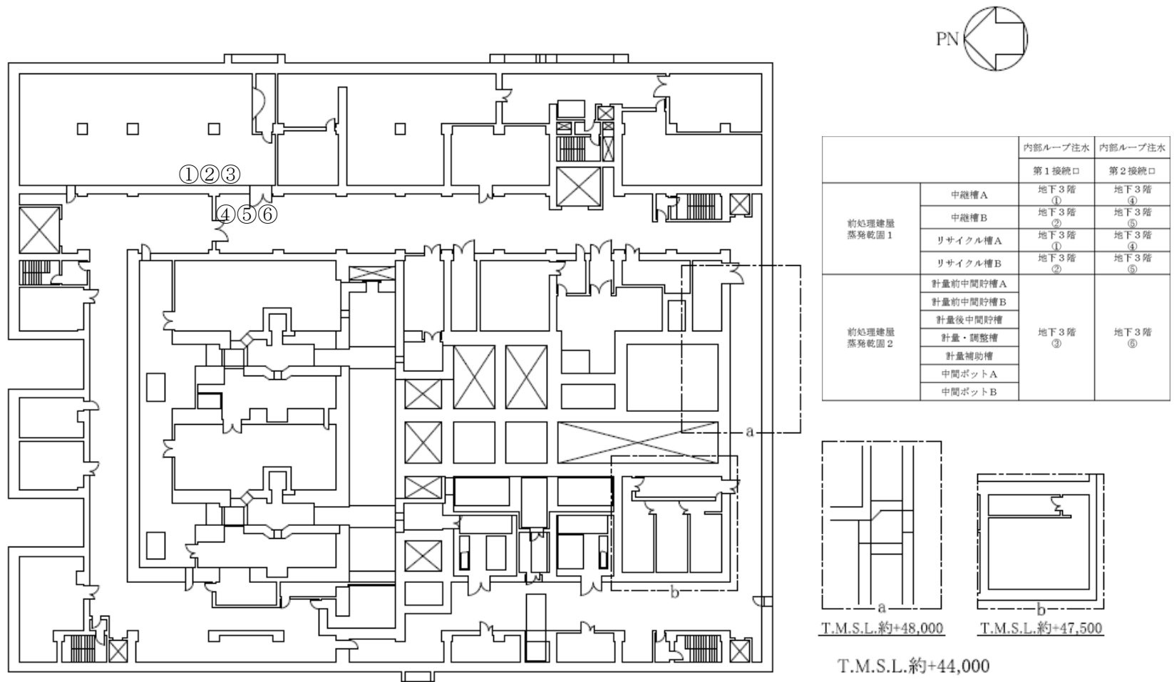
第2図 「前処理建屋の冷却機能喪失事故」の内部ループ注水接続口配置図（地下3階）
