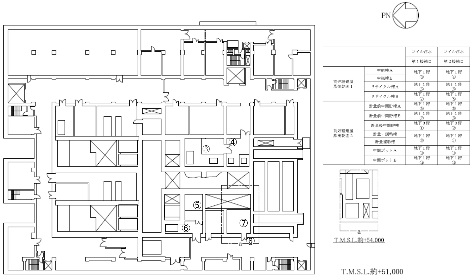
第8図 「前処理建屋の冷却機能喪失事故」の冷却コイル注水接続口配置図（地下1階）
