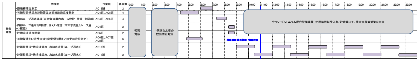
第69図 精製建屋における内部ループへの通水に必要な要員及び作業項目
