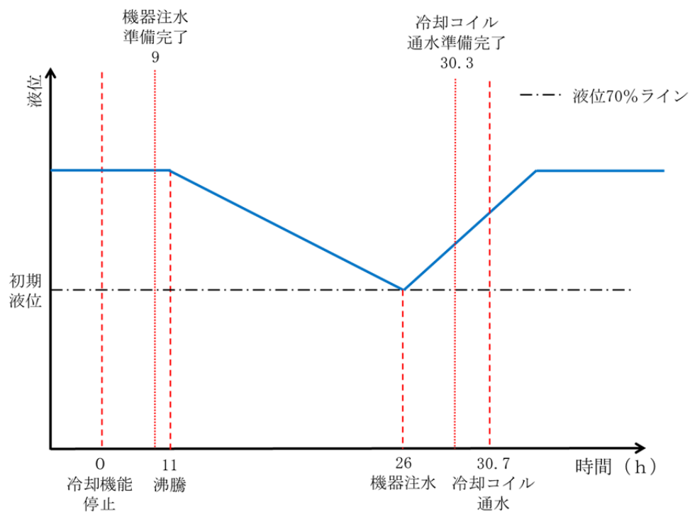
第 91 図 冷却コイル等通水及び機器注水実施時のプルトニウム濃縮液一時貯槽に内包する溶液の温度及び液位傾向
