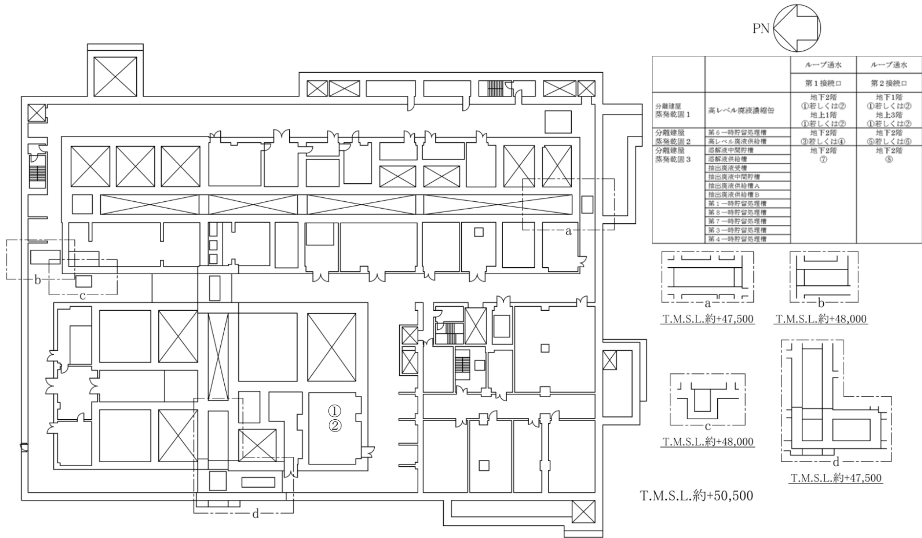
第14図 「分離建屋の冷却機能喪失事故」のループ通水接続口配置図（地下1階）
