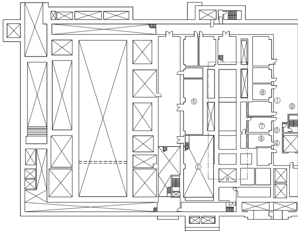
第54図 「高レベル廃液ガラス固化建屋の冷却機能喪失事故」の機器注水接続口配置図（地下2階）
