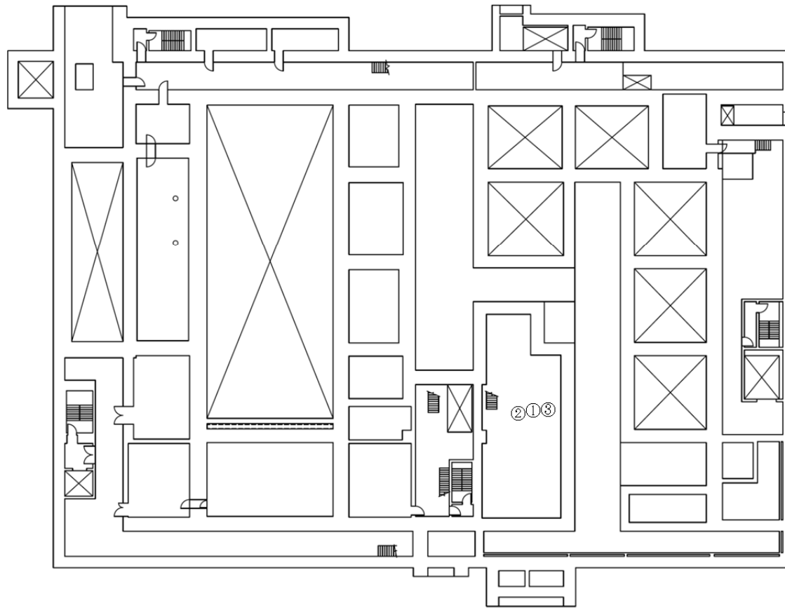
第53図 「高レベル廃液ガラス固化建屋の冷却機能喪失事故」の機器注水接続口配置図（地下3階）
