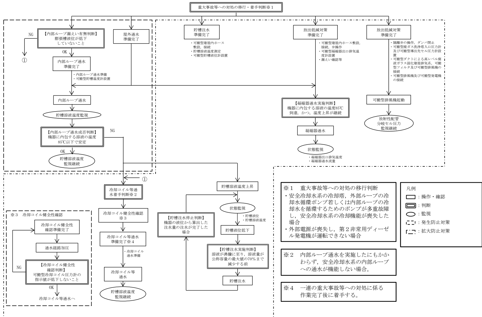
第66図 「地震発生による全交流動力電源の喪失を伴う高レベル廃液ガラス固化建屋の冷却機能喪失事故」の手順の概要
