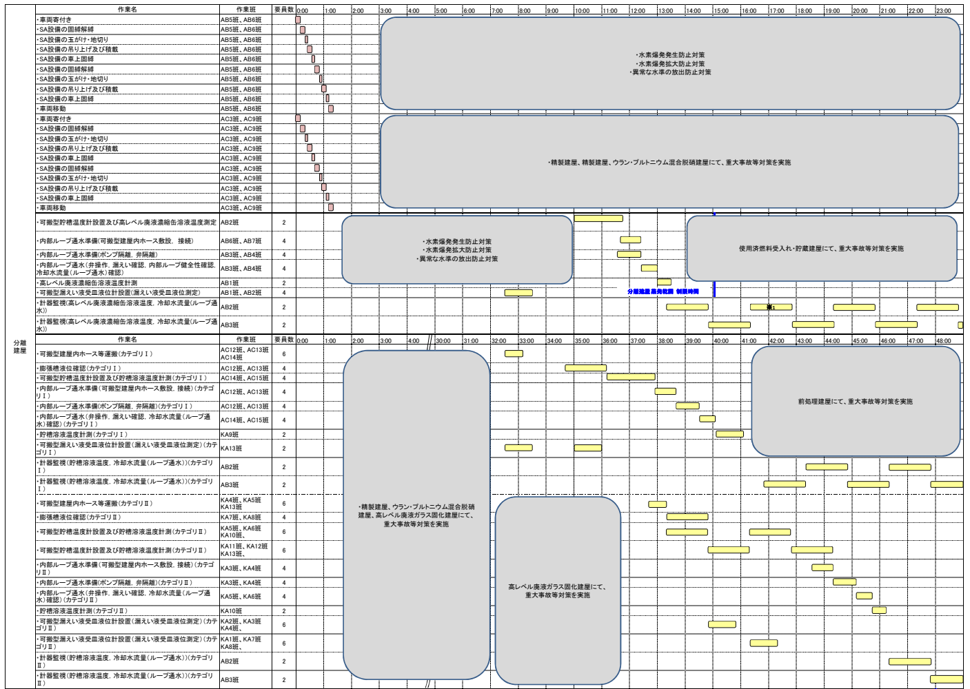
第73図 火山を想定した場合の分離建屋における内部ループへの通水に必要な要員及び作業項目
