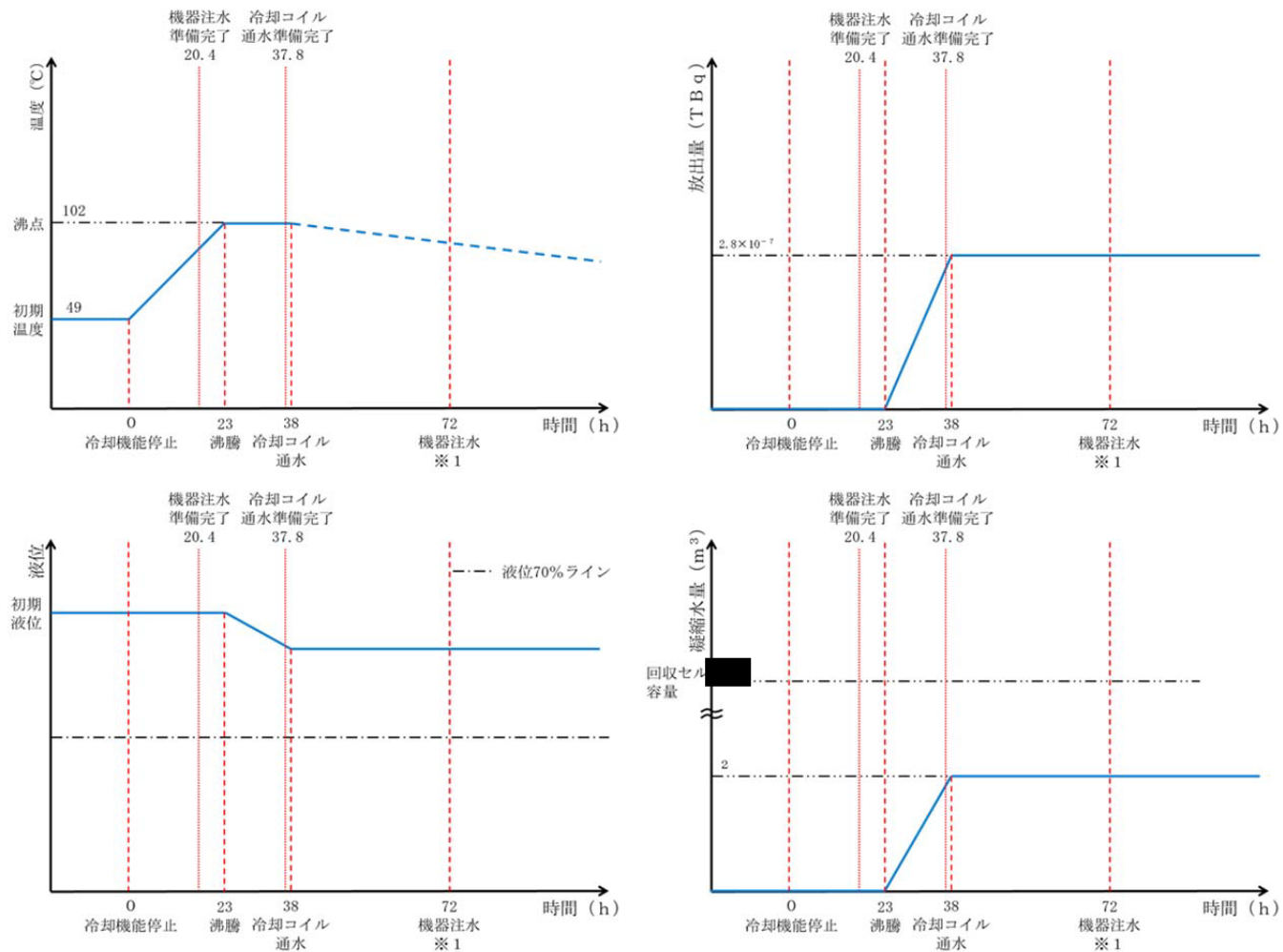
第 100 図 放出低減対策実施時の高レベル廃液混合槽に 内包する溶液の温度、液位、放出及び蒸気の凝縮傾向
