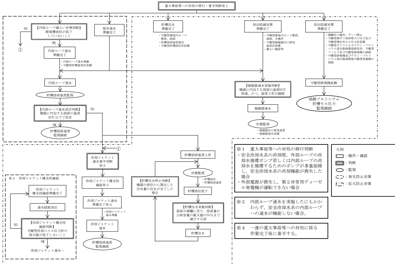
第65図 「地震発生による全交流動力電源の喪失を伴うウラン・プルトニウム混合脱硝建屋の冷却機能喪失事故」の手順の概要
