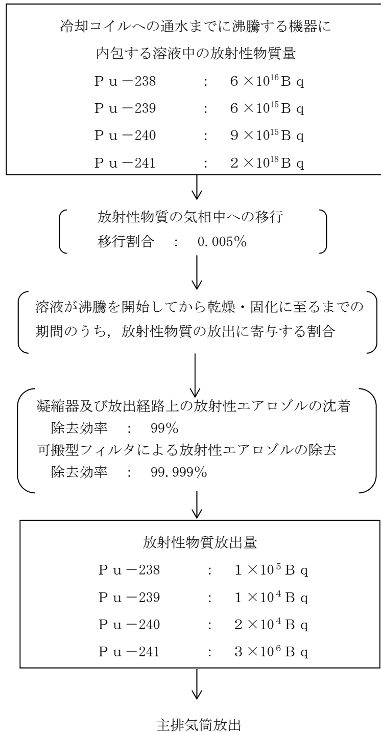
第 103 図 「地震発生による全交流動力電源の喪失を伴う精製建屋の冷却機能喪失事故」時の放射性物質の大気放出過程
