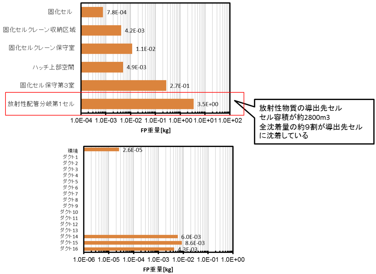
第 4. - 6 図 放出経路沈着量 (7 日目)
