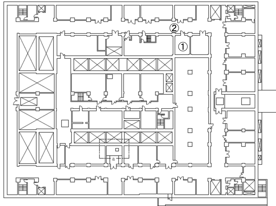
第 39 図 「精製建屋の冷却機能喪失事故」の冷却コイル通水接続口配置図（地上 2 階）
