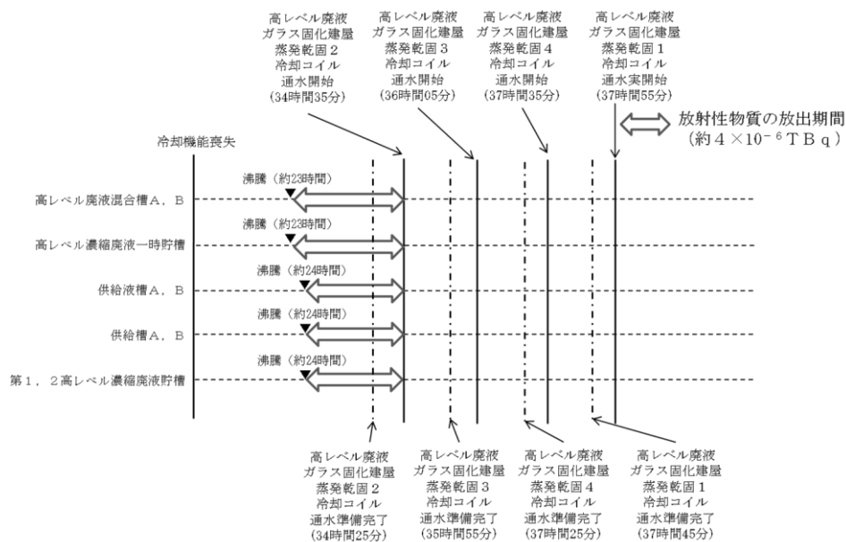
第 1. - 5 図 高レベル廃液ガラス固化建屋の放出量評価の前提
