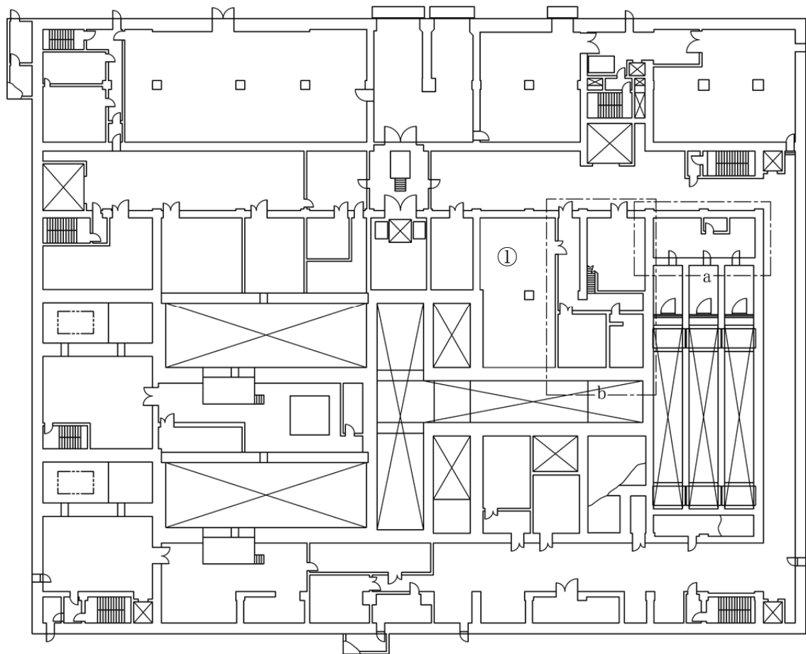
第4図 「前処理建屋の冷却機能喪失事故」の機器注水接続口配置図（地上1階）
