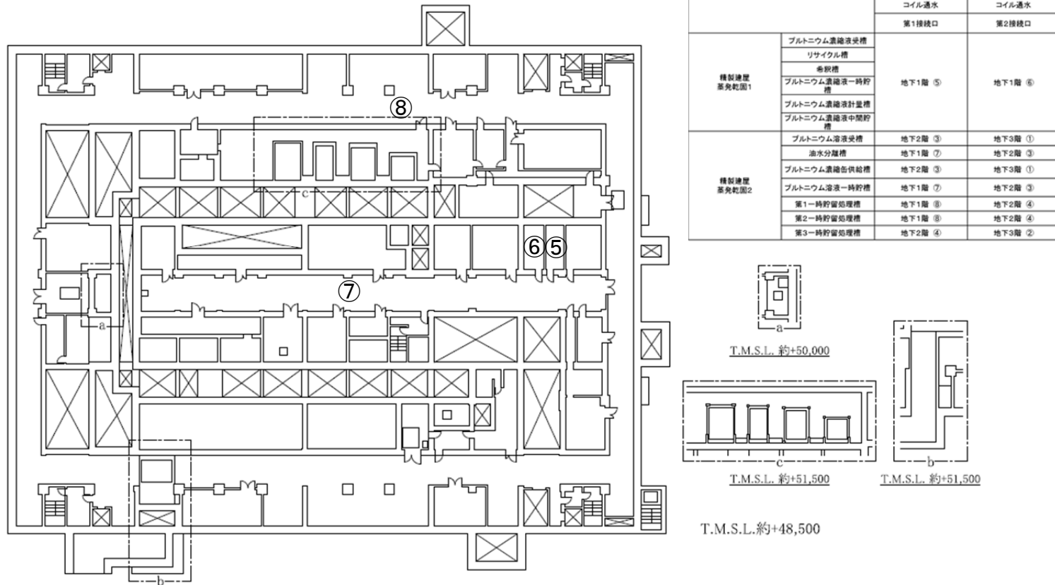
第 37 図 「精製建屋の冷却機能喪失事故」の冷却コイル通水接続口配置図（地下 1 階）
