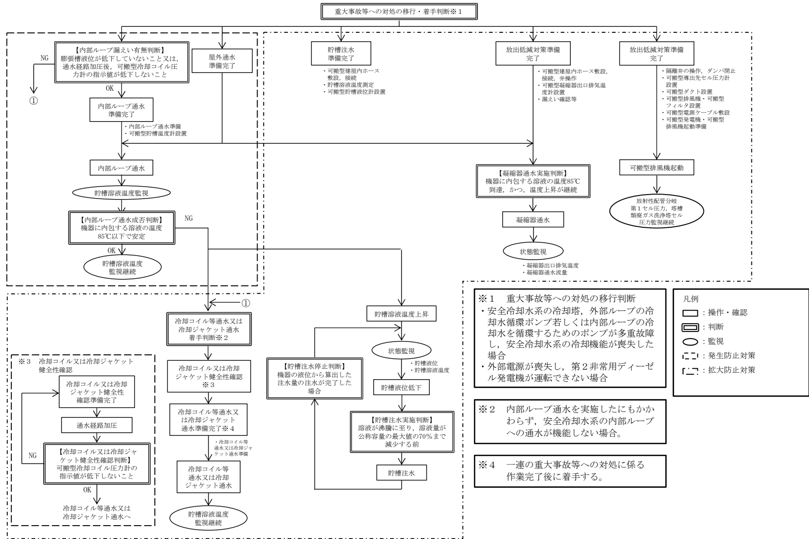
第63図 「地震発生による全交流動力電源の喪失を伴う分離建屋の冷却機能喪失事故」の手順の概要
