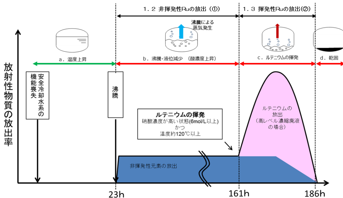
第 3. - 1 図 蒸発乾固の事象進展概要図
