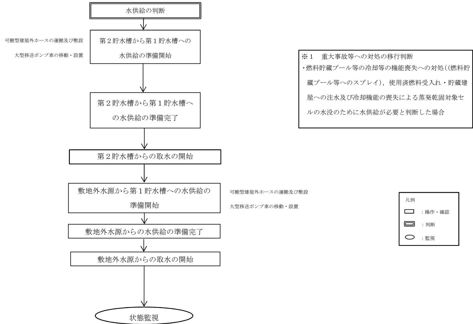
第 5.10.3.1-4 図 「水供給」 の手順の概要
