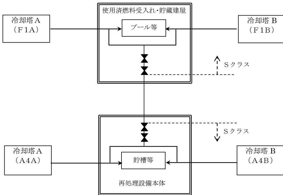
図 安全冷却水系の概要図（使用済燃料受入れ施設・貯蔵施設からのバックアップ）
