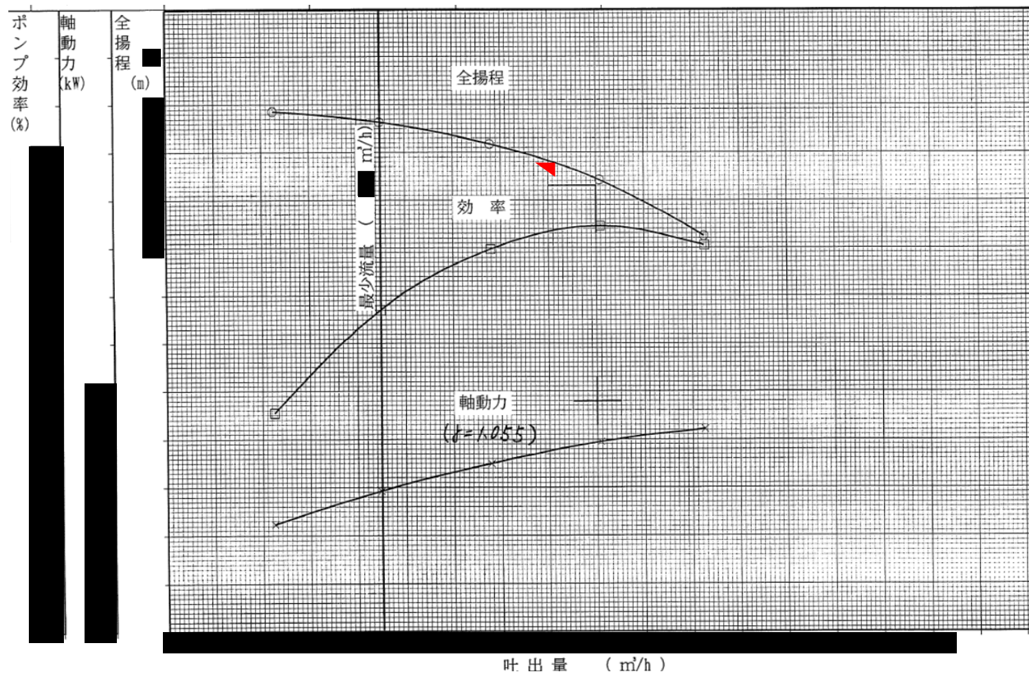
第1図 冷却水循環ポンプA, Bの流量と揚程
