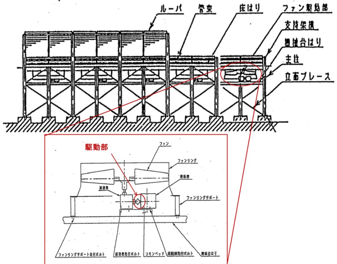
第 8 図 冷却塔の主要な駆動部の防滴構造の概要図
