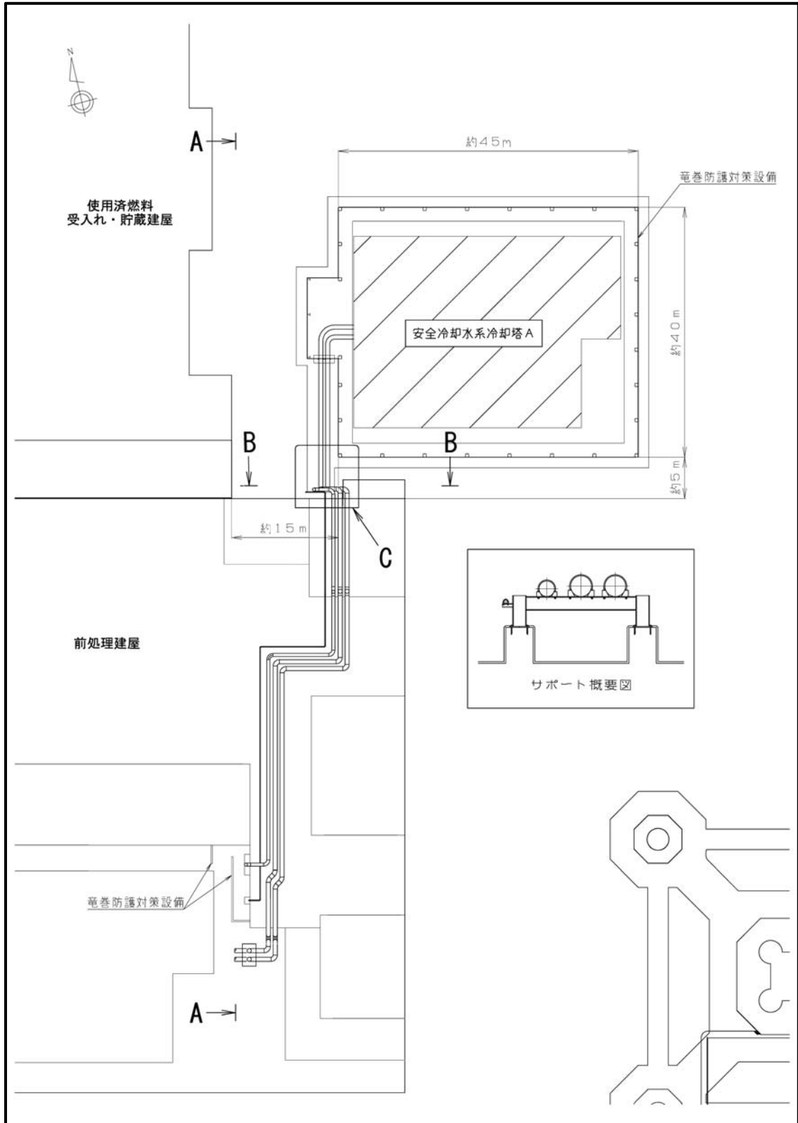
図 安全冷却水系冷却塔 A 全体配管ルート
