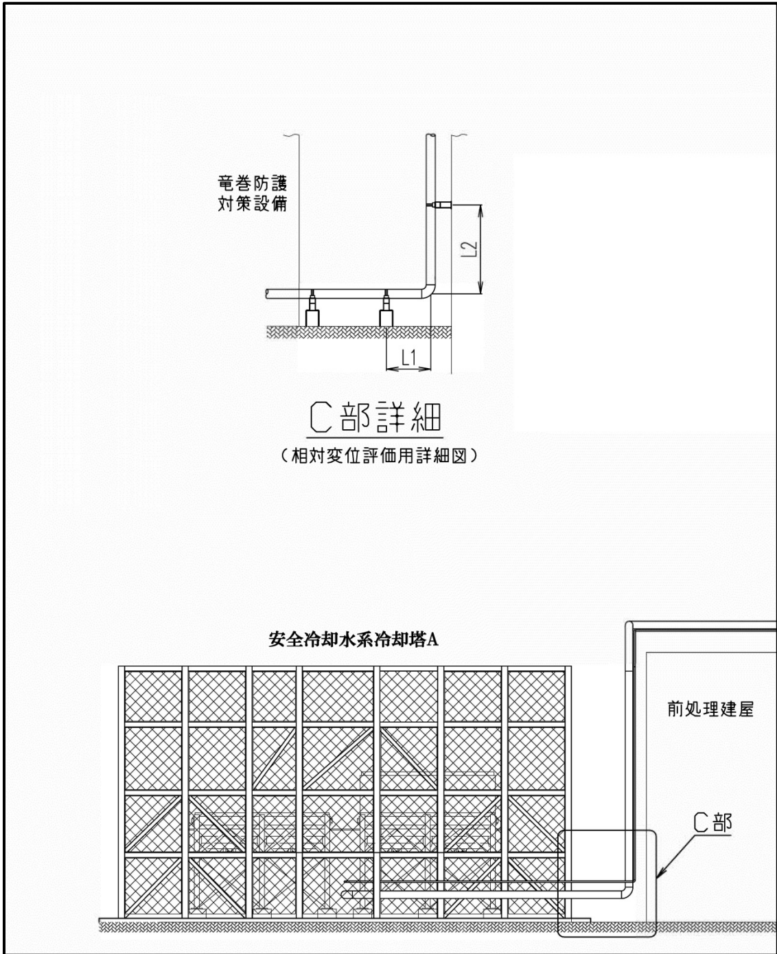
図 安全冷却水系冷却塔 A 配管ルート (冷却塔周辺) (断面)
