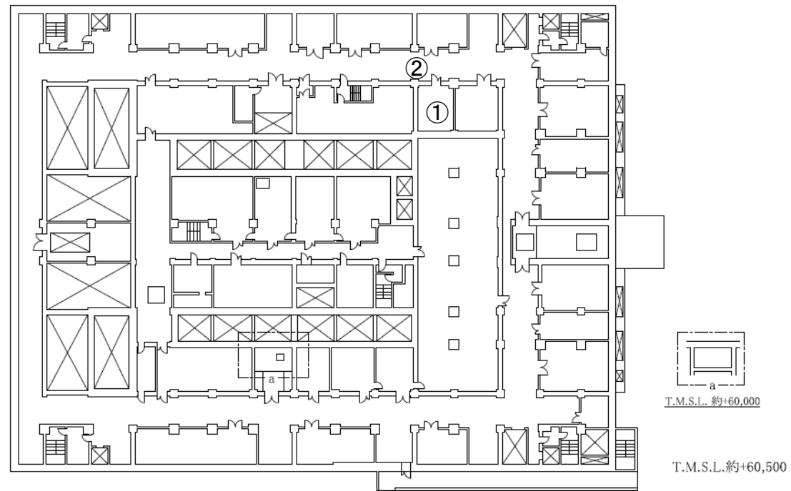
「精製建屋の冷却機能喪失事故」の冷却コイル通水接続口配置図（地上2階）
