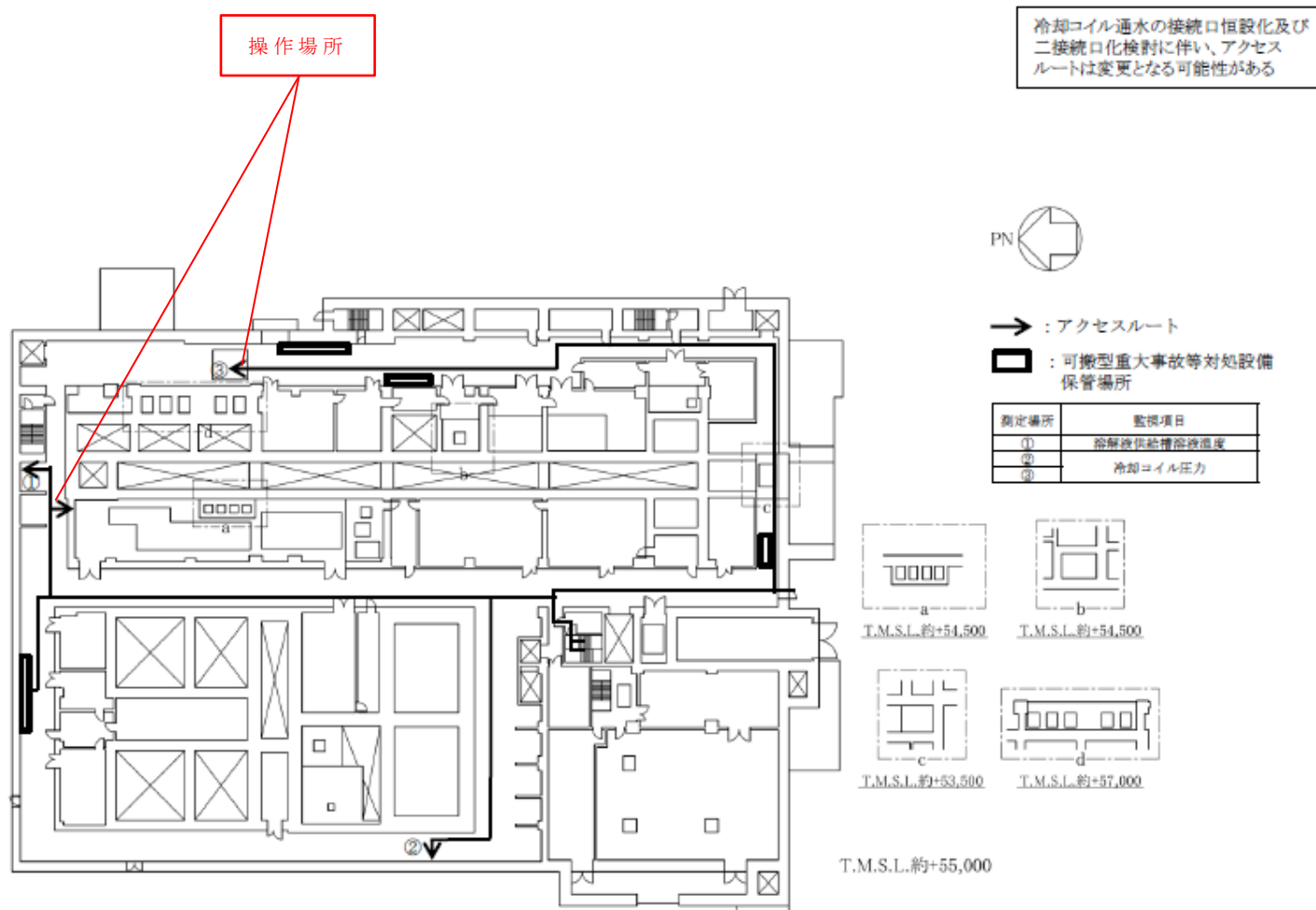
分離建屋 蒸発乾固の拡大の防止のための措置のアクセスルート（南ルート）（地上1階）（冷却コイル通水による冷却）
