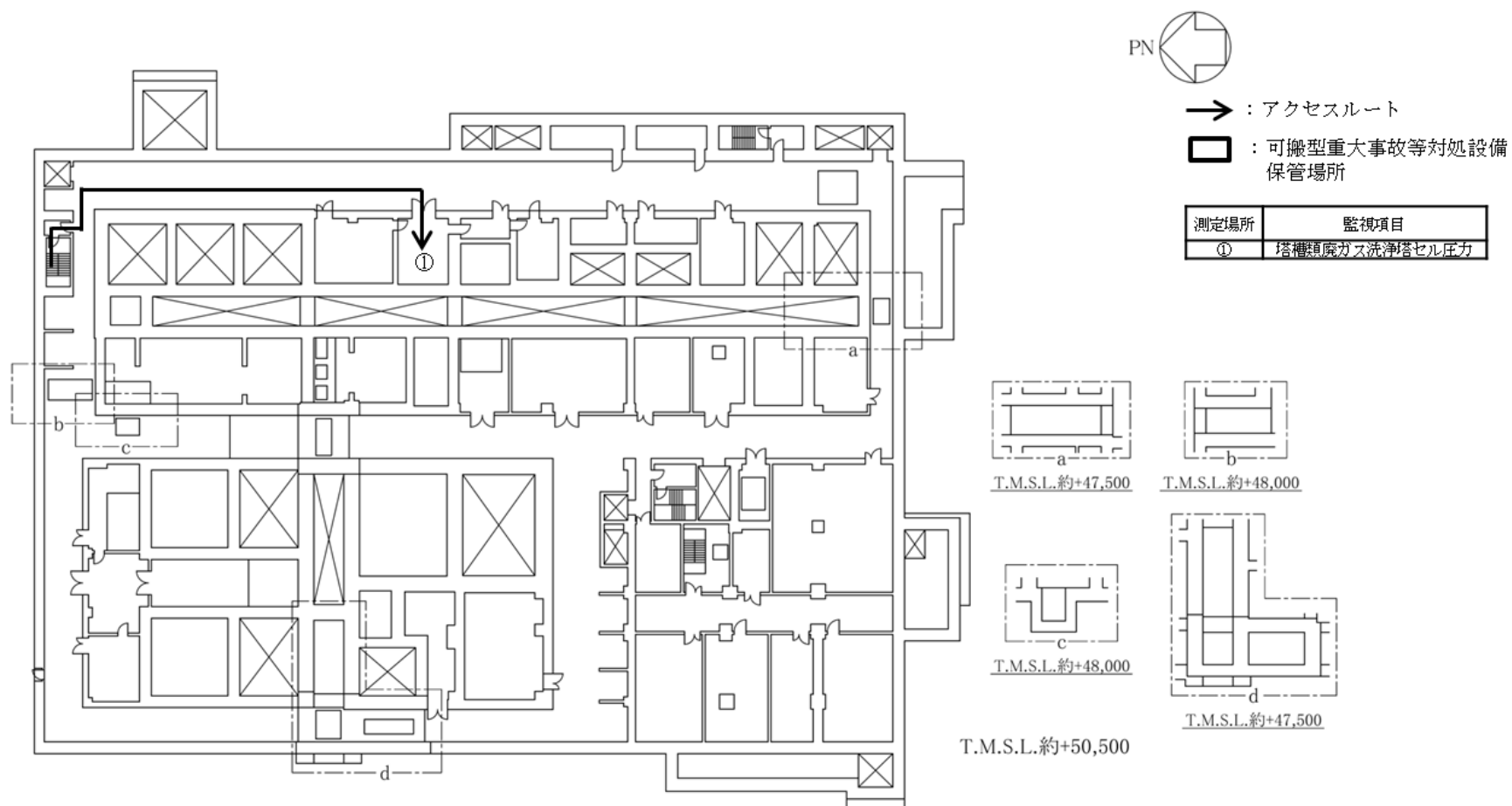
分離建屋 蒸発乾固の拡大の防止のための措置のアクセスルート（東ルート）（地下1階）（放出低減対策）
