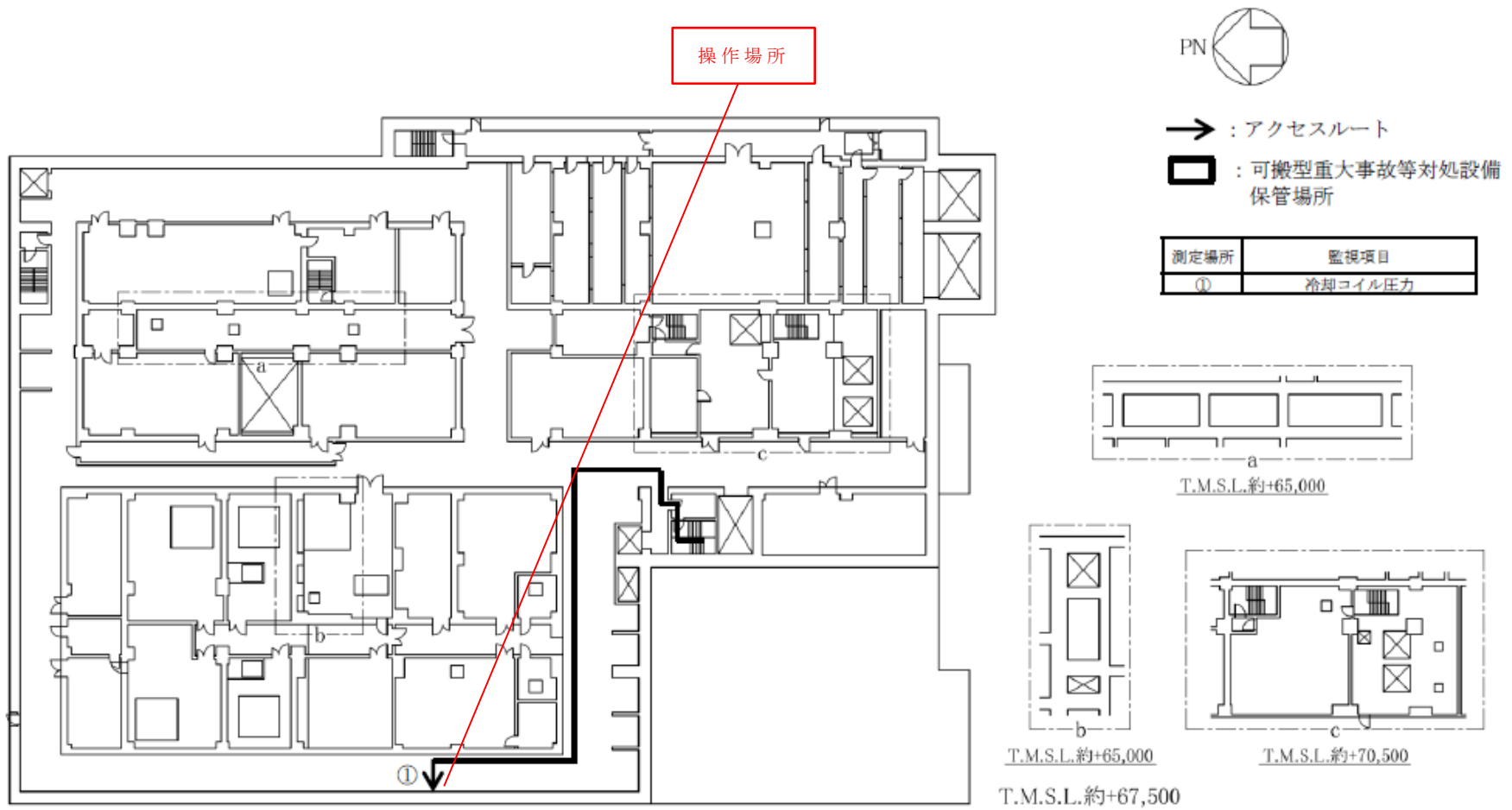
分離建屋 蒸発乾固の拡大の防止のための措置のアクセスルート（南ルート）（地上3階）（冷却コイル通水による冷却）
