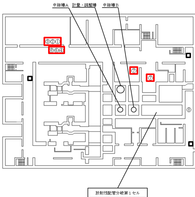
未然防止設備 安全冷却水系内部ループ通水 第1接続口（給水口及び排水口）
