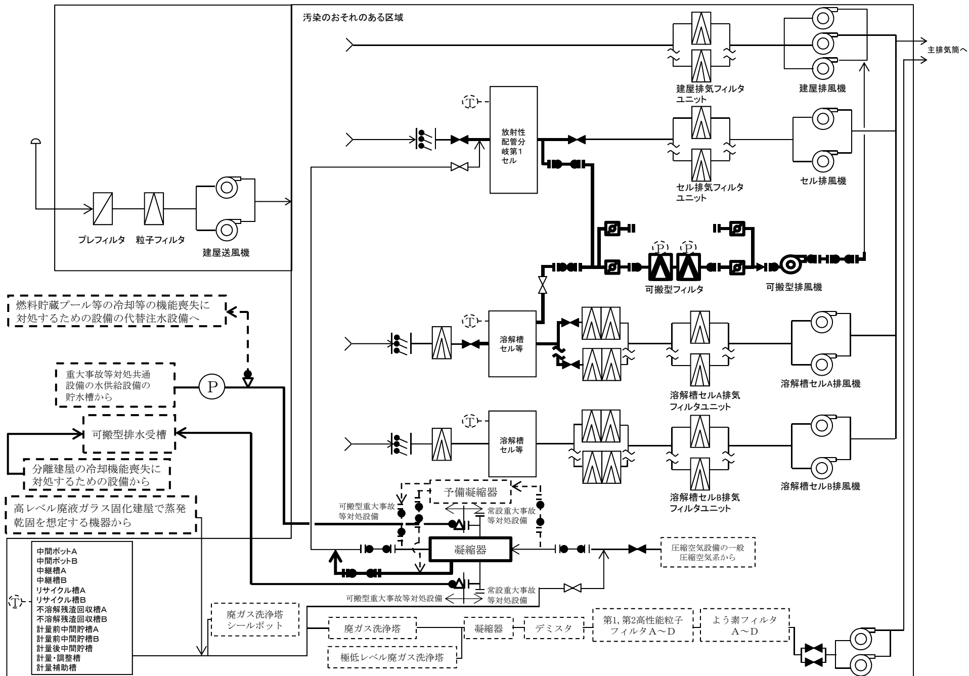
第10図 「前処理建屋の冷却機能喪失事故」の換気系統遮断・セル内導出及び放出影響緩和系統概要図
