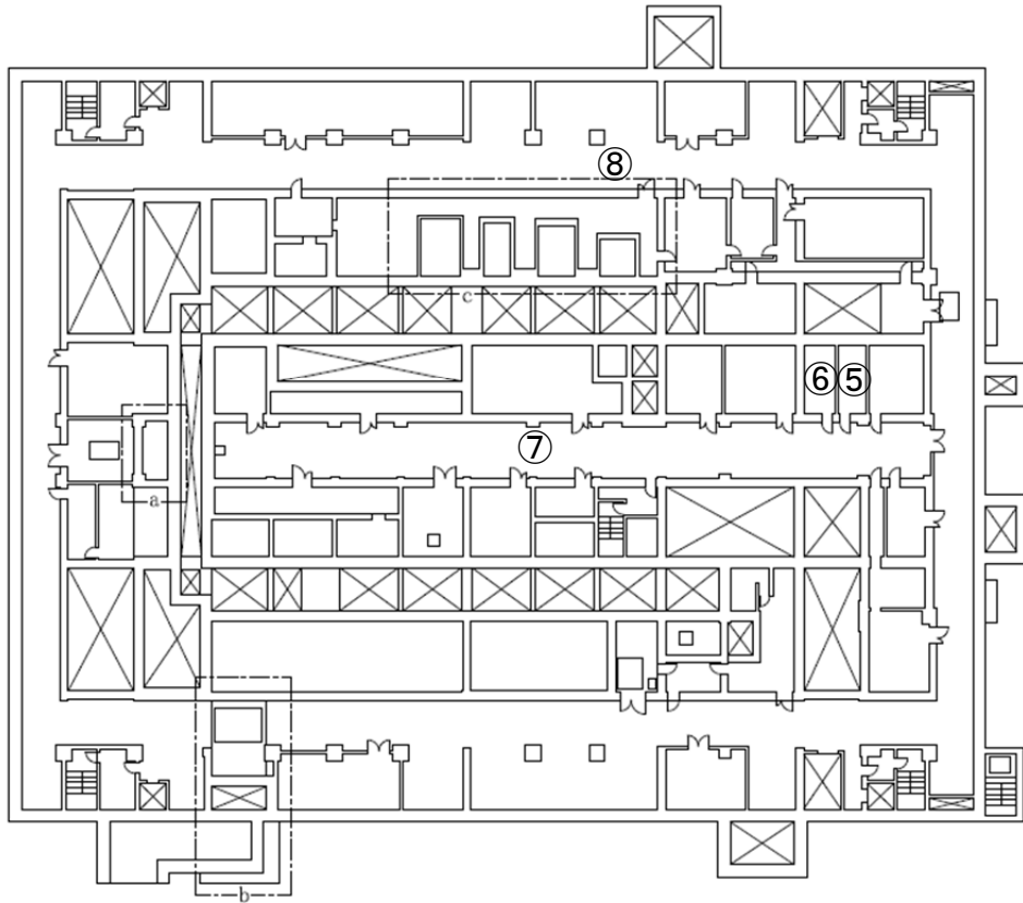
第 37 図 「精製建屋の冷却機能喪失事故」の冷却コイル通水接続口配置図（地下 1 階）
