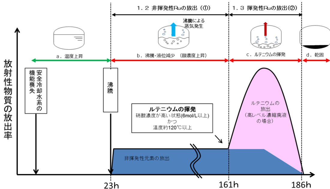
第 3. - 1 図 蒸発乾固の事象進展概要図
