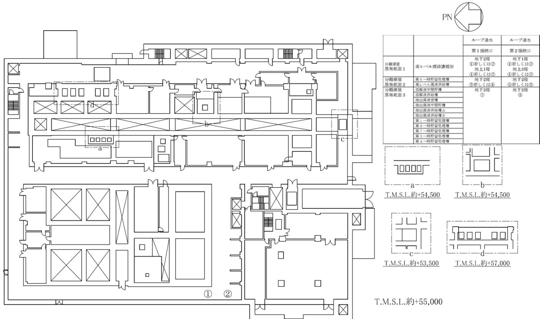
第15図 「分離建屋の冷却機能喪失事故」のループ通水接続口配置図（地上1階）
