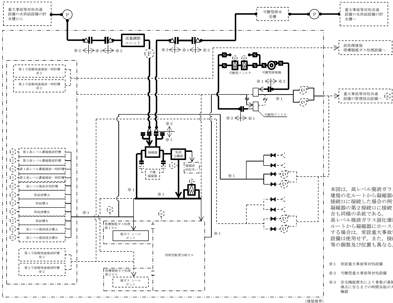
第60図 高レベル廃液ガラス固化建屋の蒸発乾固に対処するための設備の系統概要図 (異常な水準の放出防止)
