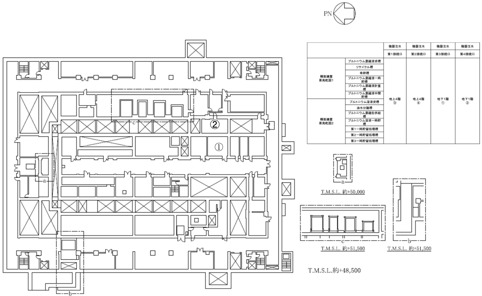
第 32 図 「精製建屋の冷却機能喪失事故」の機器注水接続口配置図（地上 1 階）
