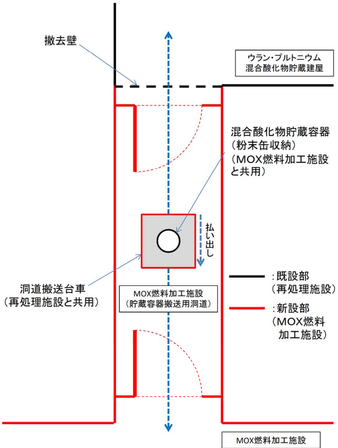
第1図 変更範囲に関する概要図
