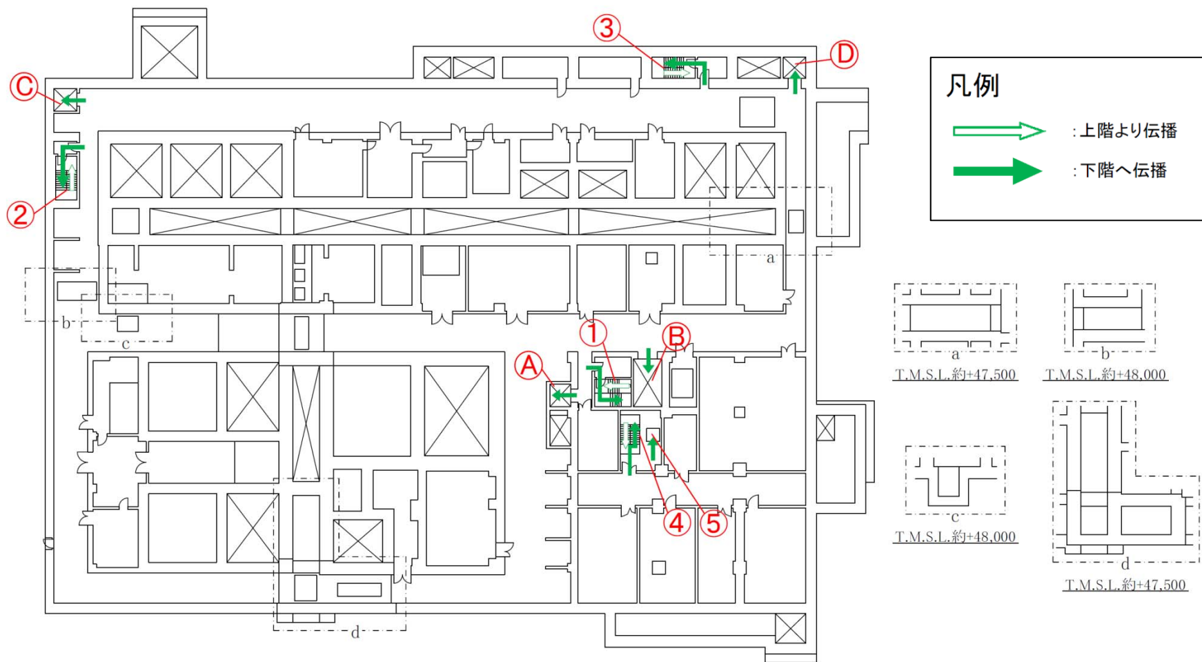
分離建屋 地下1階(EL. 50.29)
