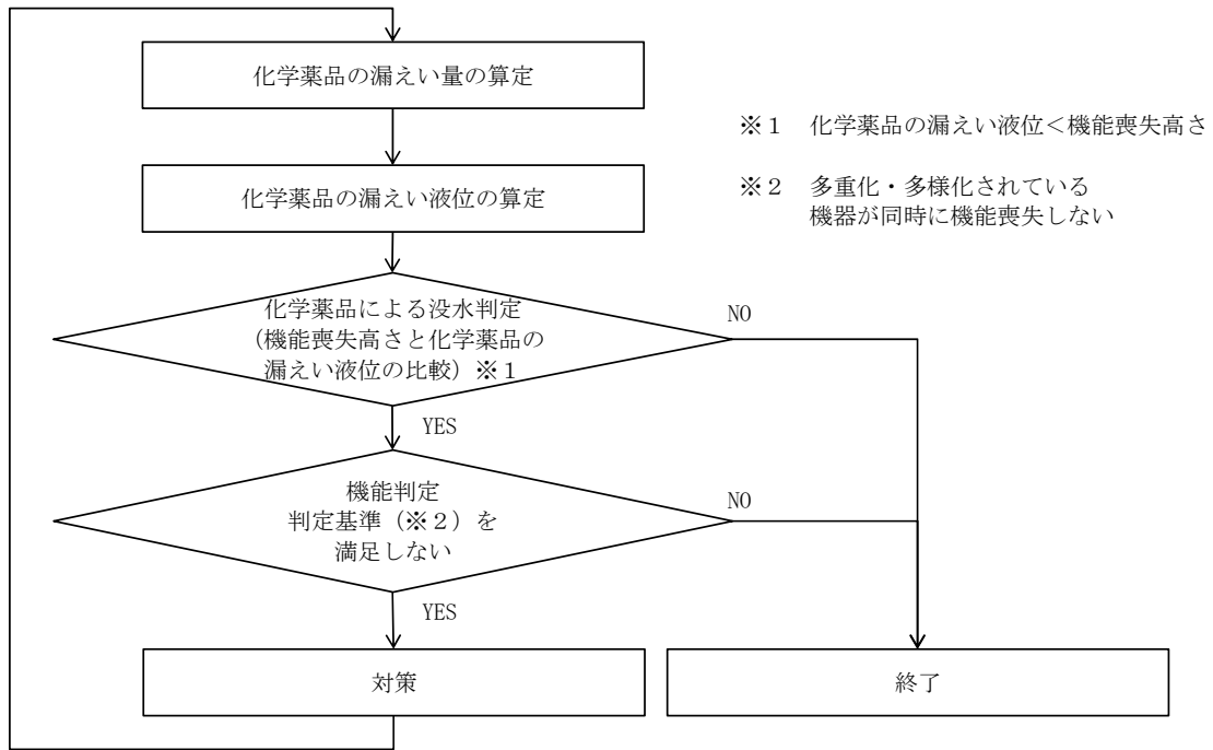
第 8.2-1 図 想定破損による化学薬品による没水影響評価フロー
