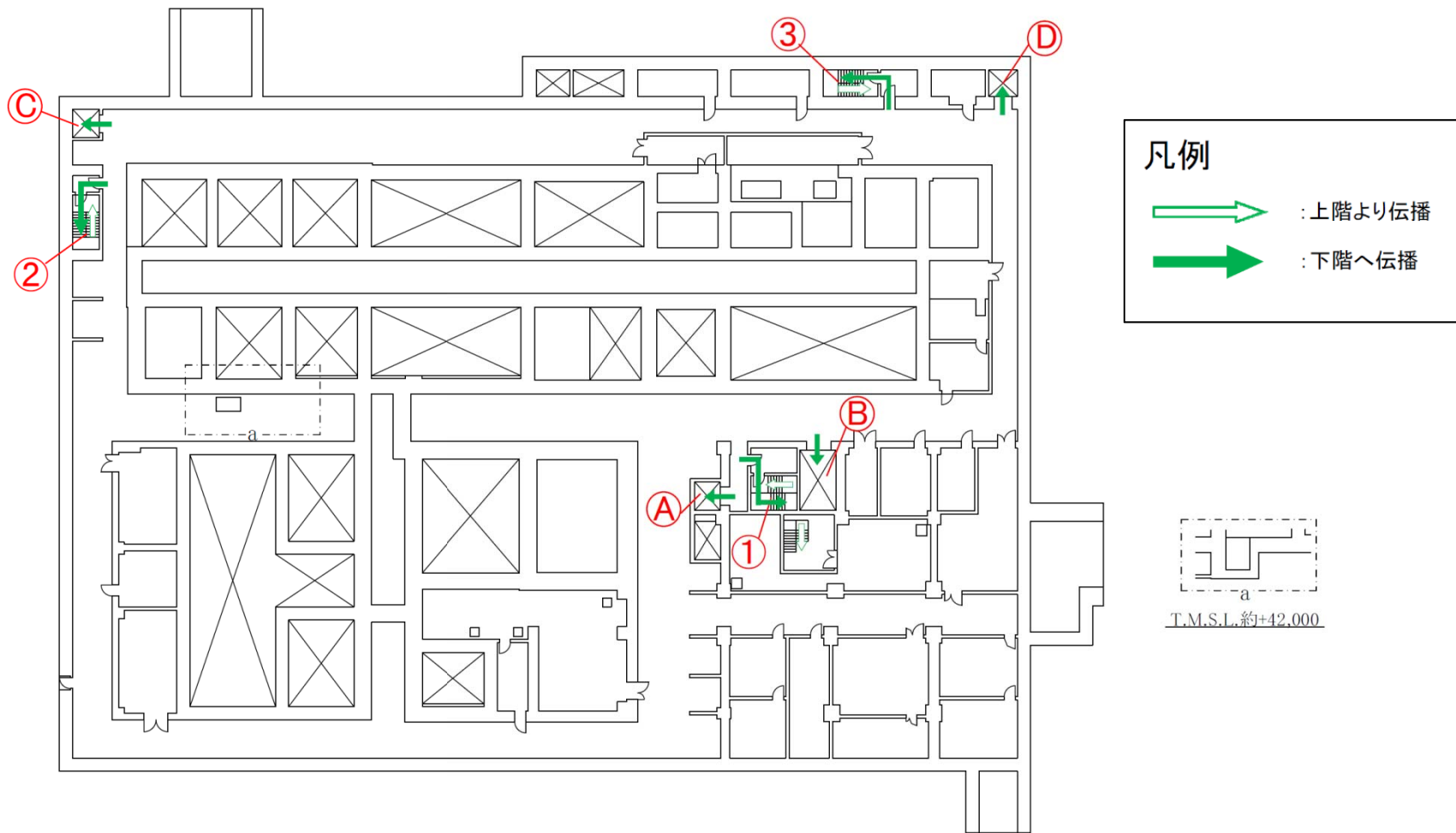
分離建屋 地下2階(EL. 43.49)
