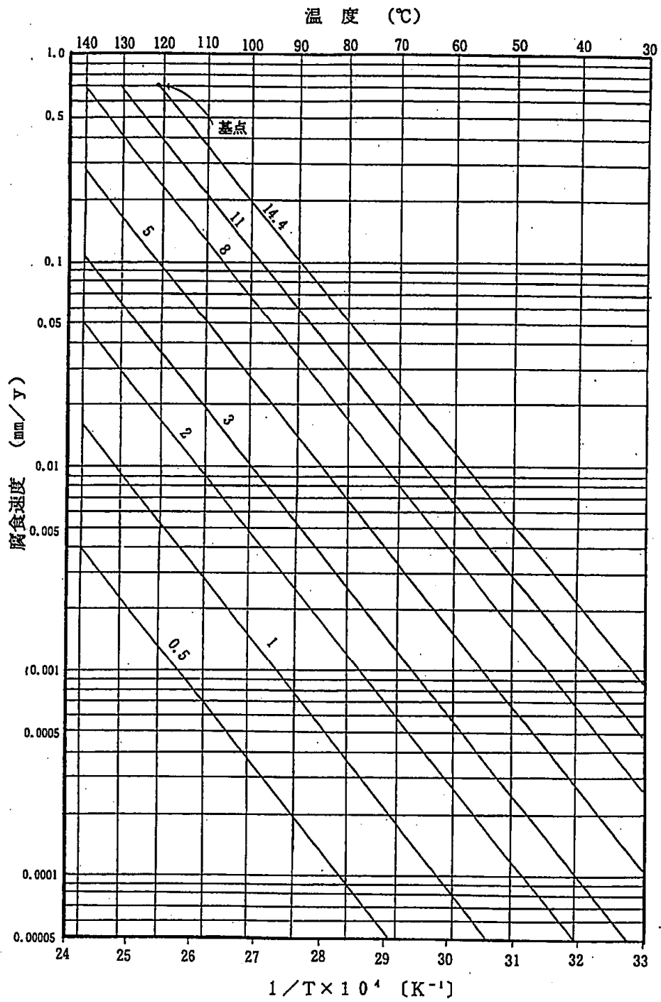
第4.4図 SUS304Lの腐食評価線図
