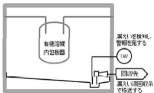
第3図 漏えい液回収系による回収
