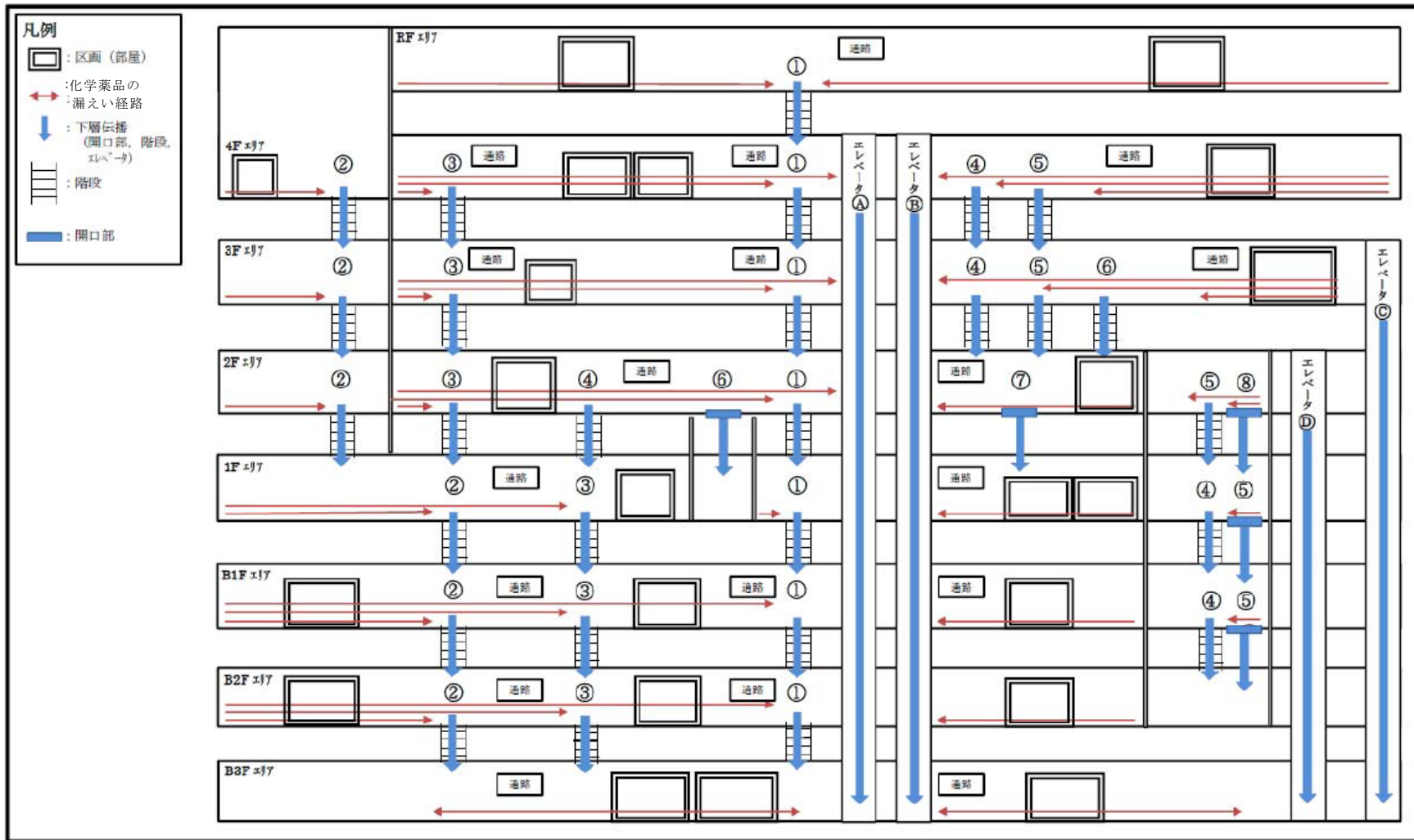
第 1 図 化学薬品の漏えい経路モデル図 代表例
