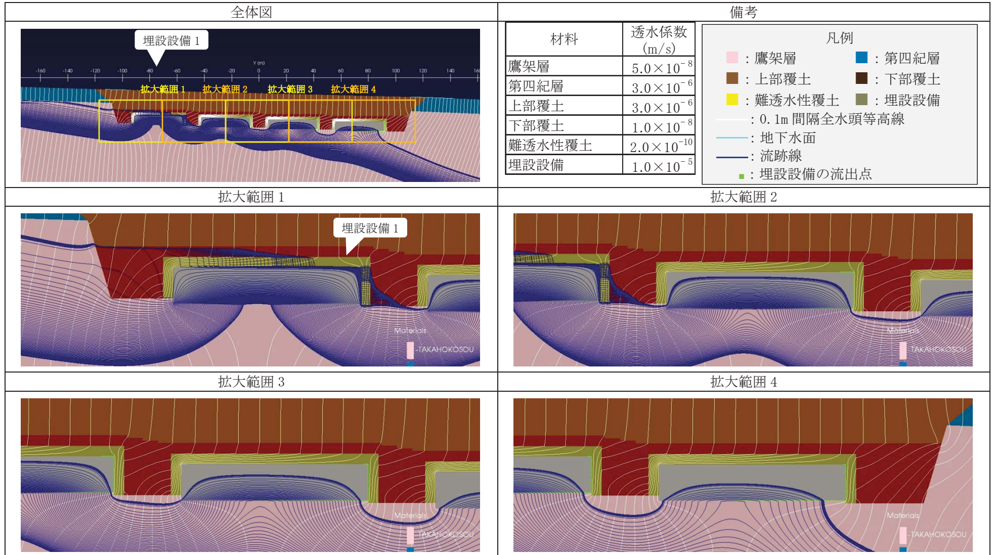
第1図 2次元地下水浸透流解析結果【3号廃棄物埋設地】(基本設定 1,000年後) (2/5) <埋設設備1の流出点を通る流跡線>
