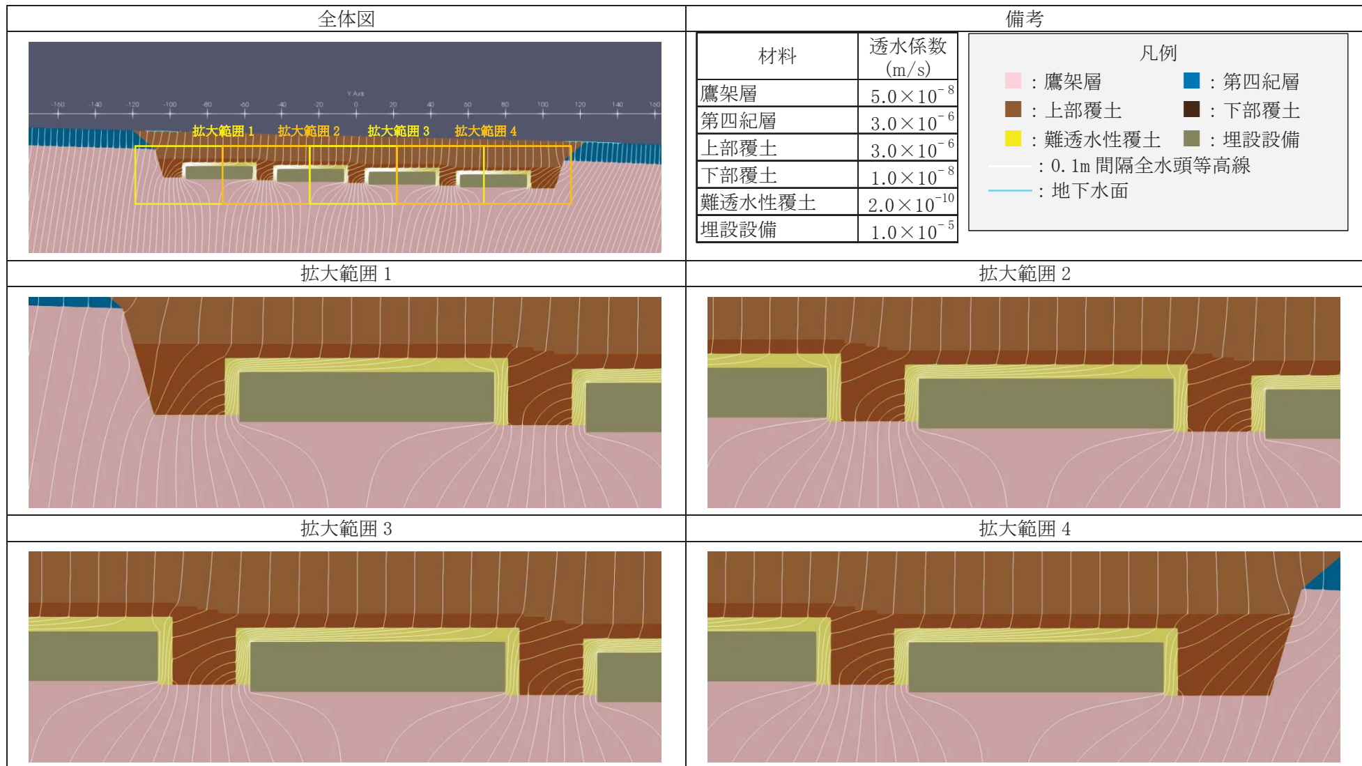
第1図 2次元地下水浸透流解析結果【3号廃棄物埋設地】(基本設定 1,000年後) (1/5) <0.1m 間隔全水頭等高線>
