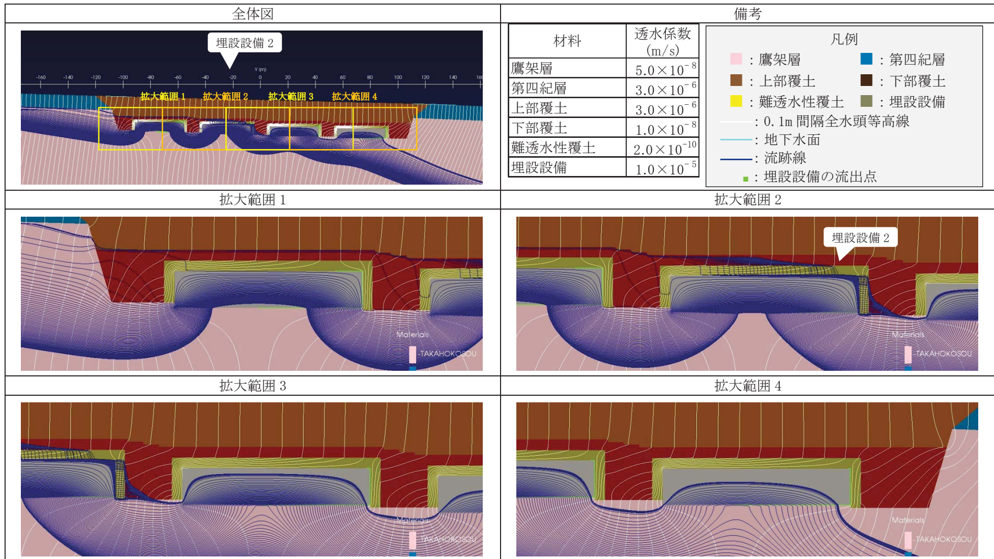
第1図 2次元地下水浸透流解析結果【3号廃棄物埋設地】(基本設定 1,000年後) (3/5) <埋設設備2の流出点を通る流跡線>
