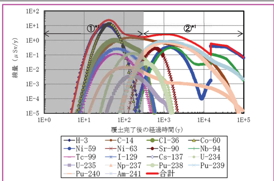
畜産業従事者：線量評価結果 (約 2.6E+00[ \mu Sv/年])
