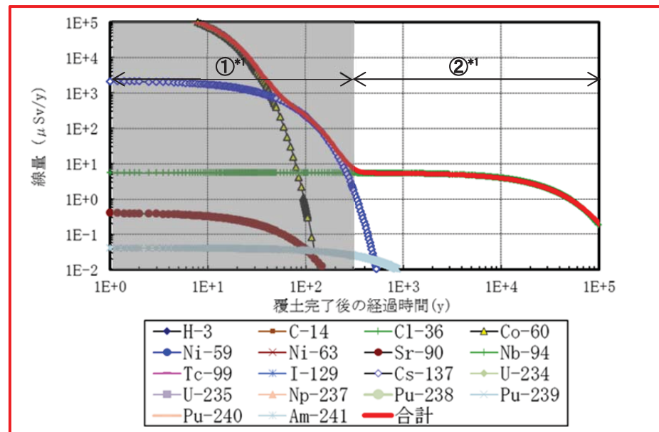
第 3 図 2 号廃棄物埋設施設における各シナリオの線量評価結果(3/3)
