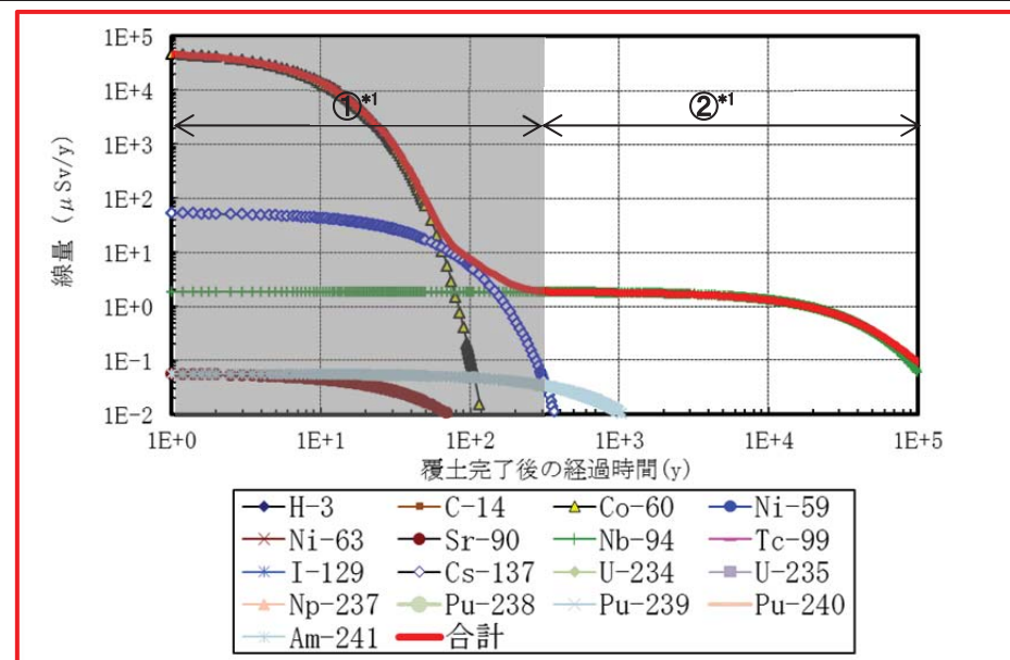
第 1 図 3 号廃棄物埋設施設における各シナリオの線量評価結果(3/3)
