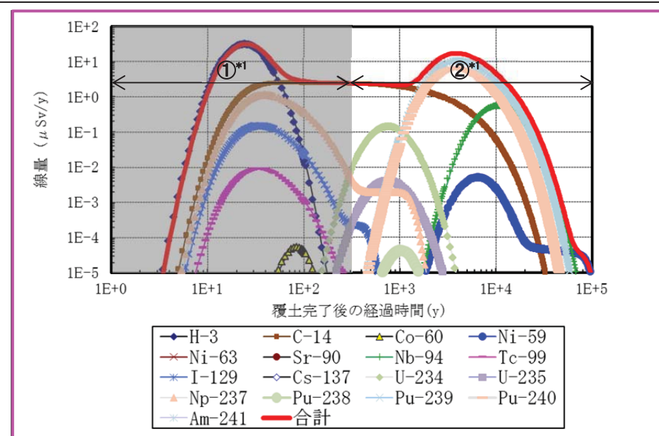
居住者：線量評価結果 (約 1.8E+01[ \mu Sv/年])
