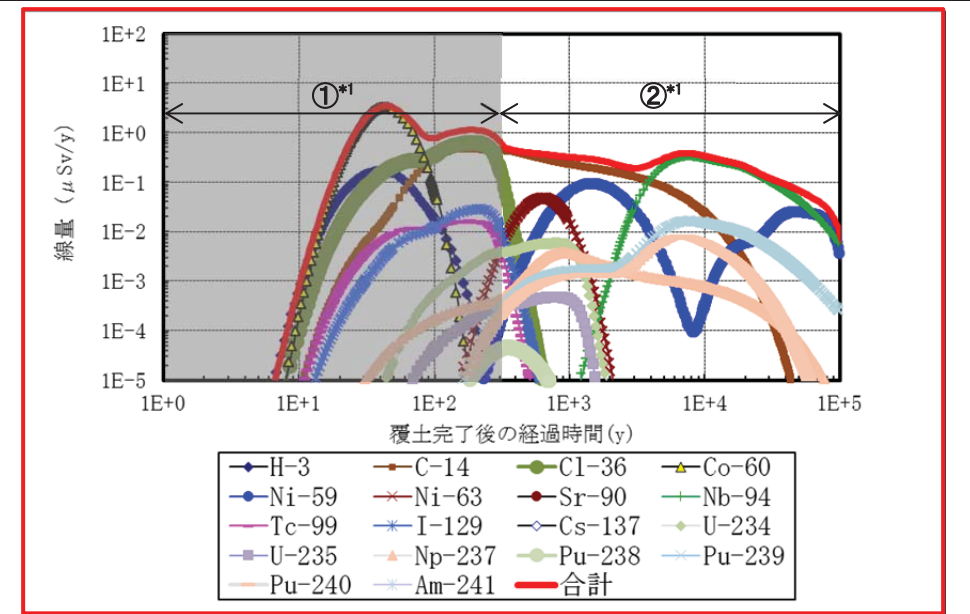
居住者：線量評価結果 (約 3.1E-01 [ \mu Sv/年])
