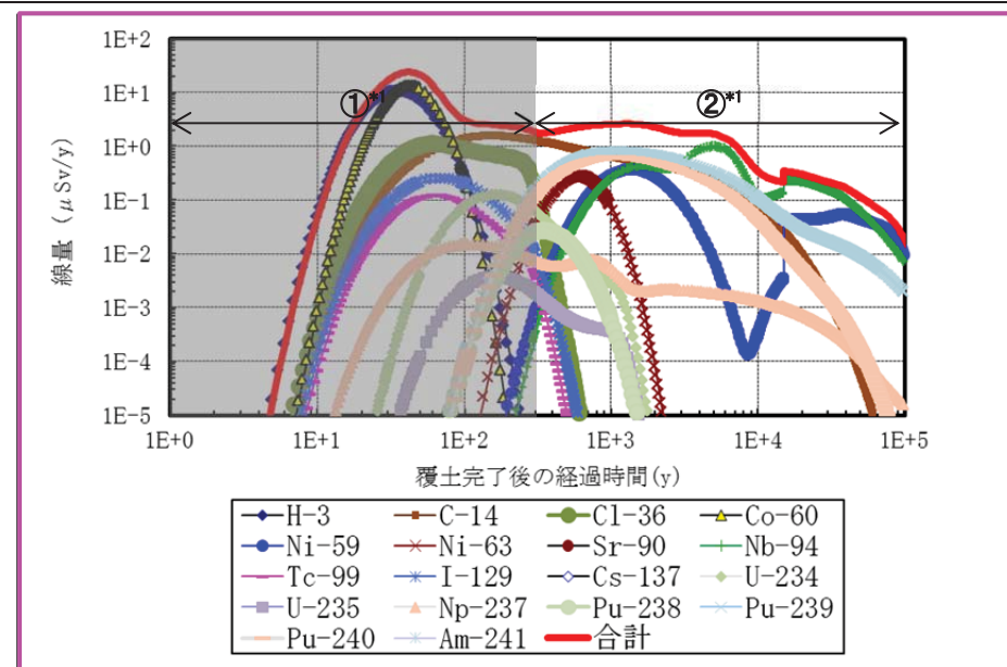
居住者：線量評価結果 (約 2.6E+00[ \mu Sv/年])
