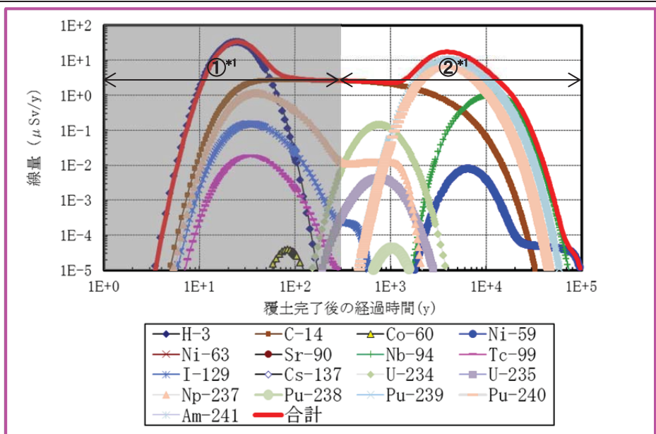
建設業従事者：線量評価結果 (約 1.8E+01[ \mu Sv/年])
