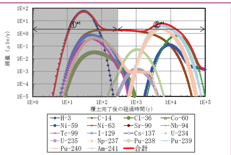
建設業従事者：線量評価結果 (約 6.3E+00[ \mu Sv/年])
