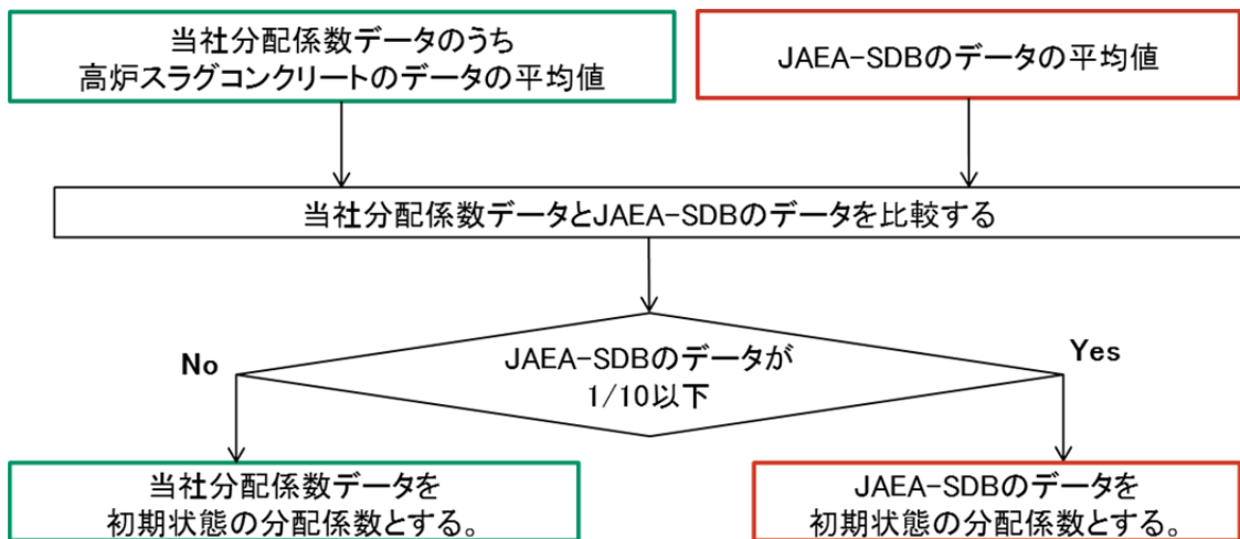
第8図 コンクリートの初期状態の分配係数の考え方(1号廃棄物埋施設(1群~6群))
