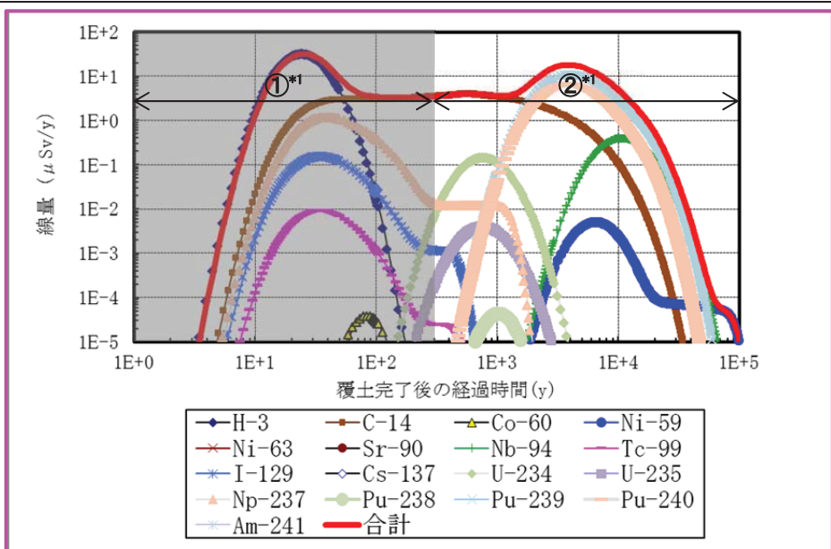
畜産業従事者：線量評価結果 (約 1.8E+01[ \mu Sv/年])
