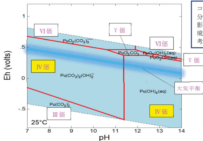
第 12 図 Pu の pH-Eh 図
