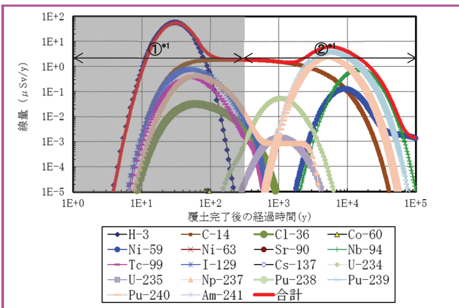
居住者：線量評価結果 (約 6.3E+00[ \mu Sv/年])
