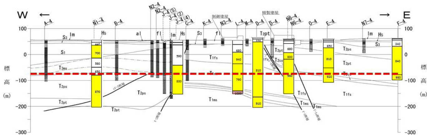
(a) EW-3 断面
