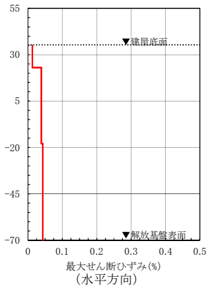
(d) 最大せん断ひずみ分布
