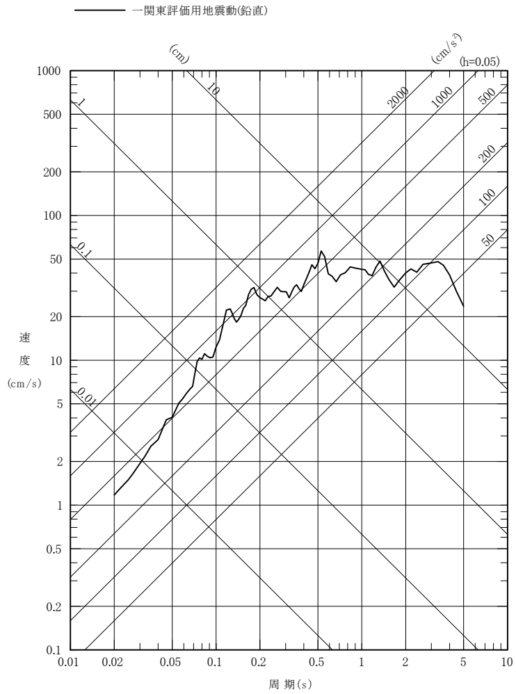
第 1.6-5 図 一関東評価用地震動（鉛直）の設計用応答スペクトル
