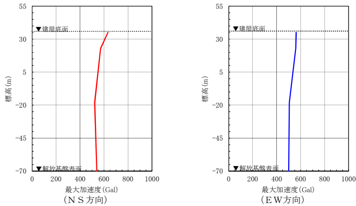
(c) 最大加速度分布
