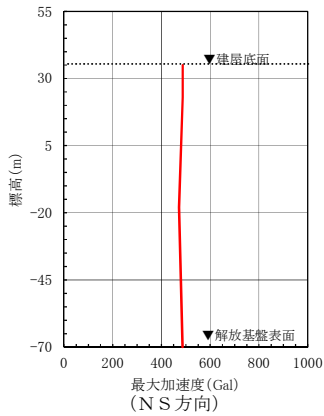
第 4 図(26) 建屋底面位置における地震動 (S s - B 5, ウラン・プルトニウム混合酸化物貯蔵建屋: 東側地盤)
