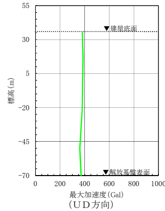
第4図(6) 建屋底面位置における地震動 (S s - B 5, 第1ガラス固化体貯蔵建屋: 西側地盤)
