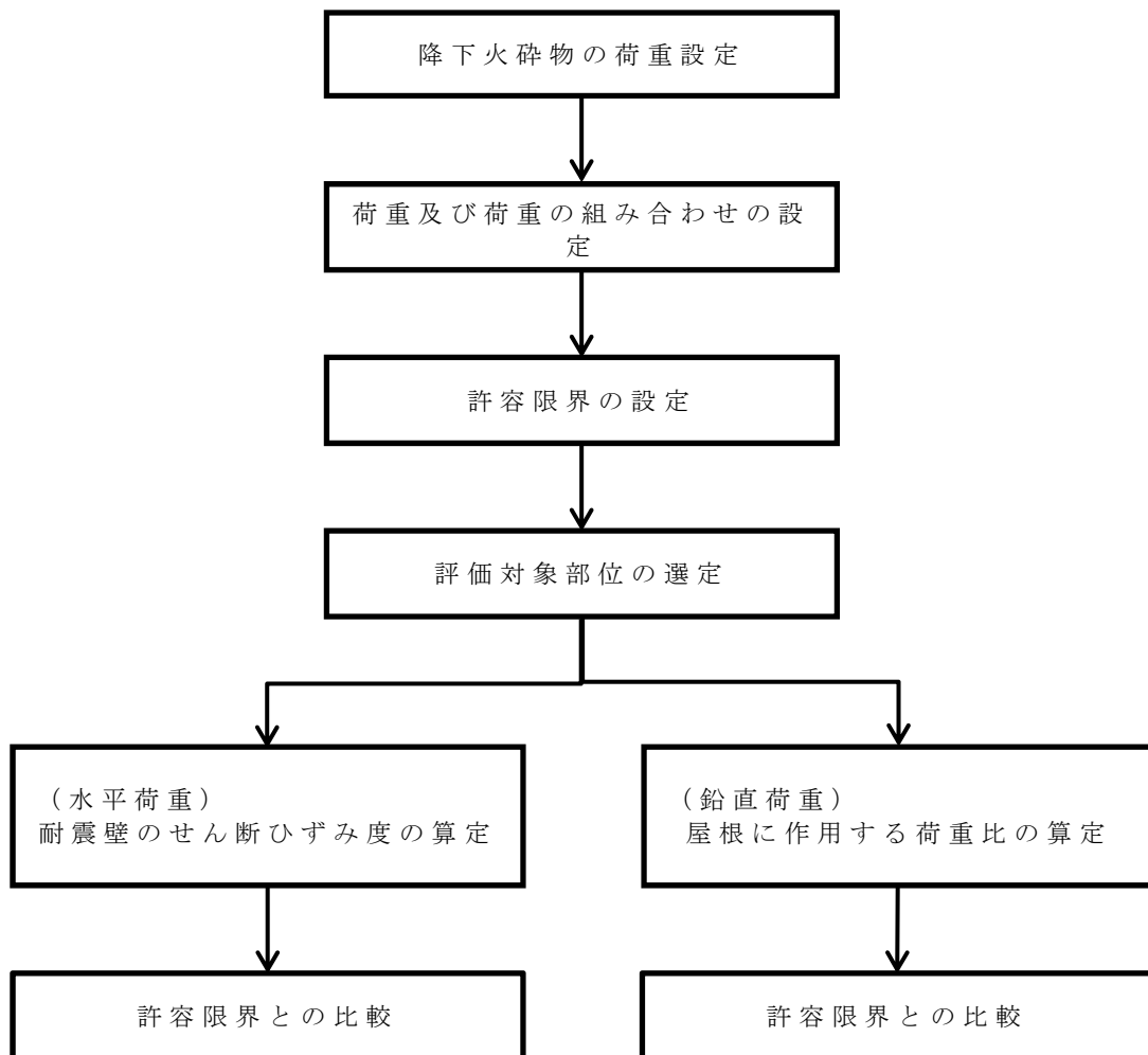
第2.3図 建屋の設計荷重に対する強度評価のフロー図
