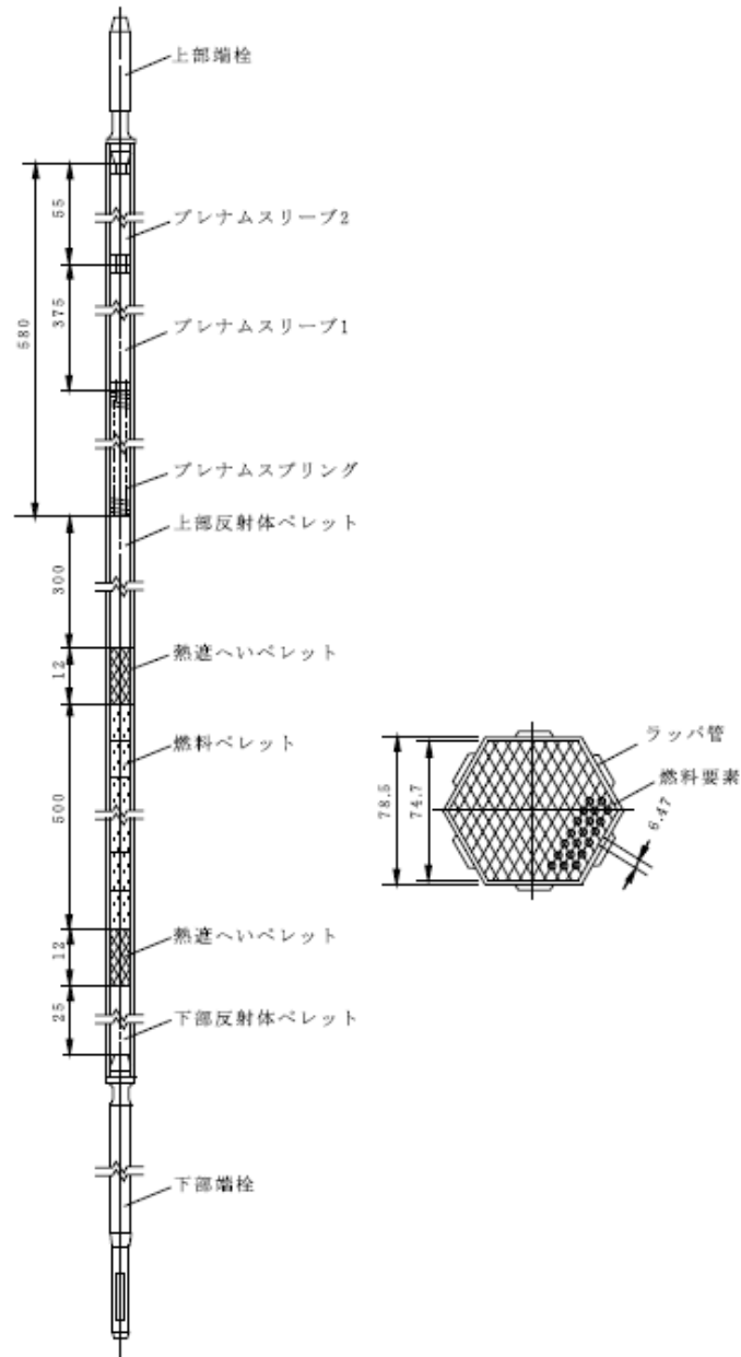
第 2.1.1 図 炉心燃料要素
