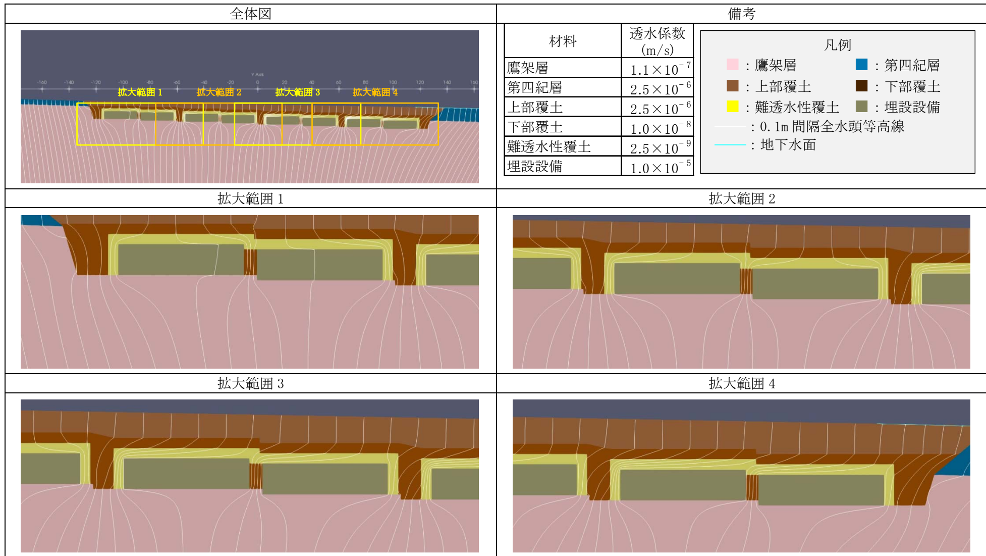
第3図 2次元地下水浸透流解析結果【1号廃棄物埋設地】(基本設定 1,000年後) (1/9) <0.1m 間隔全水頭等高線>
