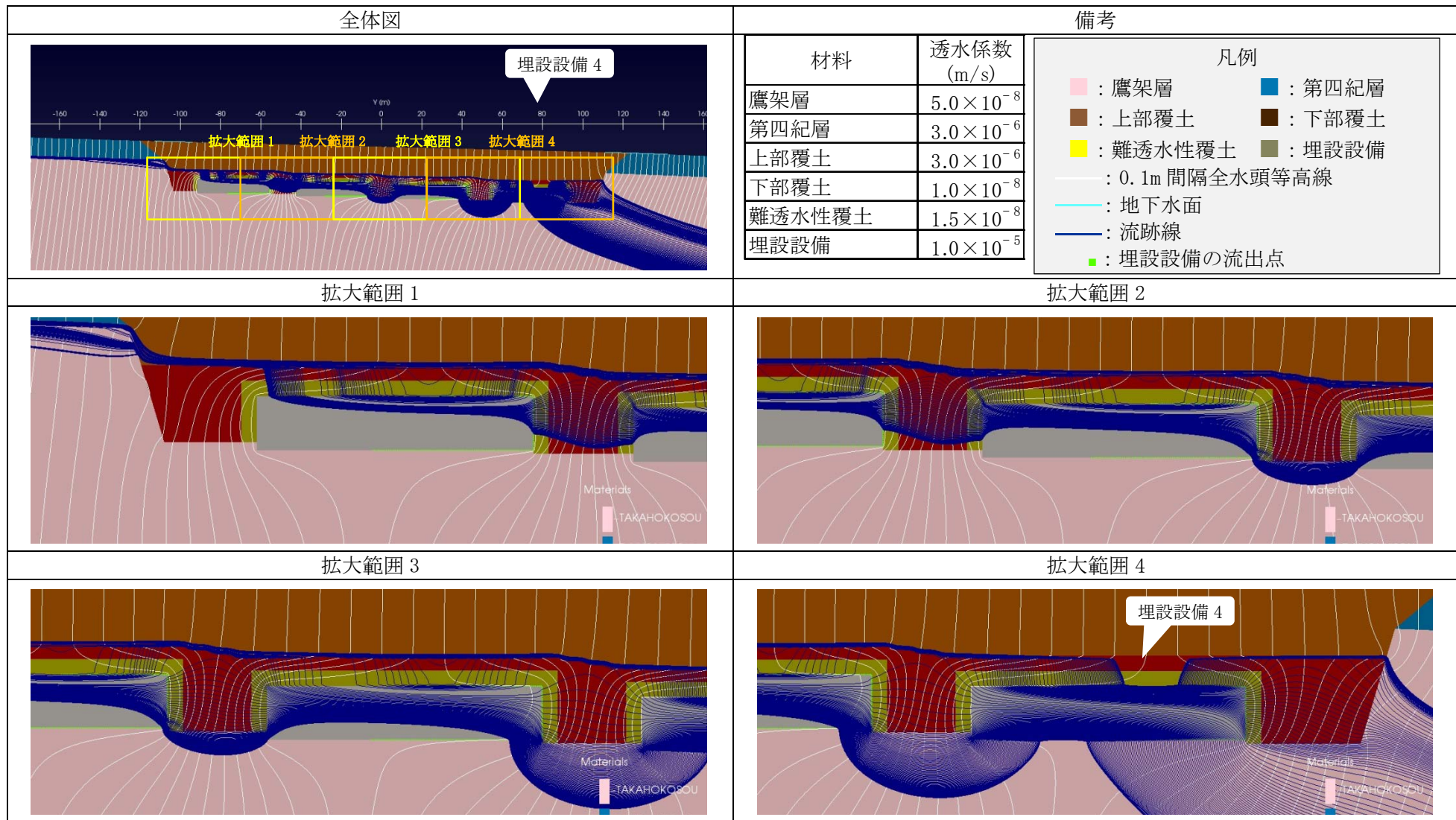
第2図 2次元地下水浸透流解析結果【3号廃棄物埋設地】(変動設定 1,000年後) (5/5) <埋設設備4の流出点を通る流跡線>
