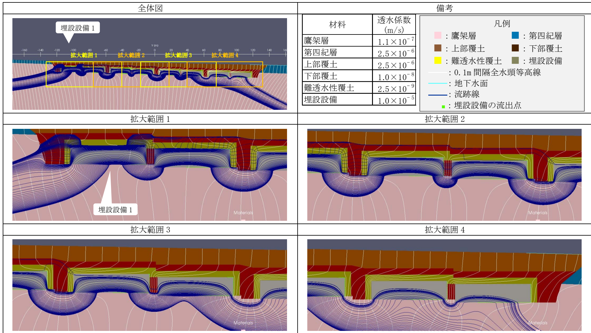
第3図 2次元地下水浸透流解析結果【1号廃棄物埋設地】(基本設定 1,000年後) (2/9) <埋設設備1の流出点を通る流跡線>
