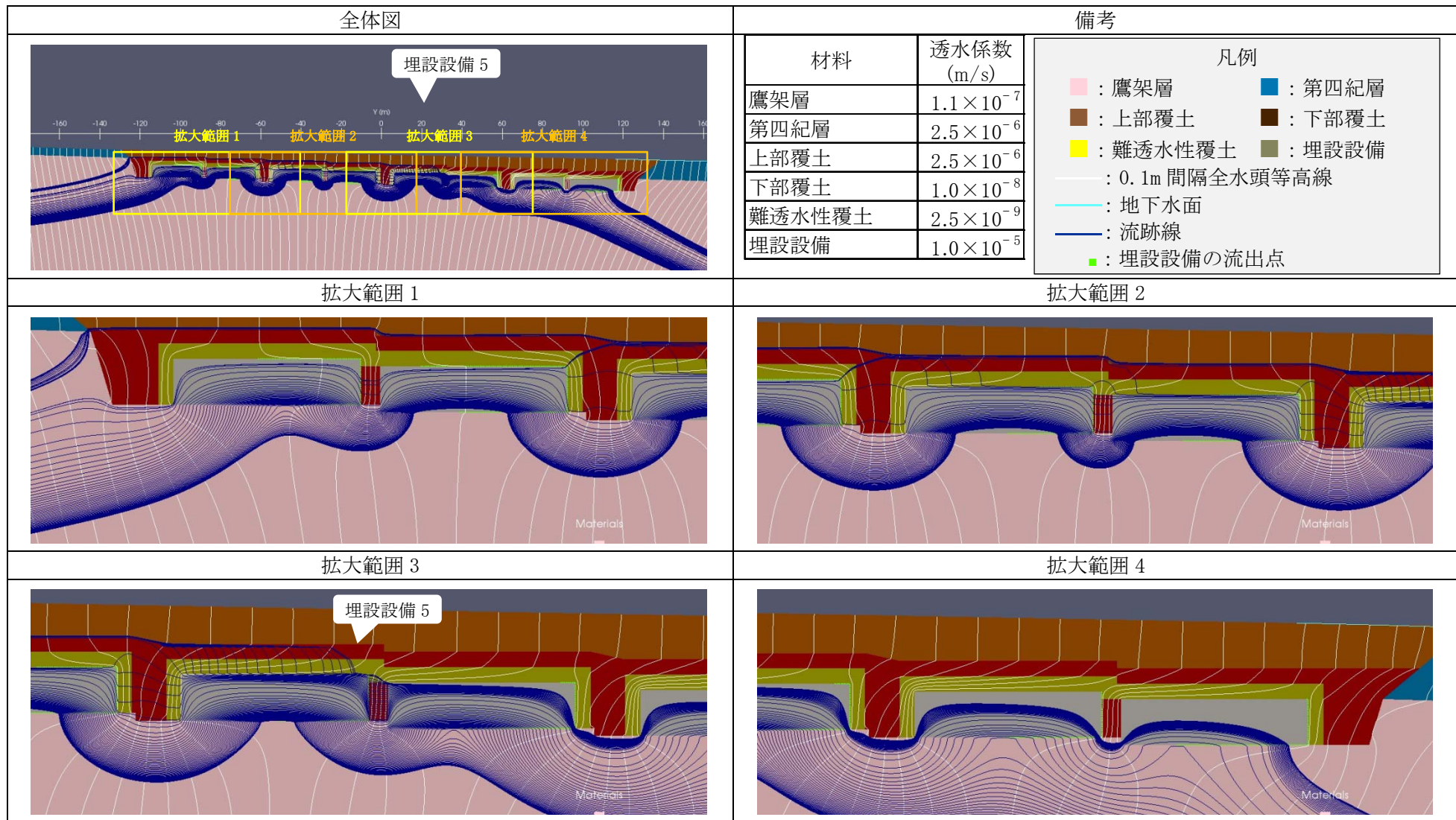
第3図 2次元地下水浸透流解析結果【1号廃棄物埋設地】(基本設定 1,000年後) (6/9) <埋設設備5の流出点を通る流跡線>
