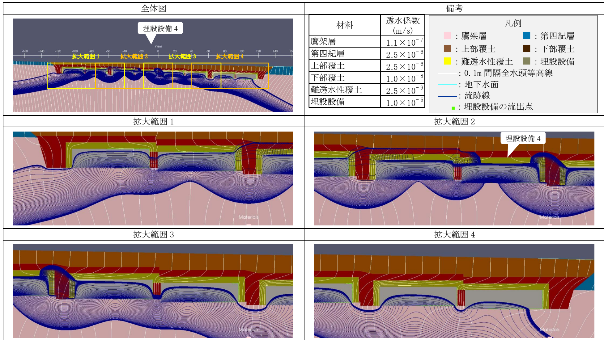
第3図 2次元地下水浸透流解析結果【1号廃棄物埋設地】(基本設定 1,000年後) (5/9) <埋設設備4の流出点を通る流跡線>
