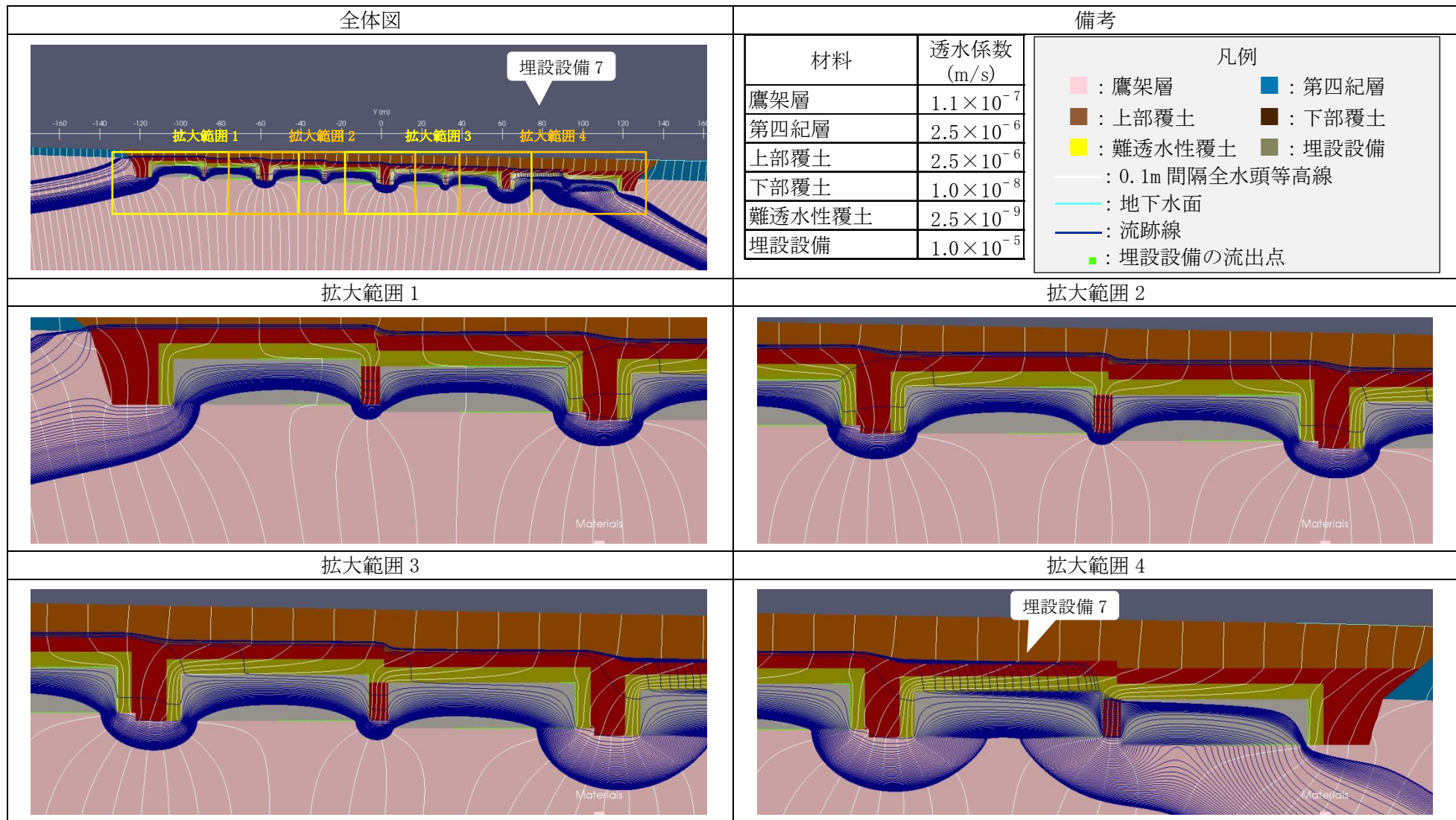
第3図 2次元地下水浸透流解析結果【1号廃棄物埋設地】(基本設定 1,000年後) (8/9) <埋設設備7の流出点を通る流跡線>
