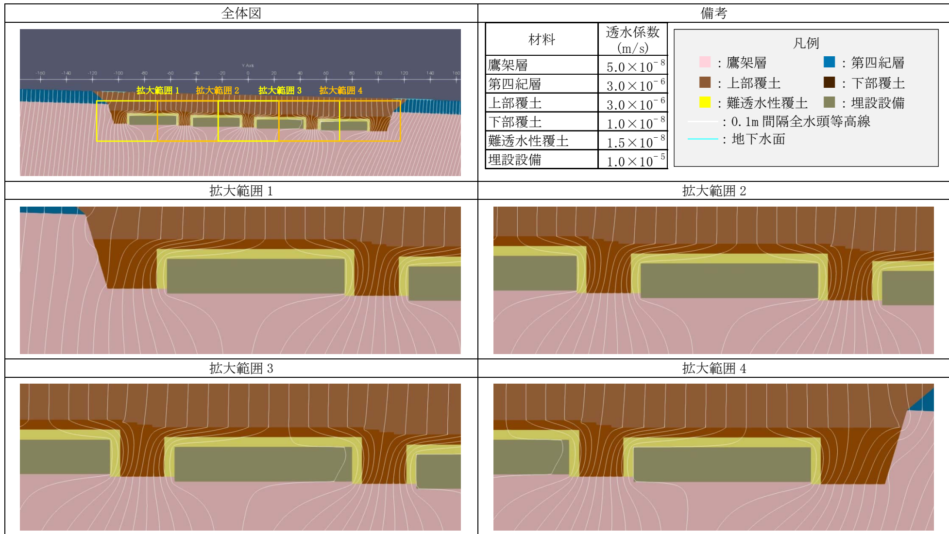
第2図 2次元地下水浸透流解析結果【3号廃棄物埋設地】(変動設定 1,000年後) (1/5) <0.1m 間隔全水頭等高線>
