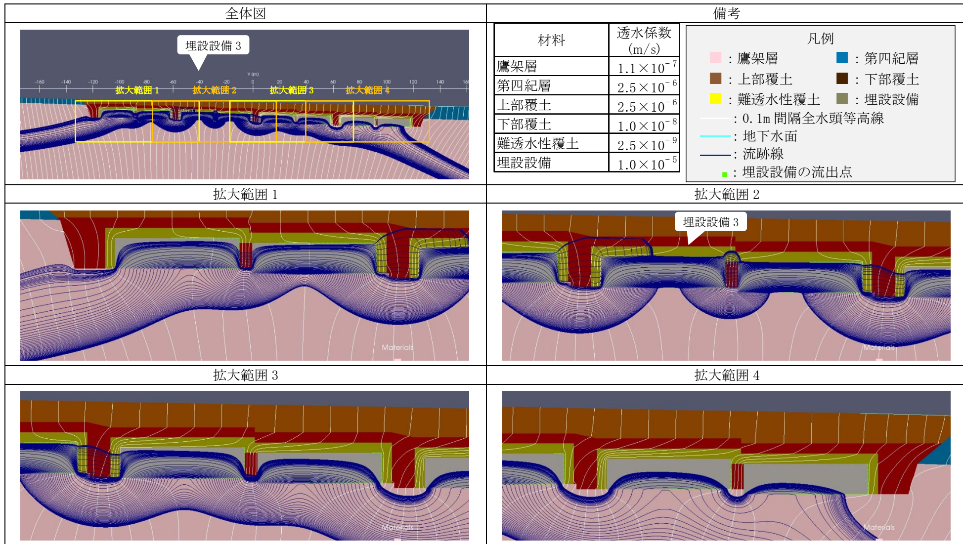
第3図 2次元地下水浸透流解析結果【1号廃棄物埋設地】(基本設定 1,000年後) (4/9) <埋設設備3の流出点を通る流跡線>
