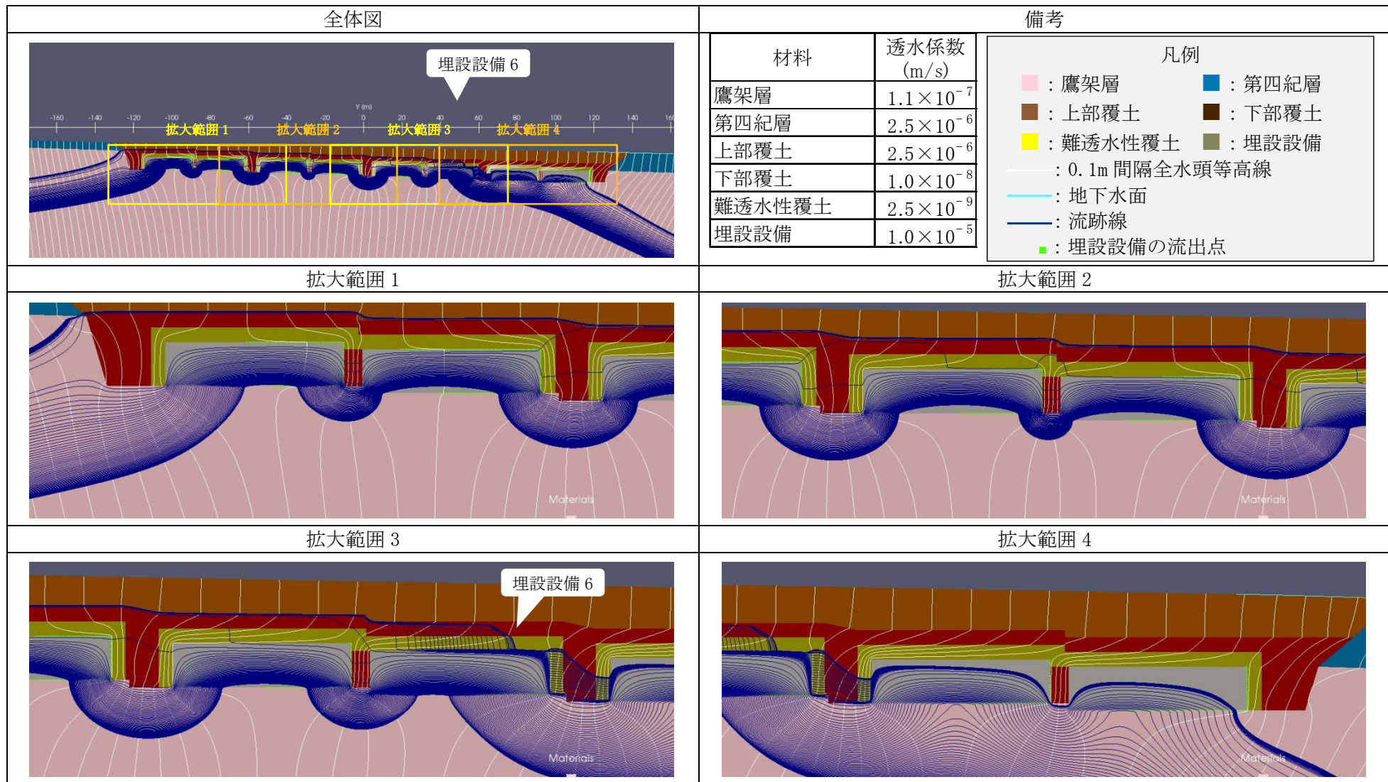
第3図 2次元地下水浸透流解析結果【1号廃棄物埋設地】(基本設定 1,000年後) (7/9) <埋設設備6の流出点を通る流跡線>
