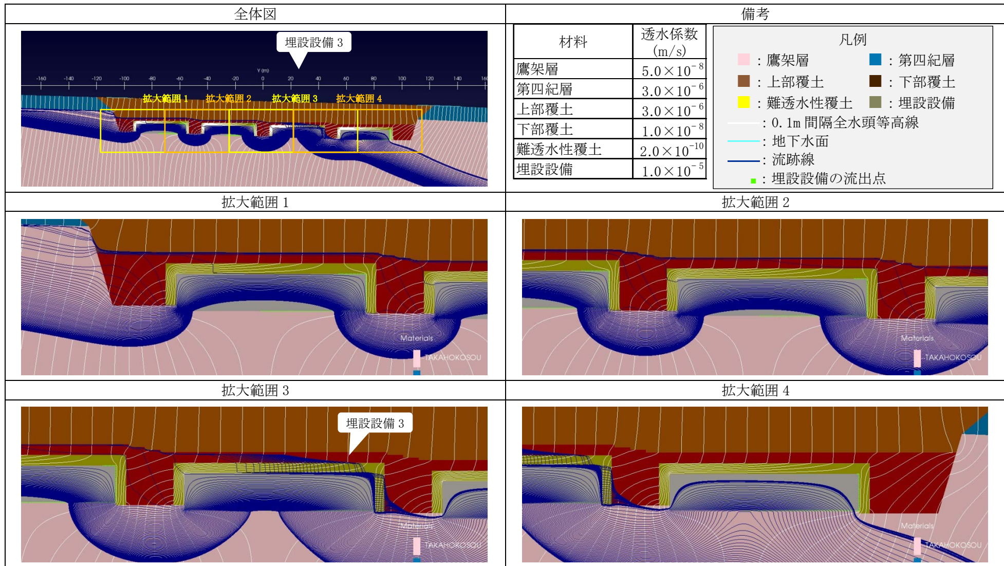
第1図 2次元地下水浸透流解析結果【3号廃棄物埋設地】(基本設定 1,000年後) (4/5) <埋設設備3の流出点を通る流跡線>
