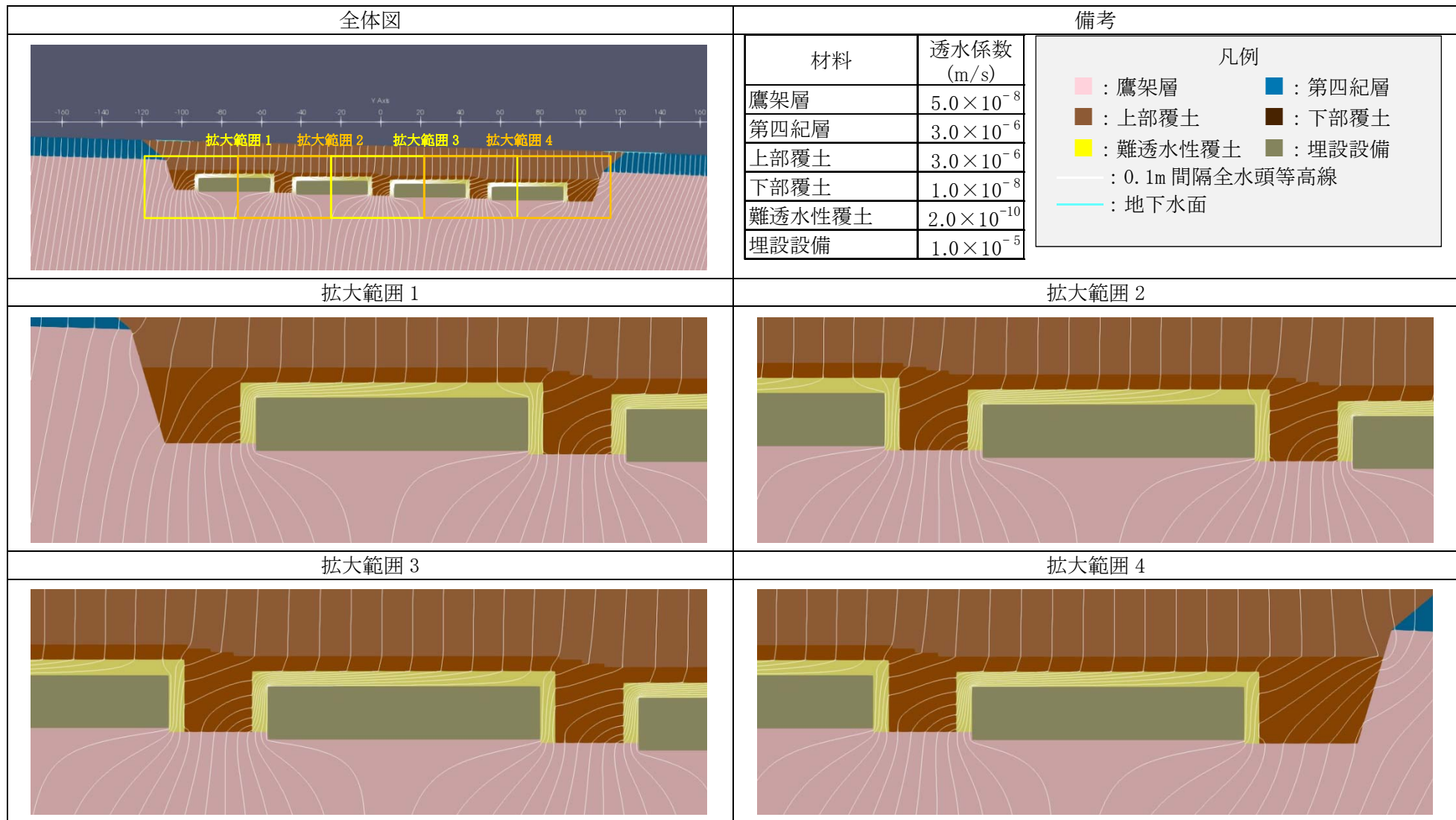
第1図 2次元地下水浸透流解析結果【3号廃棄物埋設地】(基本設定 1,000年後) (1/5) <0.1m 間隔全水頭等高線>
