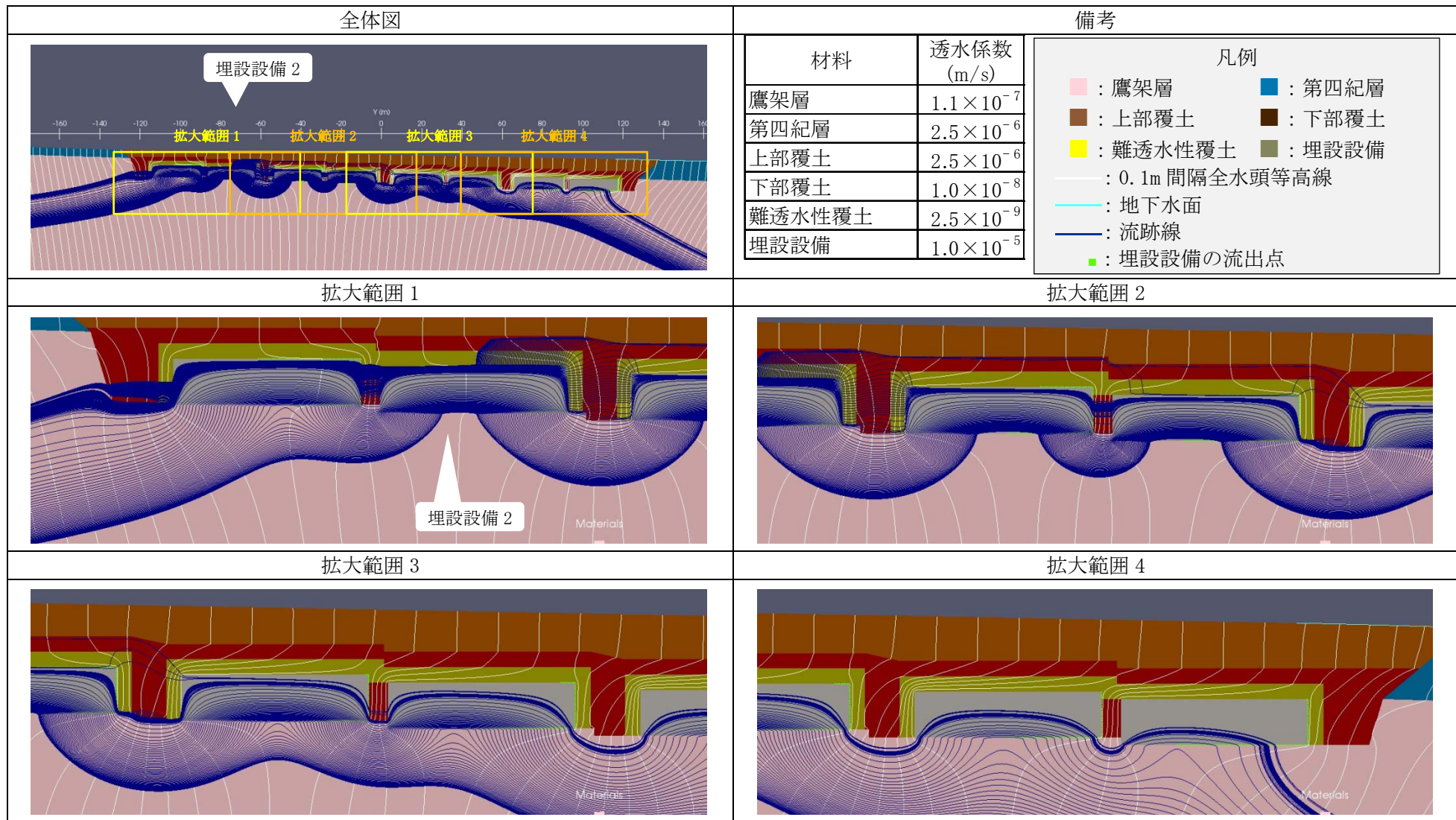
第3図 2次元地下水浸透流解析結果【1号廃棄物埋設地】(基本設定 1,000年後) (3/9) <埋設設備2の流出点を通る流跡線>
