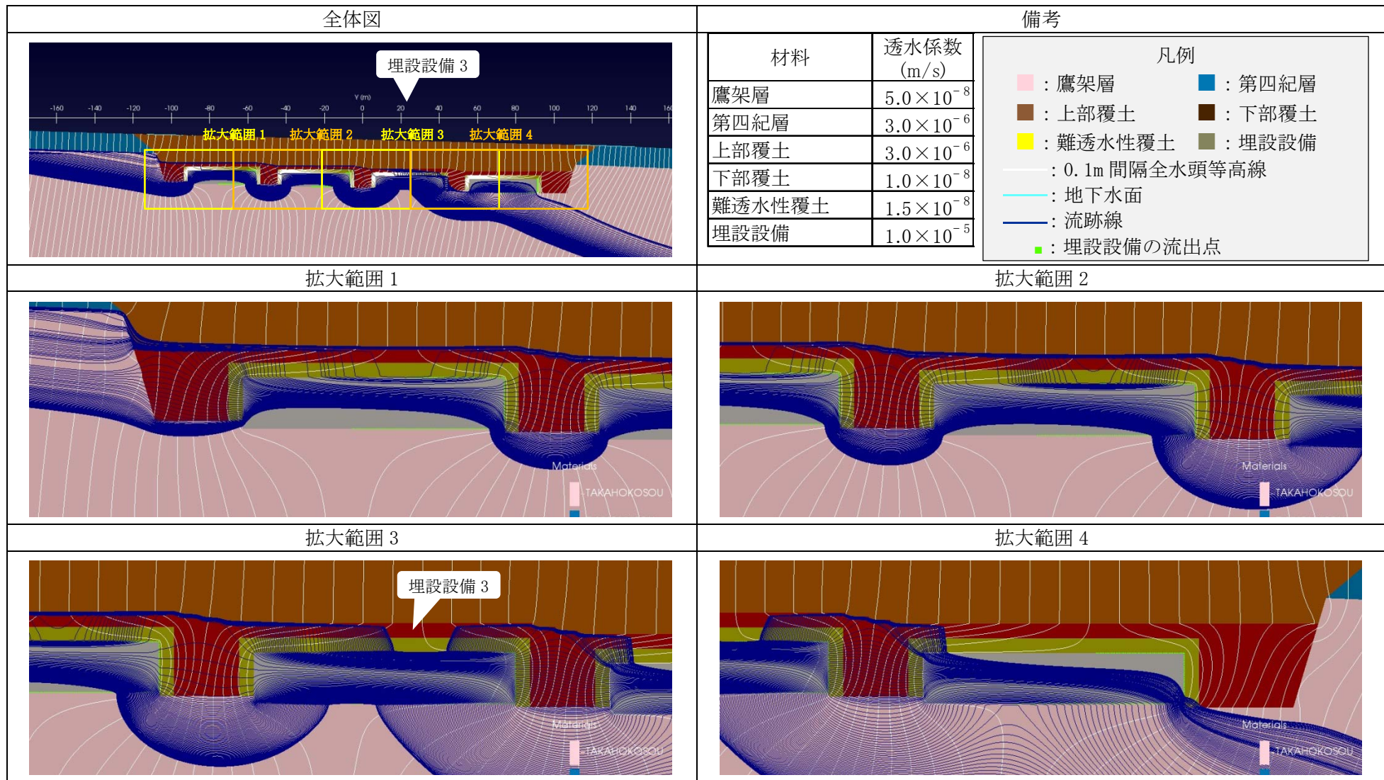
第 2 図 2 次元地下水浸透流解析結果【3号廃棄物埋設地】(変動設定 1,000 年後) (4/5) <埋設設備 3 の流出点を通る流跡線>
