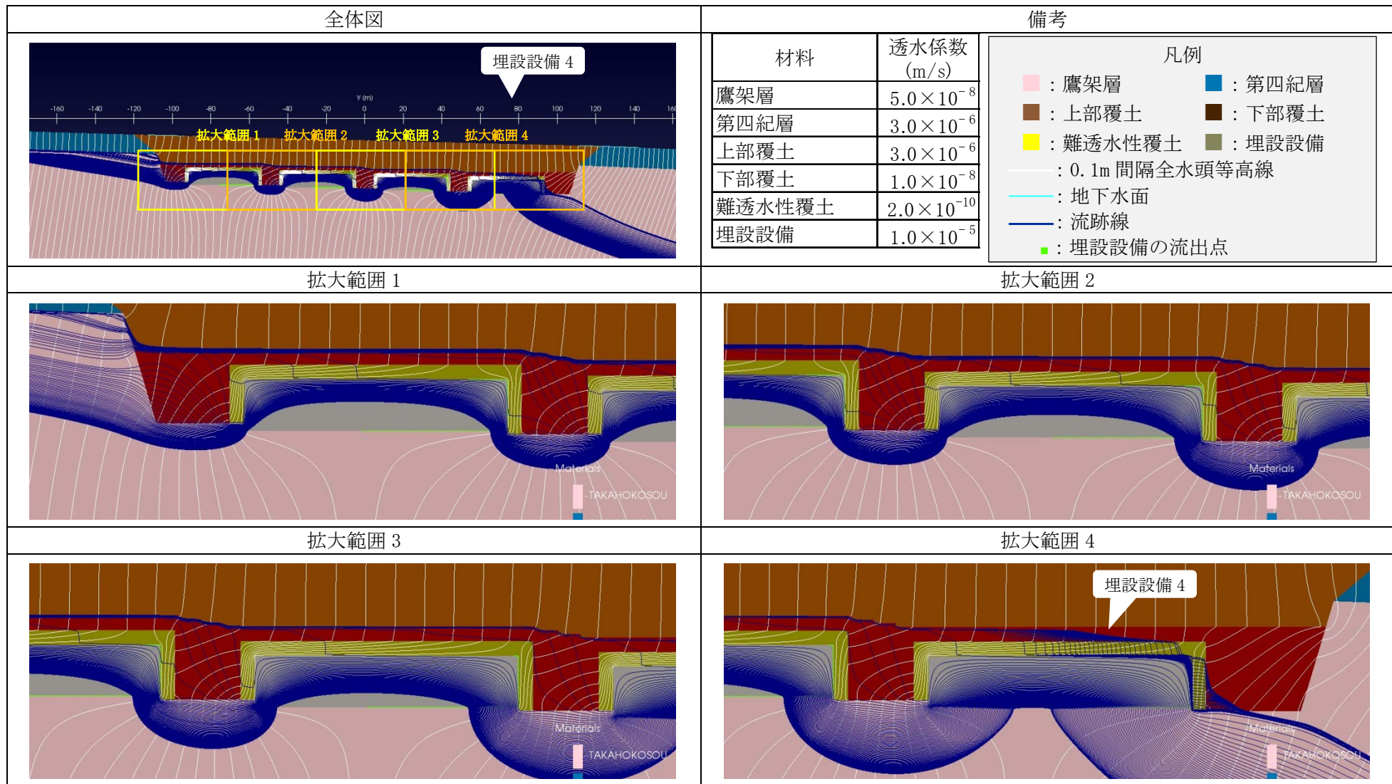
第1図 2次元地下水浸透流解析結果【3号廃棄物埋設地】(基本設定 1,000年後) (5/5) <埋設設備4の流出点を通る流跡線>
