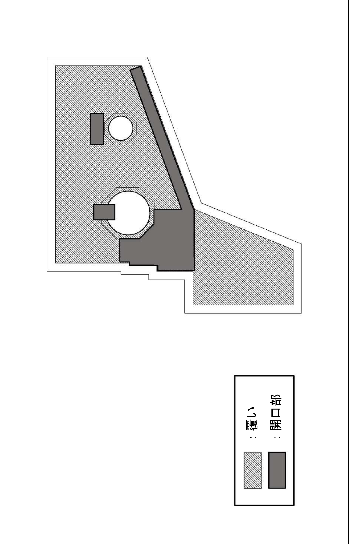
図 5(2/2) 堰 C (1/2 号補給水処理装置) 開口部イメージ
