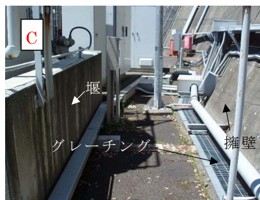
図7 堰周りの状況 (1号ヒドラジン原液タンク)
