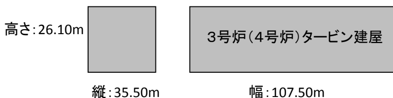
図 16 3号炉（4号炉）のタービン建屋の概要
