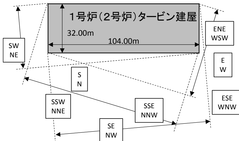
図12 1号炉（2号炉）タービン建屋の見込み方位別の建屋投影面積
