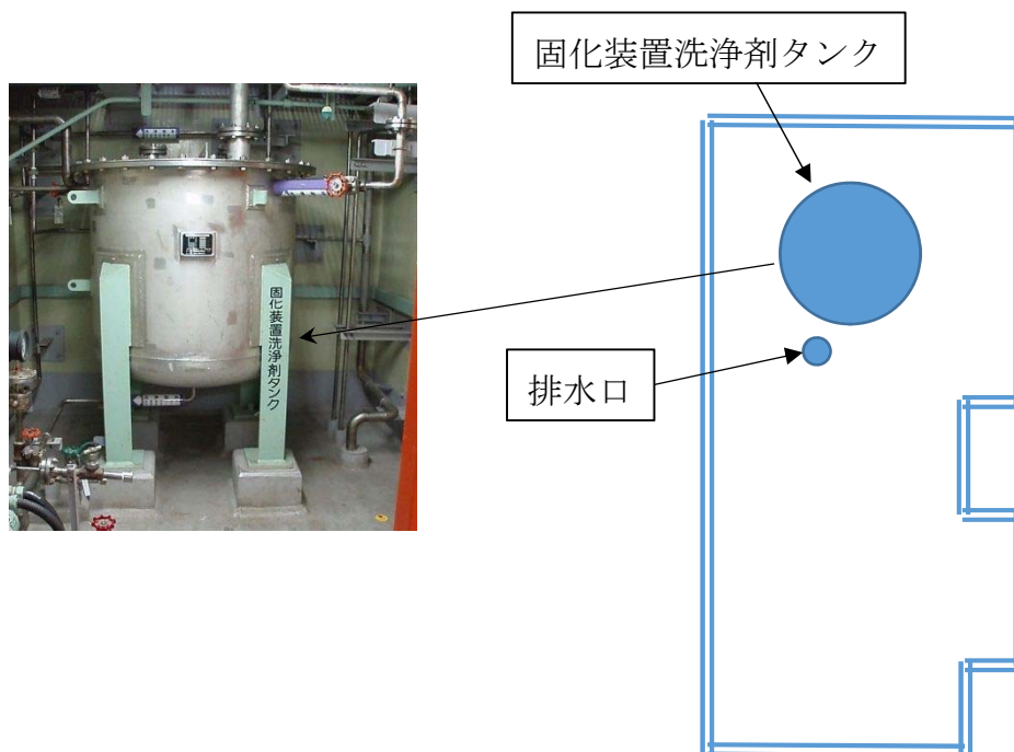
図4 12u 固化装置洗浄剤タンク
