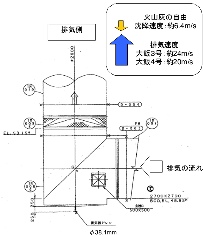
図1 排気筒曲がり部の構造（大飯3号機）
